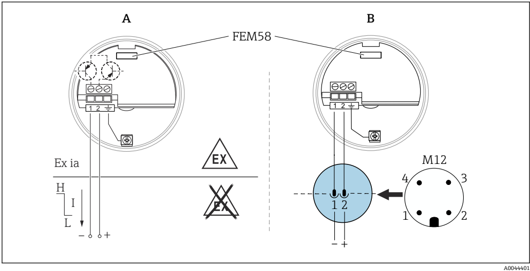
A 符合 IEC 60947-5-6 (NAMUR) 标准的隔离信号转换器; 带电缆入口, 由客户负责接线 (订购选项“080”, 选型代号“2”、“3”、“4”、“7”) B 带 M12 插头, 在工厂接线 (订购选项“080”, 选型代号“1”)
