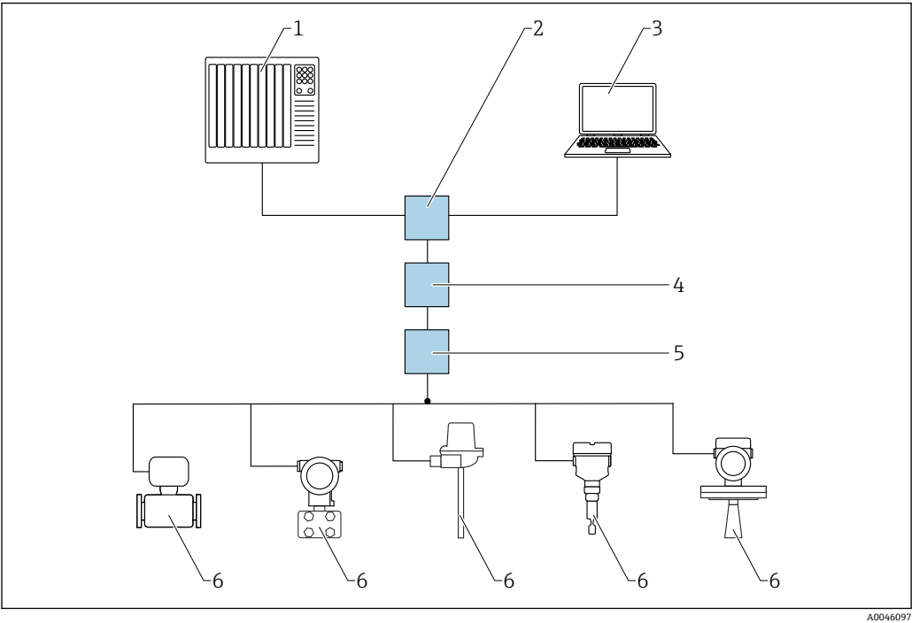
图 24 通过 PROFINET + Ethernet-APL 网络实现远程操作：星形拓扑结构 1 自动化系统，例如 Simatic S7（西门子） 2 以太网交换机 3 计算机，安装有网页浏览器（例如 Microsoft Edge），用于访问设备自带网页服务器；或安装有调试软件（例如 FieldCare、DeviceCare、SIMATIC PDM），带 iDTM PROFINET 通信 4 APL 电源交换机（选配） 5 APL 现场交换机 6 APL 现场设备
