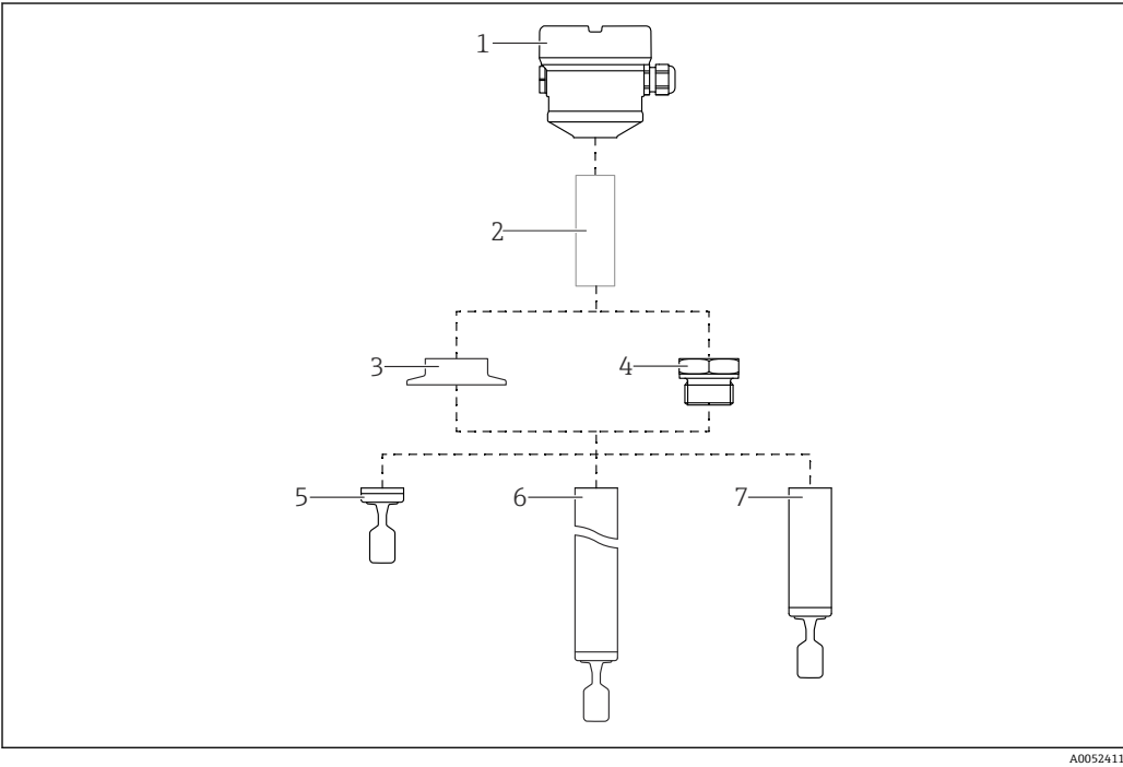
图 2 Liquiphant FTL63 的产品结构 1 外壳，安装有电子插件 FEL60D 和外壳盖 2 选配隔热管，气密馈通（第二道防护） 3 过程连接，例如卡箍/Tri-Clamp 卡箍 4 过程连接，例如螺纹 5 一体式探头，带音叉 6 延长管型探头，带音叉 7 短管型探头，带音叉
