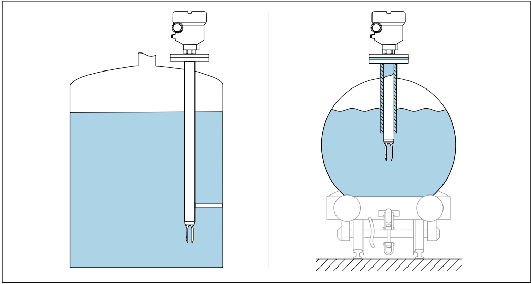
图 10 实例：存在动态负载时，应支撑设备
