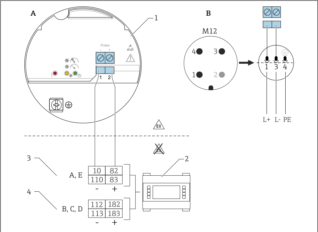
图 18 电子插件 FEL60D 和密度计算仪 FML621 的接线图
