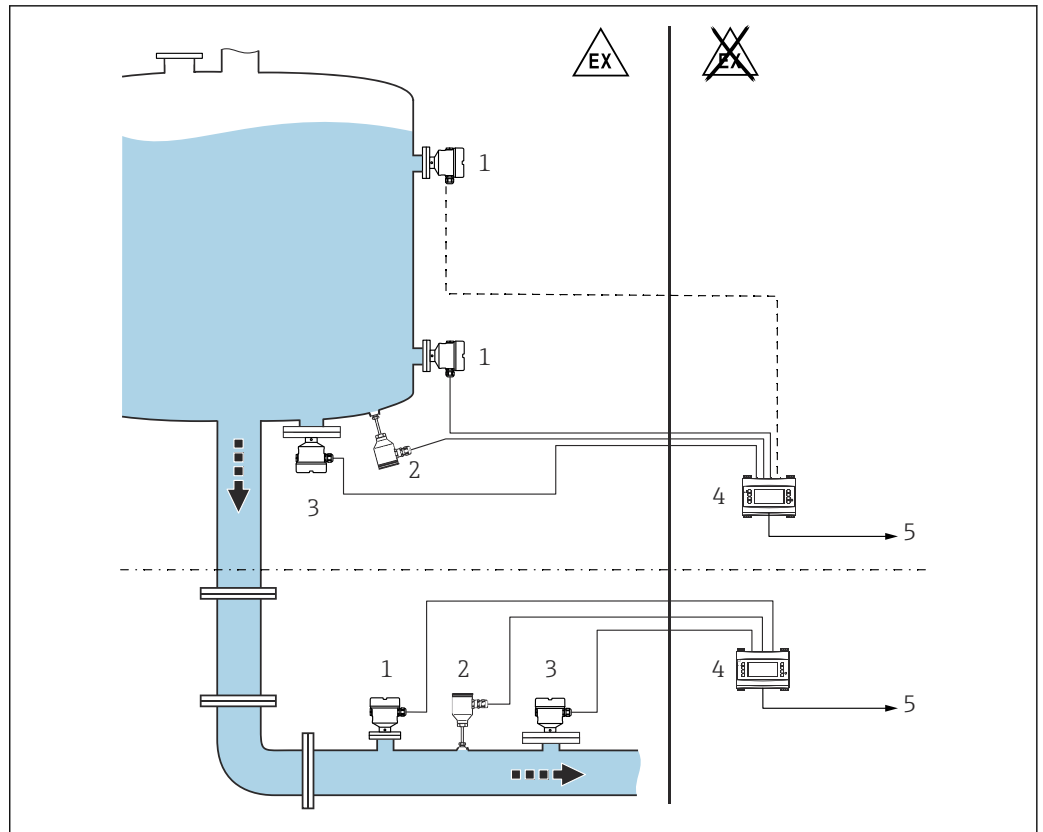
图 19 与密度计算仪 FML621 配套进行密度测量
