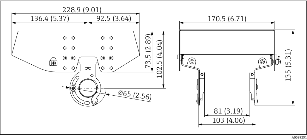
图 22 双腔体铝外壳的防护罩。测量单位 mm (in)
