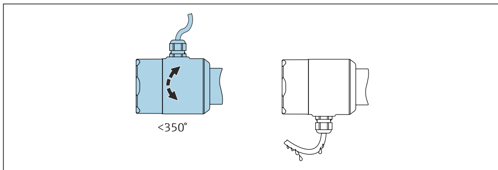
图 15 外壳不带锁紧螺丝，带排水回路
