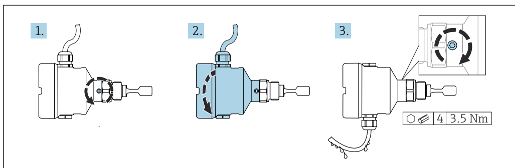
图 16 外壳带外部锁紧螺丝和排水回路
