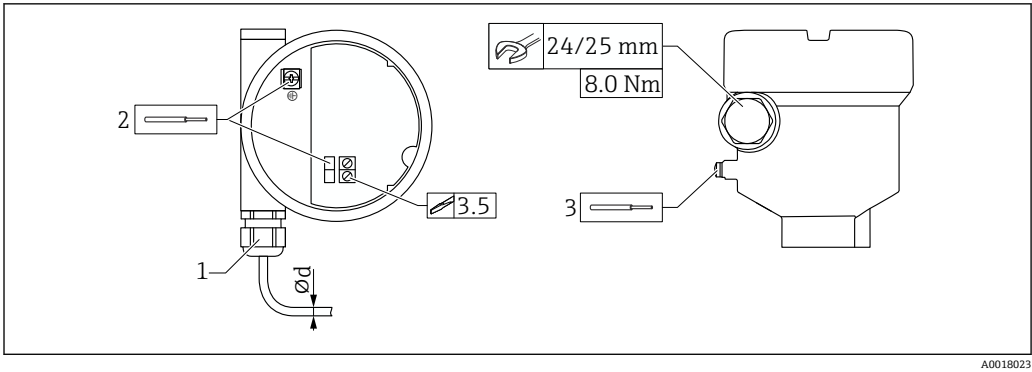
图 20 实例：缆塞（带电缆入口）和电子插件（带接线端子）
