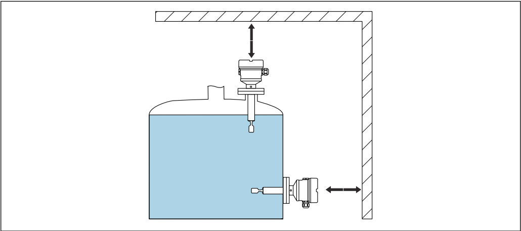
9 预留安装间隙
