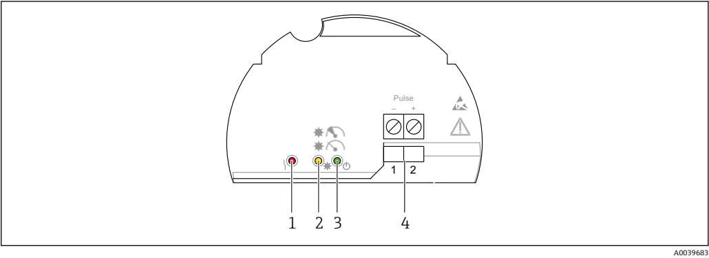
图 21 电子插件 FEL60D
