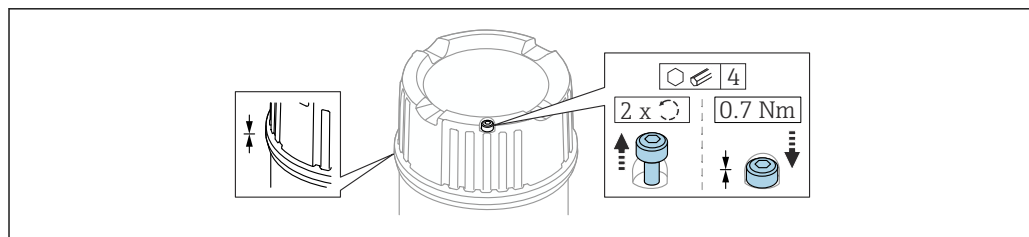
图 17 带锁定螺丝的外壳盖
