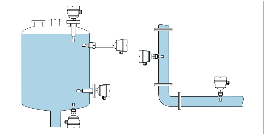
3 安装实例：安装在容器、罐体或管道中
