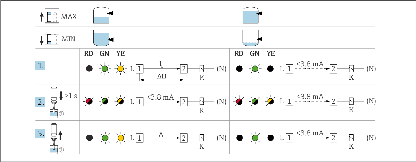
图 37 FEL61 的继电器响应和故障报警信号
