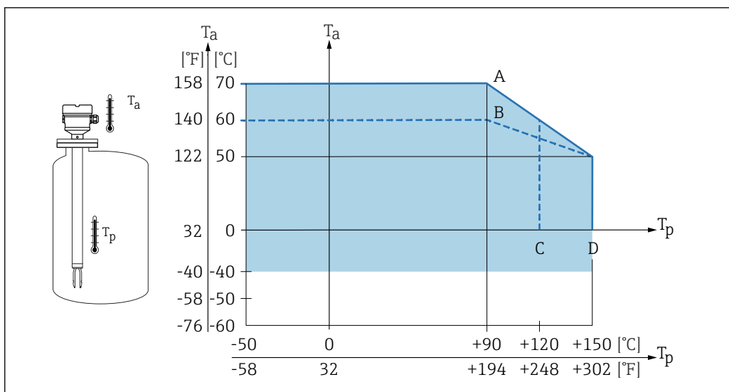
图 50 外壳允许环境温度 T_a 与罐体内部过程温度 T_p 的关系:
