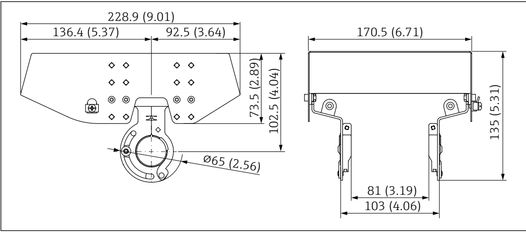
图 46 316L 防护罩 XW112 的外形尺寸示意图。测量单位 mm (in)
