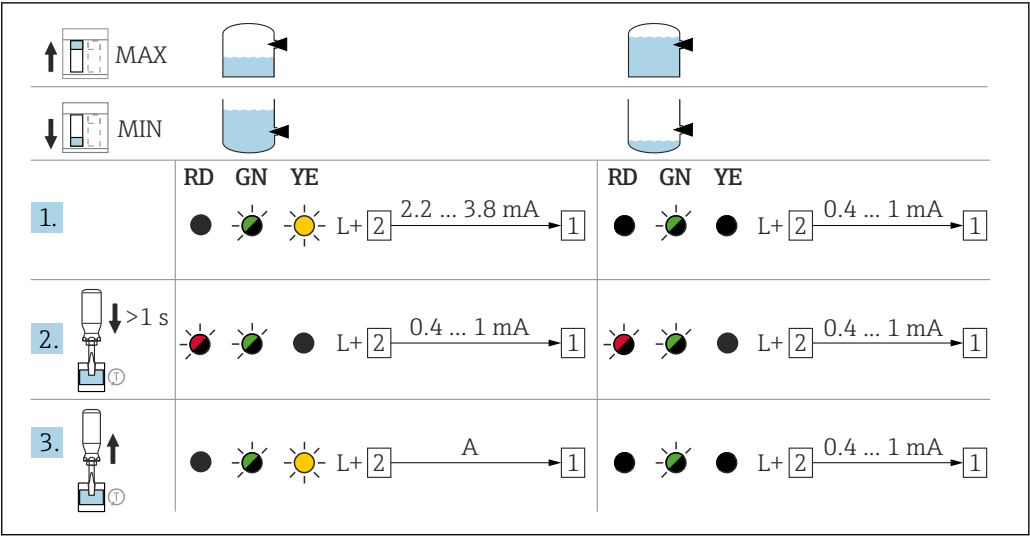
42 NAMUR 电子插件的继电器响应和故障报警信号
