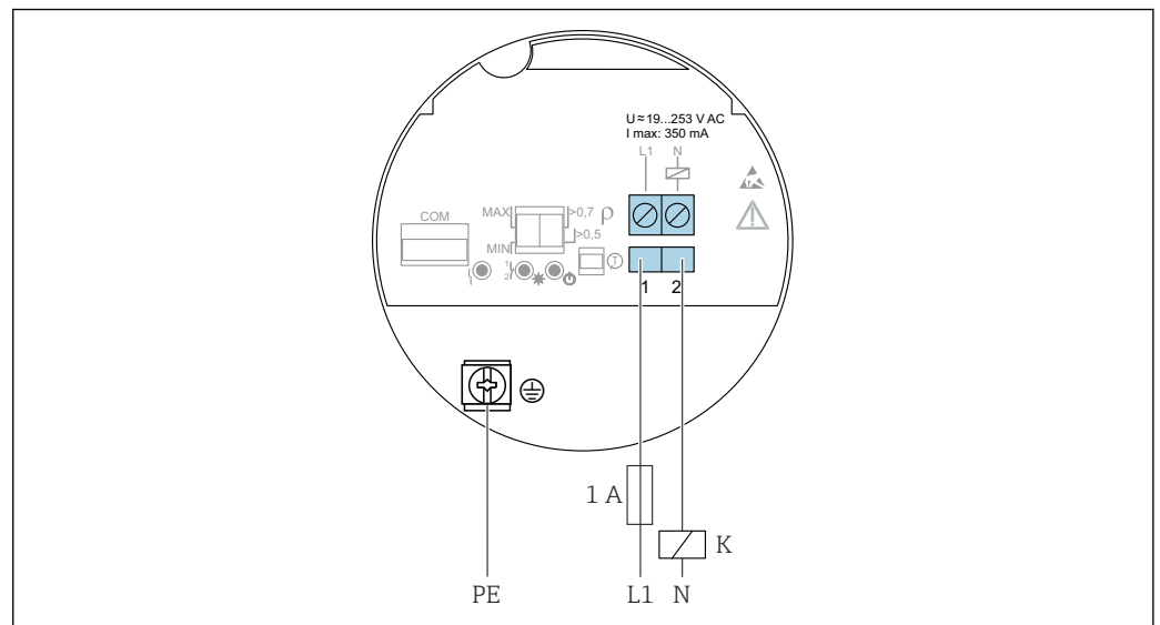
图 17 FEL61 电子插件: 两线制连接, 交流 AC 型
