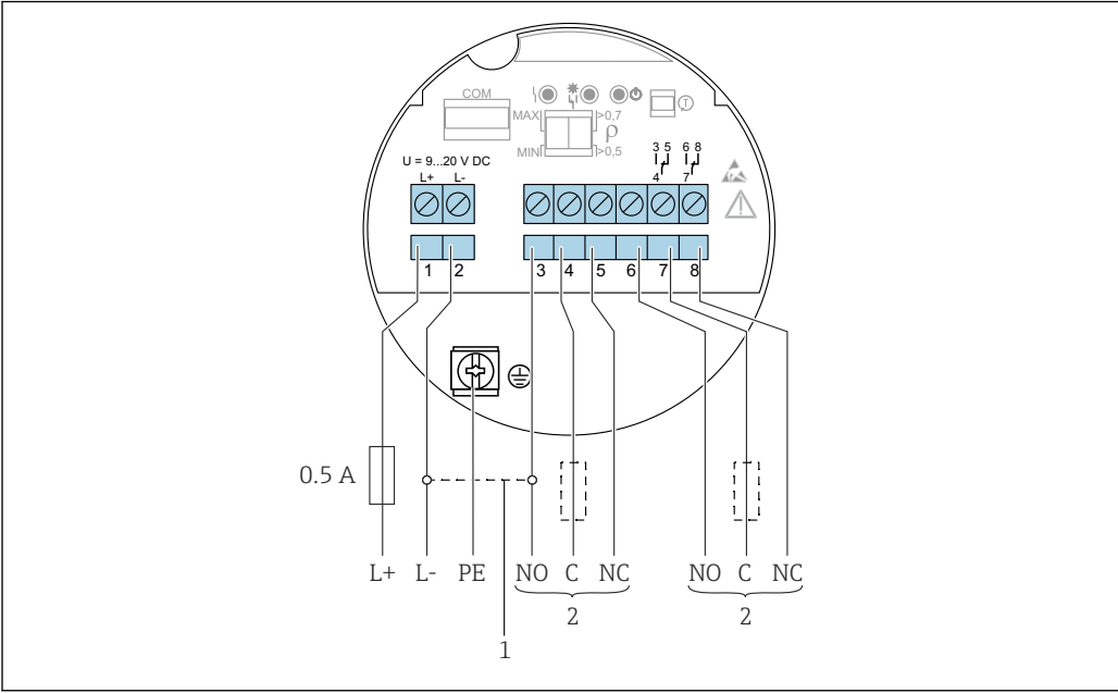
图 24 电子插件 FEL64 DC: 直流连接型, 带继电器输出
