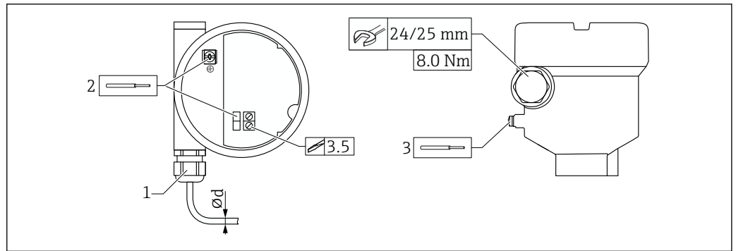
32 实例：接头（带电缆入口）和电子插件（带接线端子）
