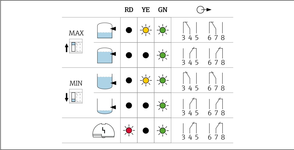
图 25 电子插件 FEL64 DC 的继电器响应和故障信号
