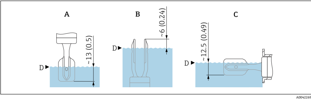
图 5 塑料涂层音叉 (ECTFE、PFA) 的常见开关点, 尺寸参数不含涂层厚度。测量单位 mm (in)
