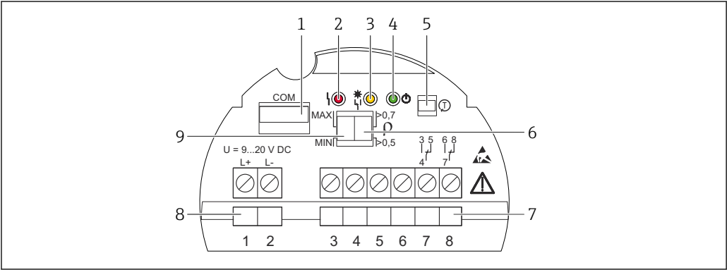
图 33 实例：电子插件 FEL64DC 1 通信接口，用于连接附加模块（LED 指示灯、Bluetooth®蓝牙模块） 2 红色 LED 指示灯：警告或报警 3 黄色 LED 指示灯：音叉开关状态 4 绿色 LED 指示灯：设备工作状态（设备开启） 5 测试按钮，用于执行功能测试 6 DIP 开关，密度设定值为 0.7 或 0.5 7 继电器触点接线端子（3...8） 8 电源接线端子（1...2） 9 DIP 开关，高限（MAX）/低限（MIN）检测设置
