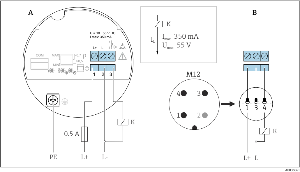
图 20 电子插件 FEL62: 三线制连接, 直流 DC-PNP 型
