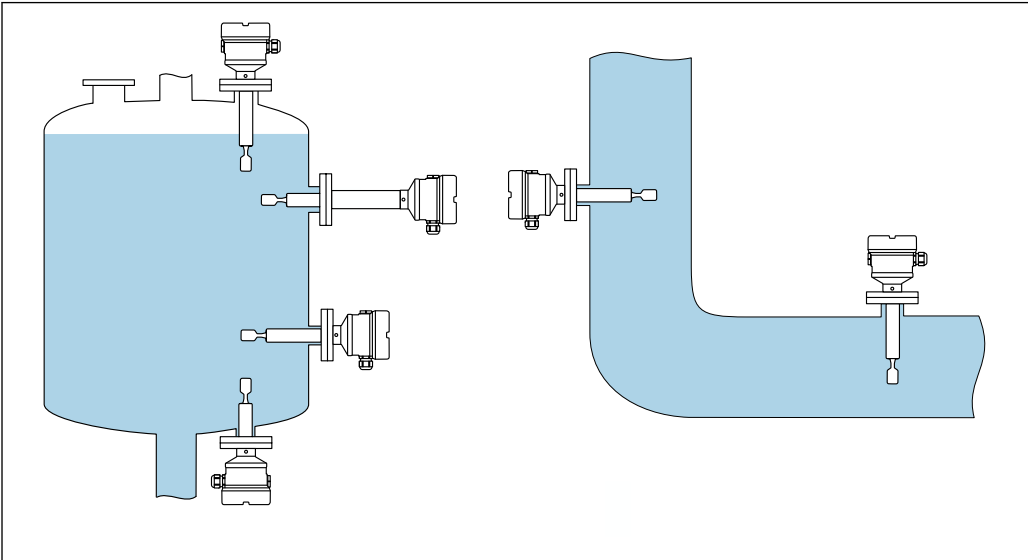
图 4 安装实例：安装在容器、罐体或管道中
