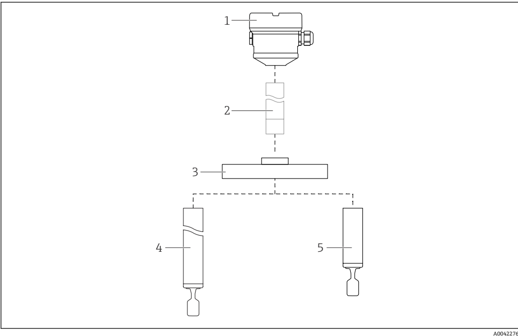
图 2 Liquiphant FTL62 的产品结构 1 外壳，安装有电子插件 FEL60D 和外壳盖 2 选配隔热管，带气密馈通功能（第二道防护） 3 法兰过程连接 4 延长管型探头，带音叉 5 短管型探头，带音叉
