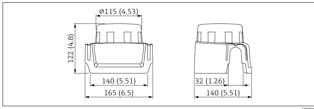
图 24 防护罩，适用单腔体铝外壳。测量单位 mm (in)
