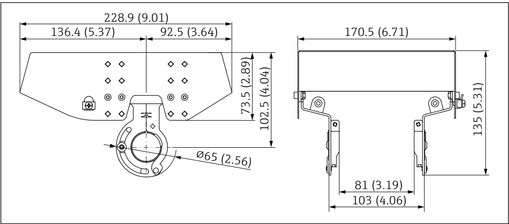
图 23 316L 防护罩 XW112 的外形尺寸示意图。测量单位 mm (in)
