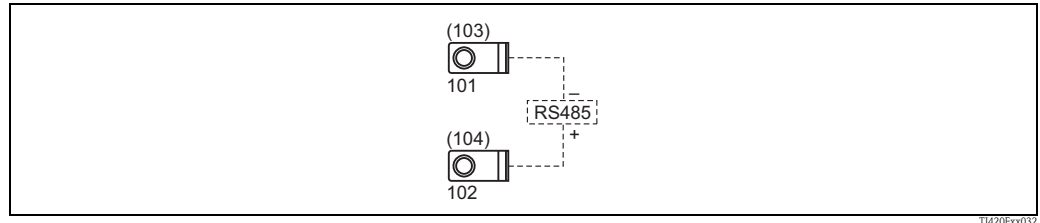
接口连接
