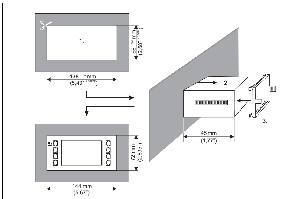
盘式安装
