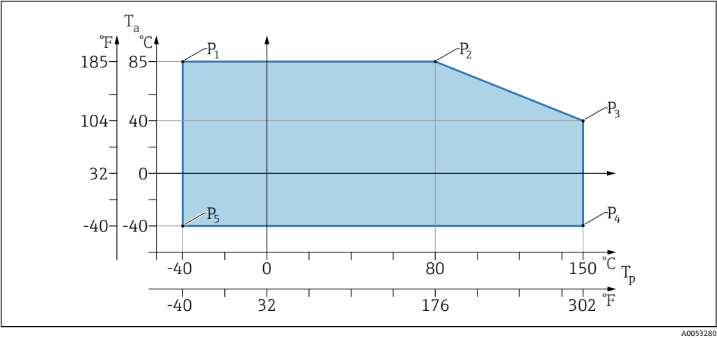
图 22 环境温度 T_a ，取决于过程温度 T_p
