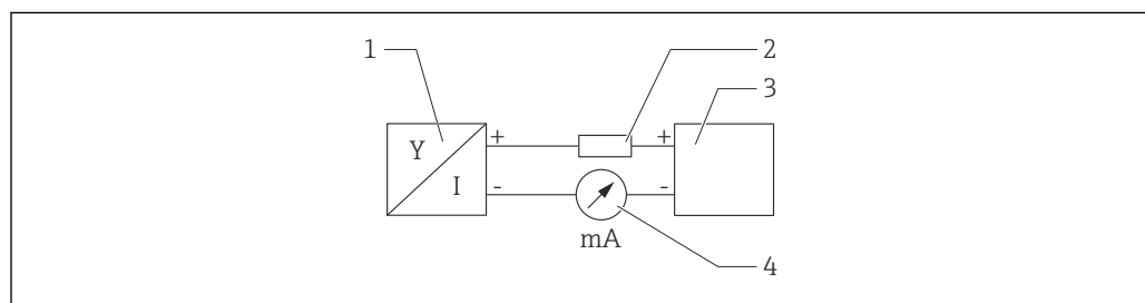
图 16 HART 信号回路接线图
