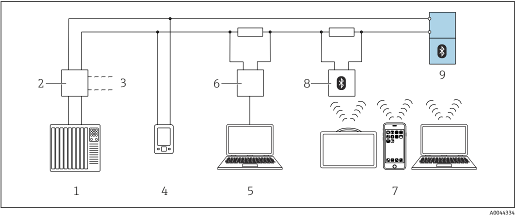
图 19 通过 HART 通信实现远程操作
