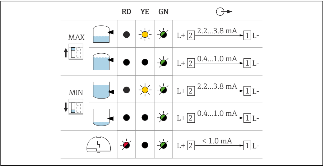
图 22 FEL48 的继电器响应和故障信号
