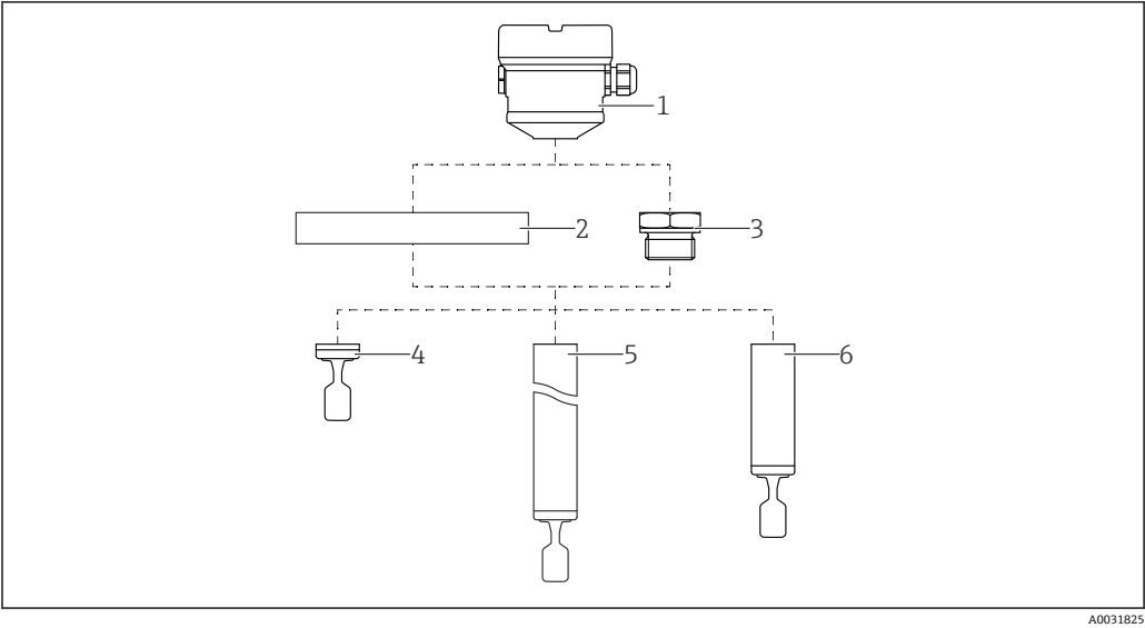
1 产品设计 1 外壳，安装有电子插件和外壳盖 2 过程连接法兰（选配） 3 过程连接（选配） 4 一体型探头，带音叉 5 延长管型探头，带音叉 6 短管型探头，带音叉
