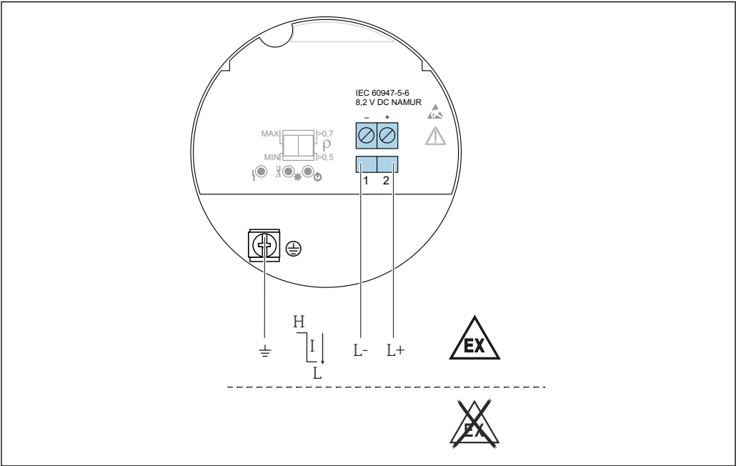
图 21 电子插件 FEL48: 两线制连接, NAMUR 信号 ( \geq 2.2 \text{ mA} / \leq 1.0 \text{ mA} )
