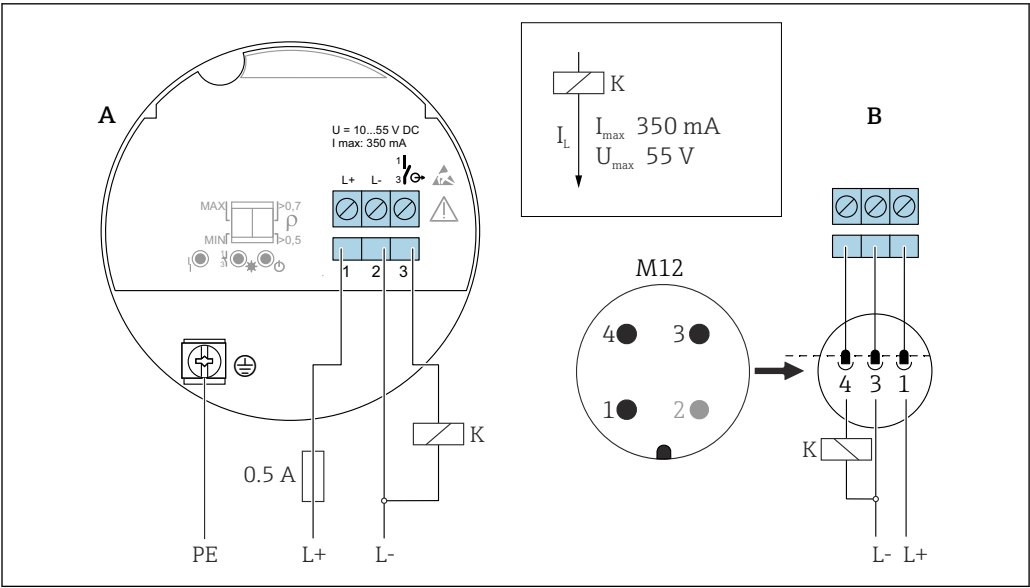
图 17 FEL42 的接线端子分配 A 电子插件的接线端子分配 B M12 连接头的接线端子分配符合 EN61131-2 标准
