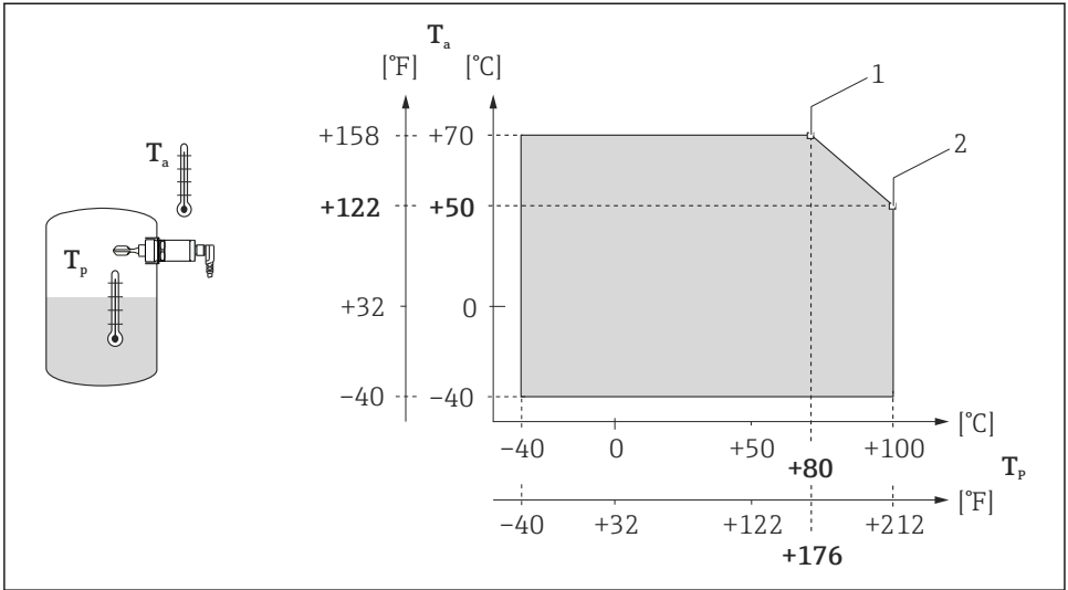
17 温压曲线: 100 °C (212 °F)
