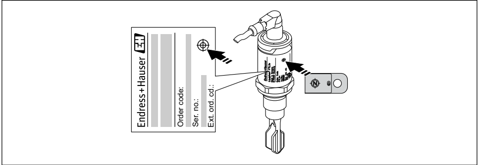
16 外壳上的测试磁铁位置
