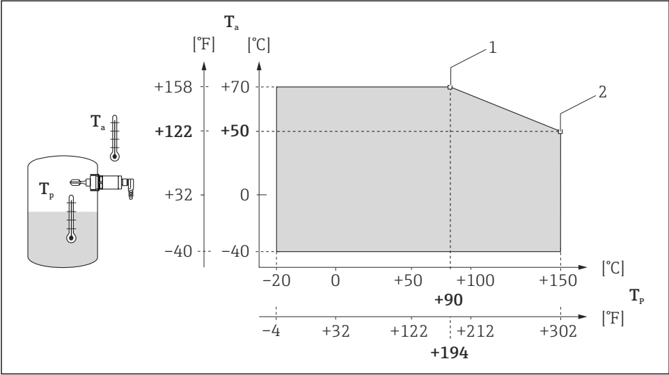
图 18 温压曲线: 150 °C (302 °F)
