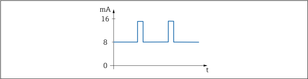
32 PFM 信号，频率范围 17 ... 185 Hz
