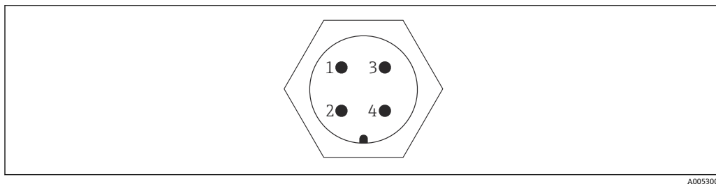
图 7 FEI55、FEI57S、FEI58
