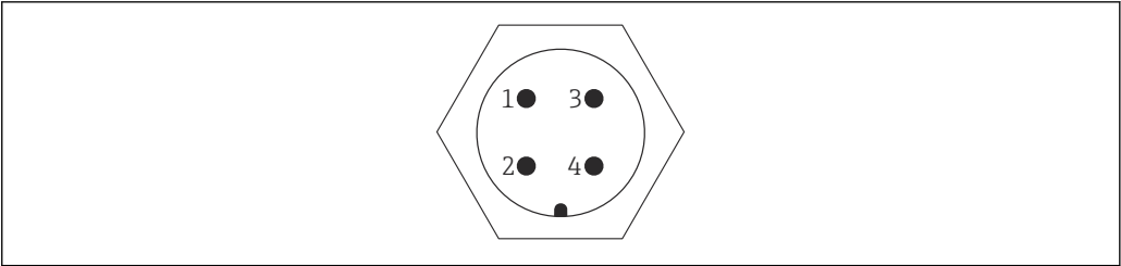
图 6 FEI52、FEI53
