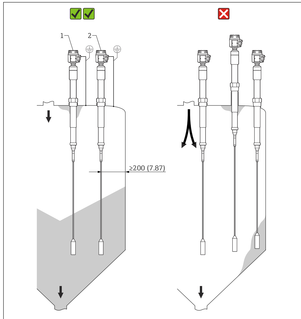
图 17 缆式探头安装实例
