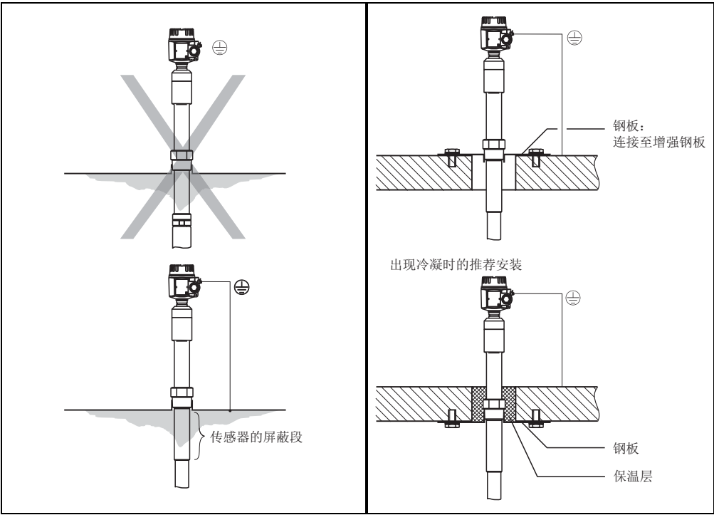
导电性料仓壁
