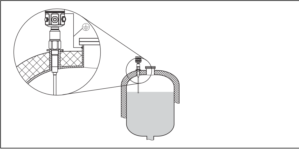
FTI51: 杆式传感器，带接地管和屏蔽段长度 ( 安装短管 )
