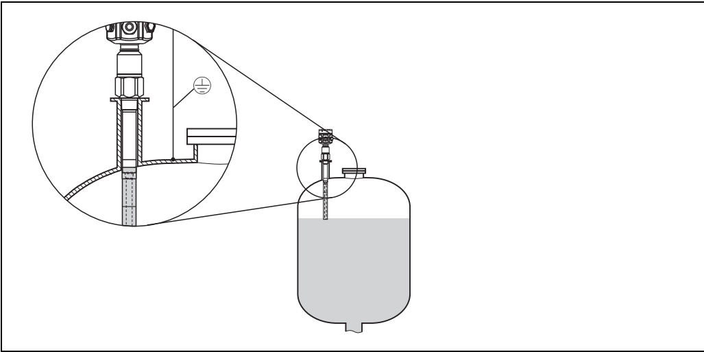
FTI51: 全绝缘传感器，带涂层法兰，用于腐蚀性介质测量
