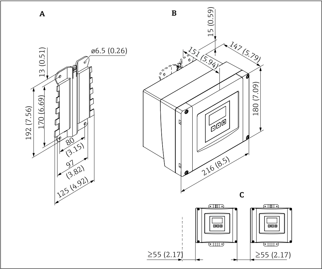
4 采用聚碳酸酯现场型外壳的 Prosonic S 的外形尺寸。测量单位 mm (in)
