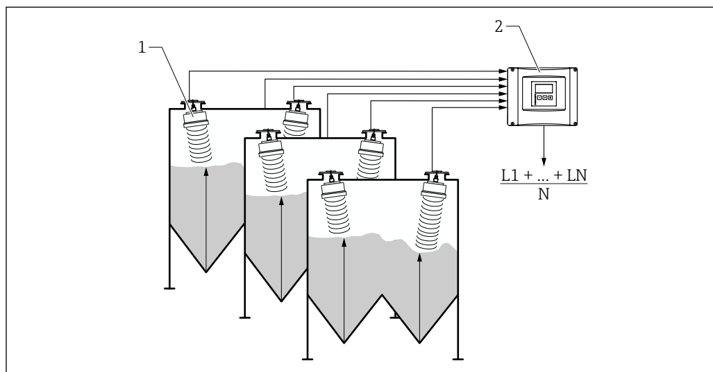
图 3 多通道物位测量（计算平均物位）
