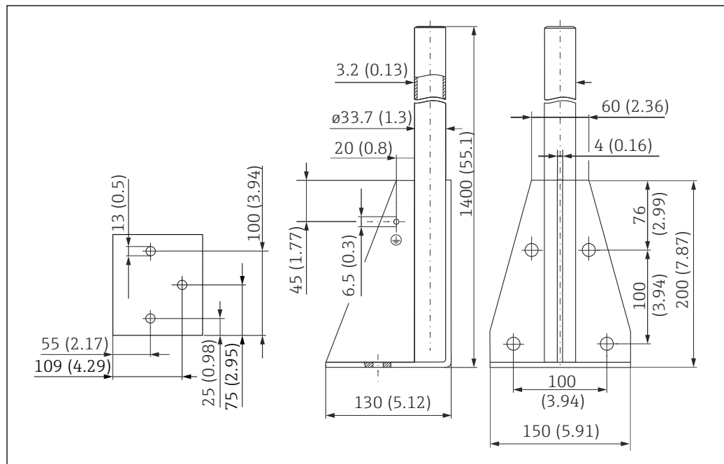
图 15 外形尺寸。测量单位 mm (in)
