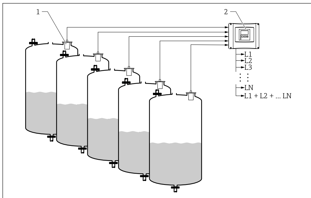
图 2 多通道物位测量（计算累计物位）
