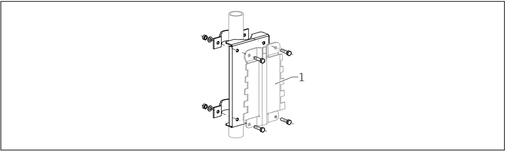
图 13 安装板，适用聚碳酸酯现场型外壳
