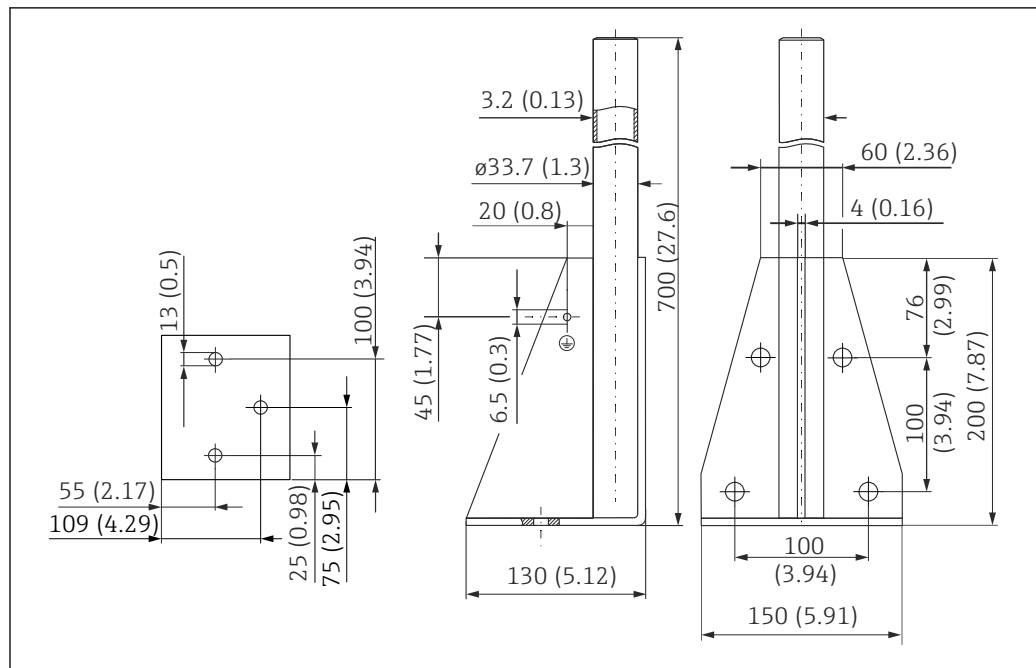
图 14 外形尺寸。测量单位 mm (in)
