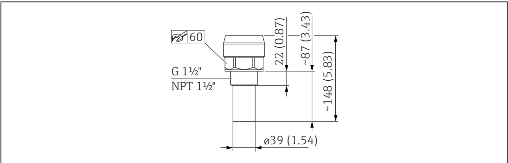
19 FMU40 传感器的外形尺寸。测量单位 mm (in)
