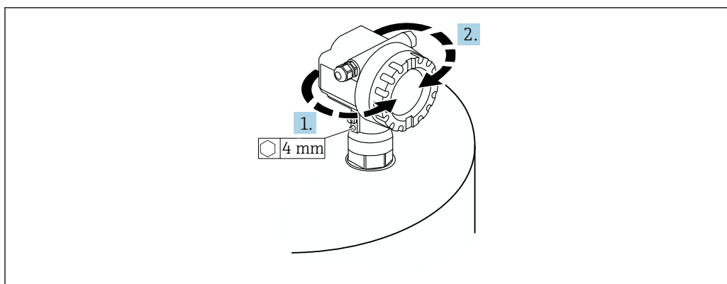
图 14 旋转 F12 或 T12 外壳（实例：F12 外壳）
