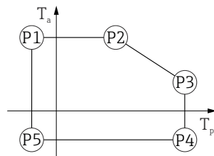
图 44 316L 外壳，卫生型；过程温度范围：-40 ... +80 °C (-40 ... +176 °F)
