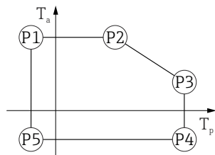
图 37 铝外壳, 带涂层; 过程温度: -40 ... +280 °C (-40 ... +536 °F)
