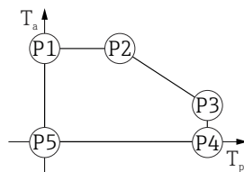
图 29 塑料外壳; 过程温度范围: 0 \dots +200 \text{ }^{\circ}\text{C} ( +32 \dots +392 \text{ }^{\circ}\text{F} ), 适用 CSA C/US 认证型仪表
