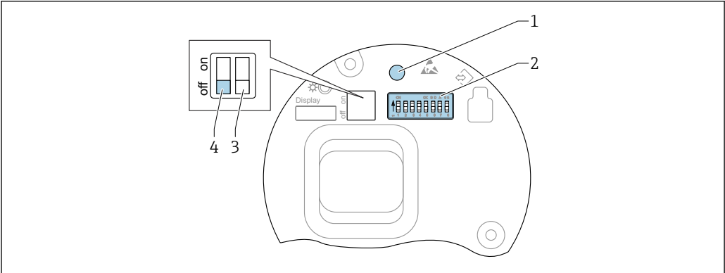
图 11 PROFIBUS PA 电子插件上的操作按键和 DIP 开关 1 操作按键，用于密码重置（Bluetooth 蓝牙登陆和切换至维护用户角色） 2 DIP 开关，用于地址设置 3 DIP 开关，无功能 4 DIP 开关，用于锁定和解锁设备
