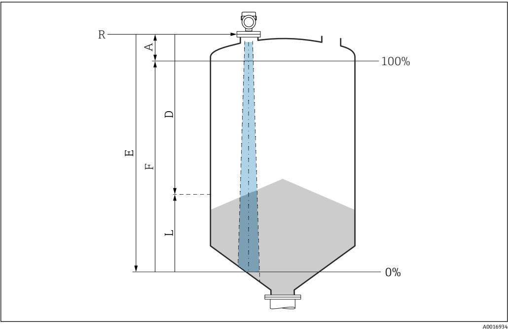
图 16 固体散料料位测量的设置参数
