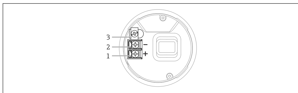
图 7 接线腔内的接线端子和接地端，单腔室外壳
