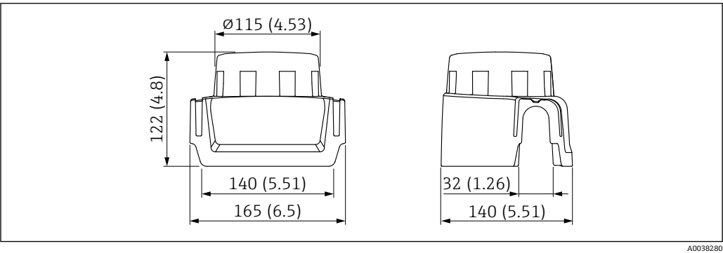
图 23 塑料防护罩 XW111 的外形尺寸示意图。测量单位 mm (in)
