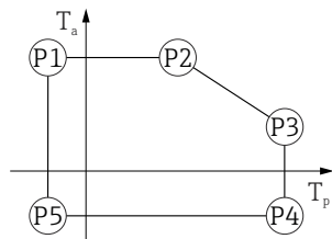
图 38 铝外壳, 带涂层; 过程温度: -40 ... +450 °C (-40 ... +842 °F)
