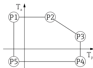
图 45 316L 外壳，卫生型；过程温度范围：-40 ... +150 °C (-40 ... +302 °F)
