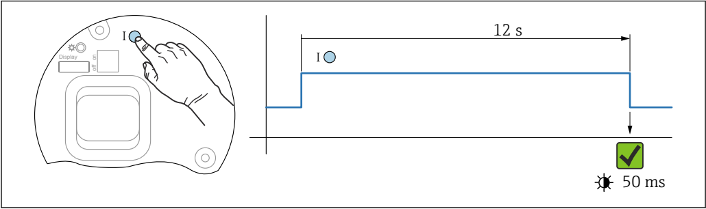
图 21 时序图 - 恢复出厂设置
