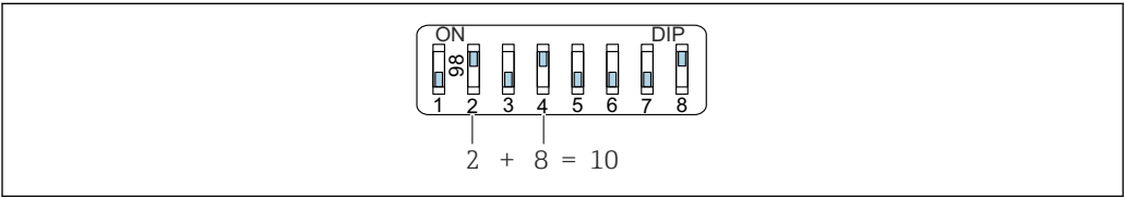
图 12 硬件地址设定示意图；开关 8 拨至“ON”位置，使用开关 1...7 设置设备地址
