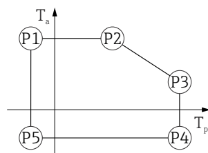
图 43 316L 外壳；过程温度：-40 ... +450 °C (-40 ... +842 °F)
