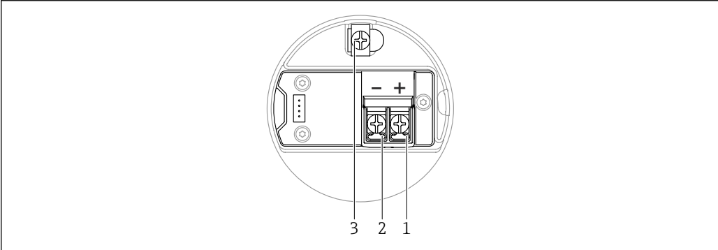
图 9 接线腔中的接线端子和接地端
