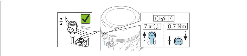
图 6 带锁定螺丝的外壳盖；卫生型外壳（仅适用粉尘防爆场合）
