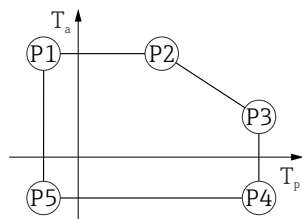
图 39 316L 外壳; 过程温度范围: -40 ... +80 °C (-40 ... +176 °F)
