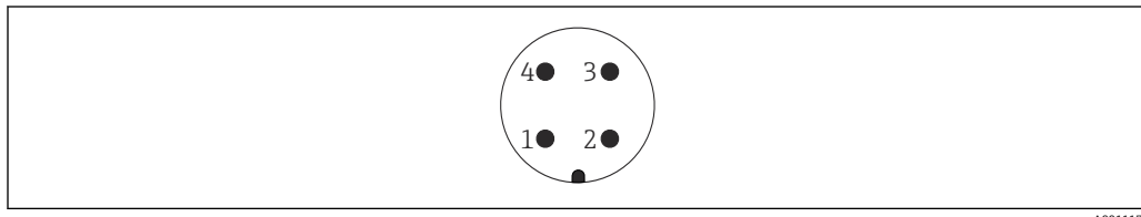
图 10 仪表连接插头示意图
