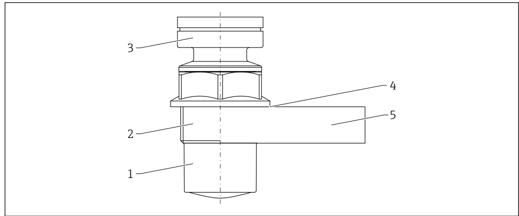
图 36 PVDF 全密封天线（40 mm (1.5 in) 口径）的材质
