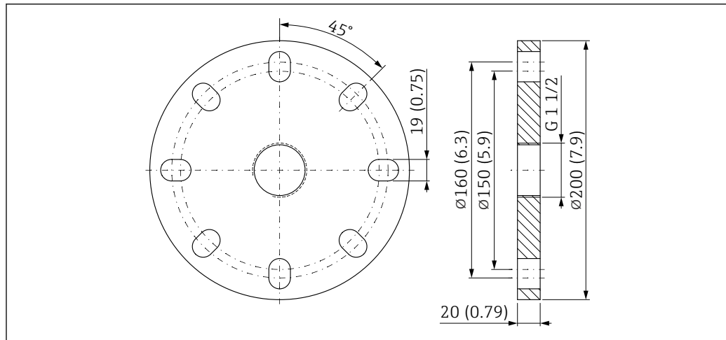
图 33 UNI 3"/DN80/80A 法兰的外形尺寸示意图。测量单位 mm (in)
