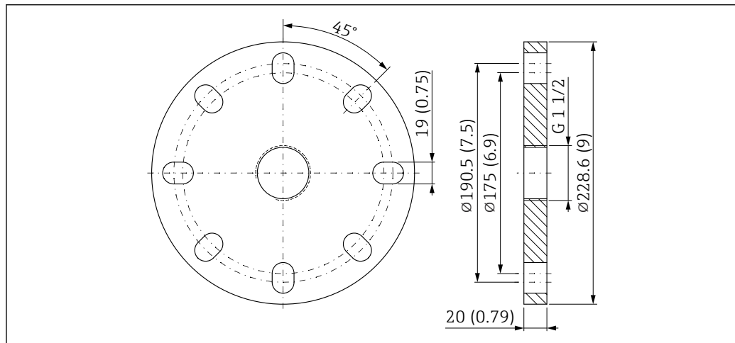
图 34 UNI 4"/DN100/100A 法兰的外形尺寸示意图。测量单位 mm (in)
