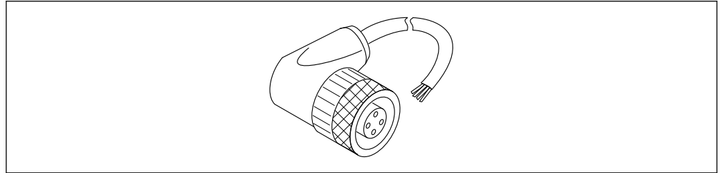
图 48 M12 插座（100 度弯角），5 m (16 ft) 电缆
