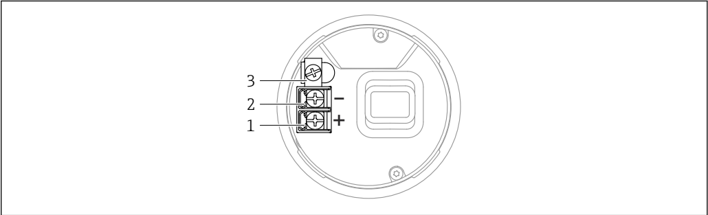
📌 3 接线腔内的接线端子和接地端，单腔室外壳
