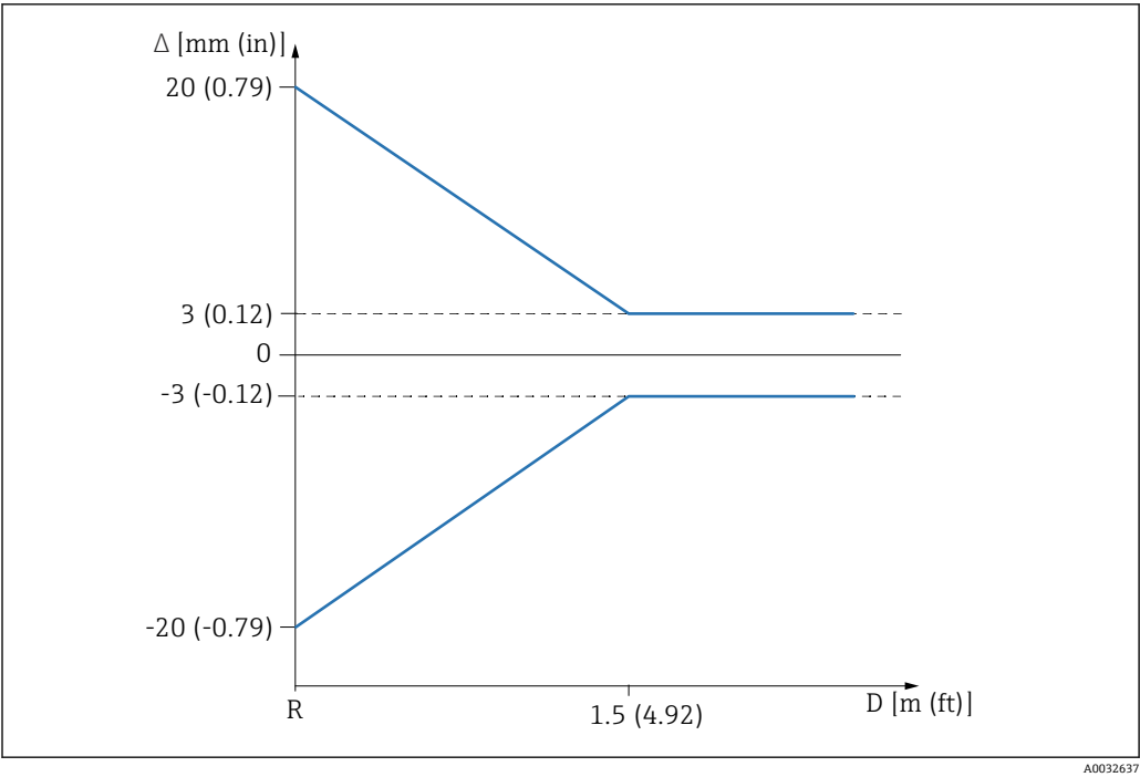
图 8 近距离测量时的最大测量误差
