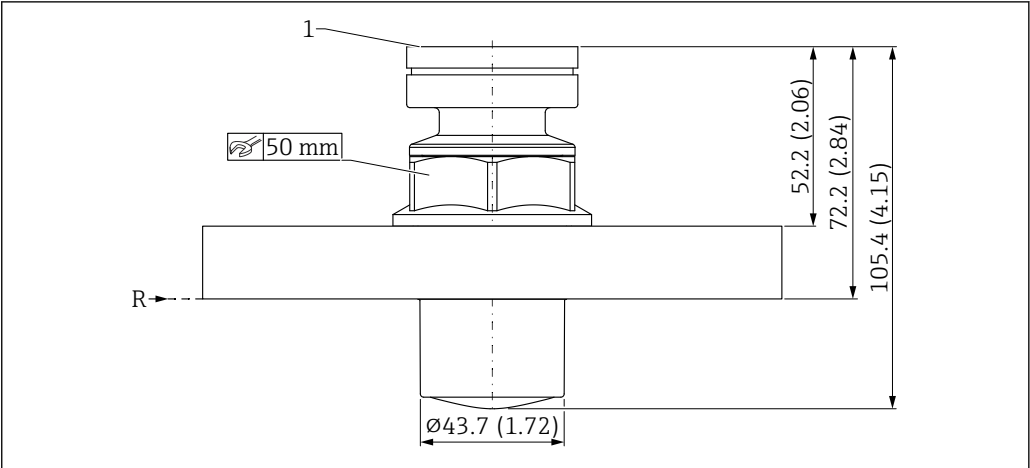
27 PVDF 全密封天线 (40 mm (1.5 in)口径) 的外形尺寸示意图；UNI 法兰过程连接。测量单位 mm (in) R 测量参考点 1 外壳底部
