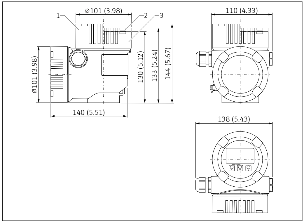
图 24 L 型双腔室铝外壳（带涂层）的外形尺寸示意图；包括 M20 接头和塑料插头。测量单位 mm (in)
