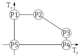
图 11 塑料外壳；过程温度范围：0 ... +80 °C (+32 ... +176 °F)，适用 CSA C/US 认证型仪表
