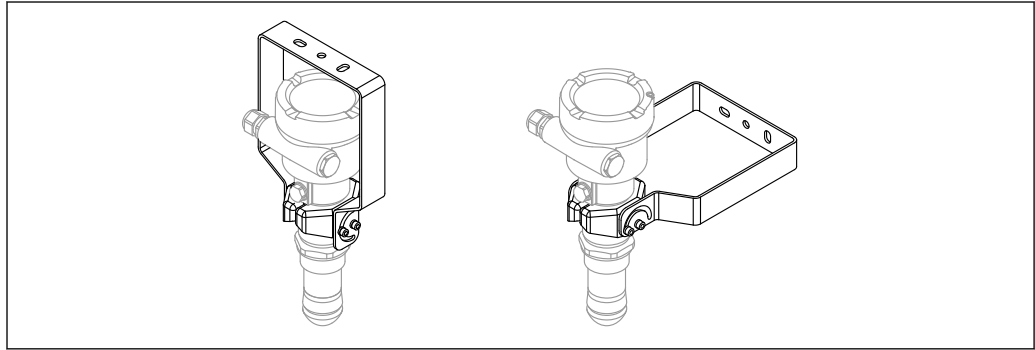
图 43 FMR6xB 的安装架（可调节）；安装在罐顶或墙壁上
