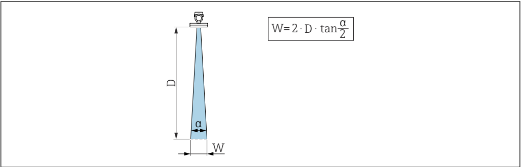
图 9 波束角 \alpha 、距离 D 和波束宽度 W 的相互关系
