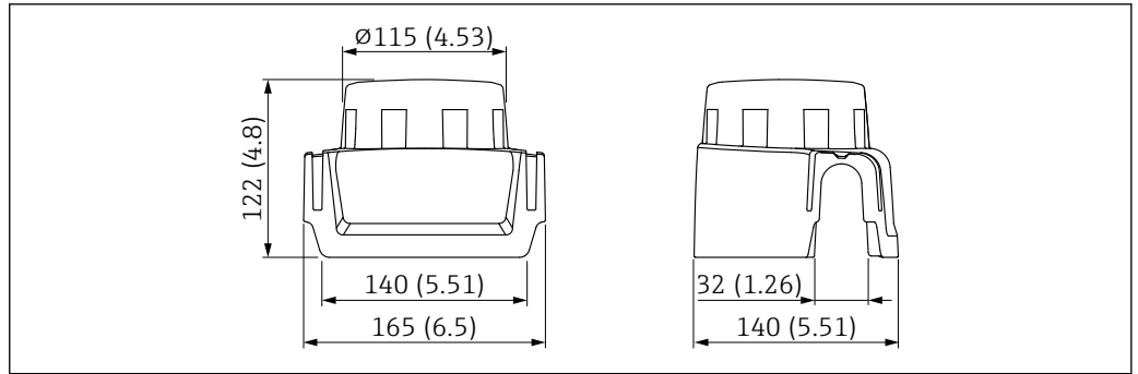
图 42 塑料防护罩 XW111 的外形尺寸示意图。测量单位 mm (in)
