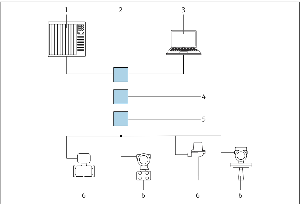
图 40 通过 PROFINET + Ethernet-APL 网络实现远程操作：星形拓扑结构
