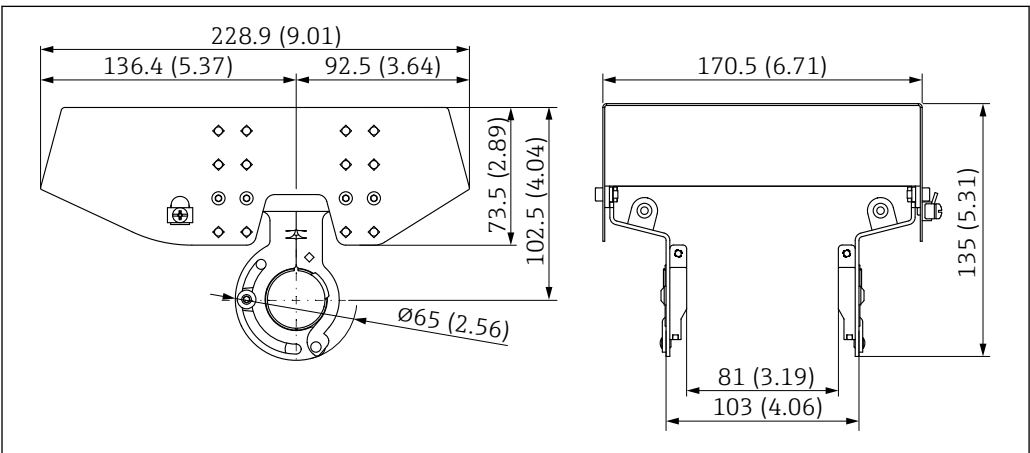
图 41 316L 防护罩 XW112 的外形尺寸示意图。测量单位 mm (in)
