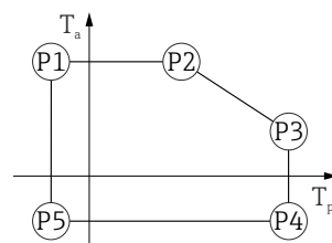
图 15 铝外壳, 带涂层; 过程温度范围: -40 \dots +130 \text{ }^{\circ}\text{C} ( -40 \dots +266 \text{ }^{\circ}\text{F} )
