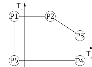
图 14 铝外壳, 带涂层; 过程温度范围: -40 \dots +80 \text{ }^{\circ}\text{C} ( -40 \dots +176 \text{ }^{\circ}\text{F} )
