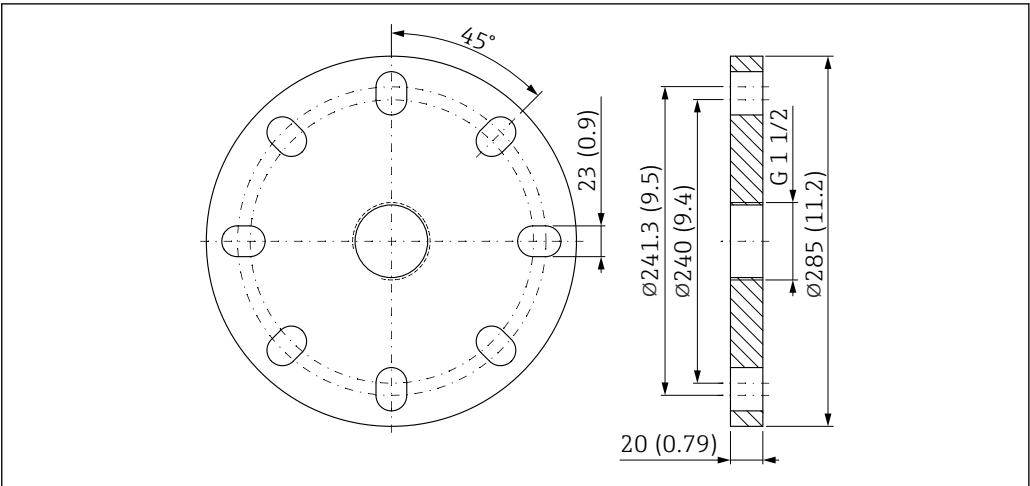
图 35 UNI 6"/DN150/150A 法兰的外形尺寸示意图。测量单位 mm (in)
