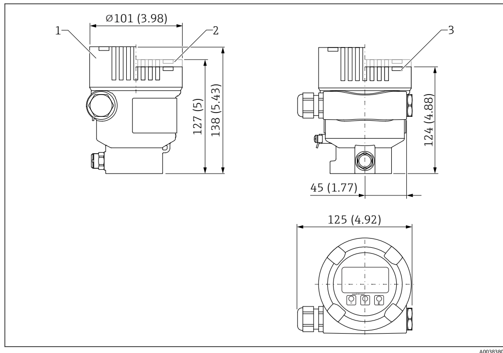
图 21 单腔室铝外壳（带涂层）的外形尺寸示意图；包括 M20 接头和塑料插头。测量单位 mm (in)
