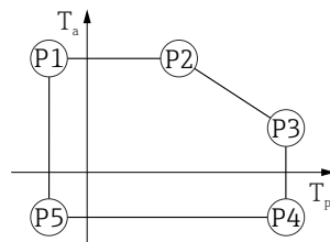
图 12 塑料外壳；过程温度范围：-40 ... +130 °C (-40 ... +266 °F)
