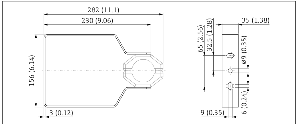
图 44 外形尺寸示意图；FMR6xB 的安装架（可调节）。测量单位 mm (in)
