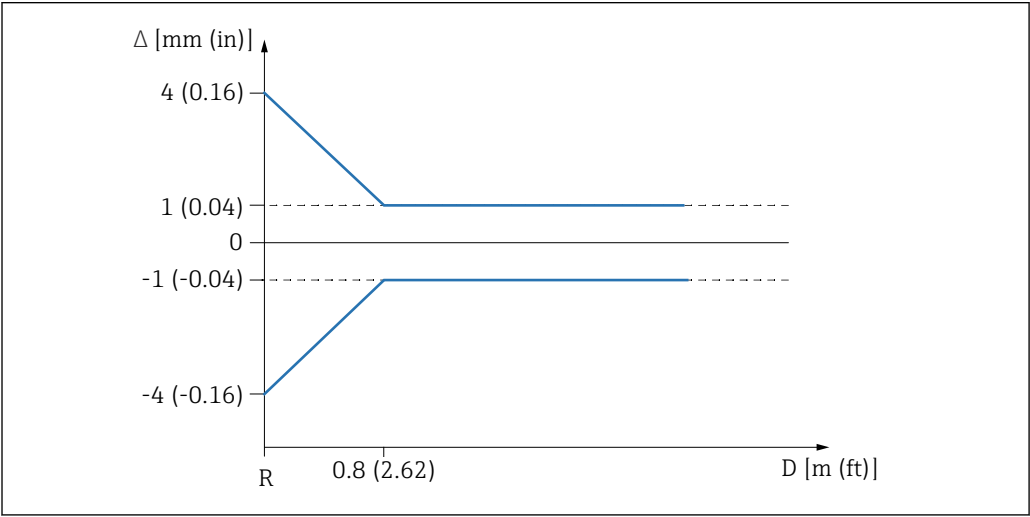
17 近距离测量时的最大测量误差
