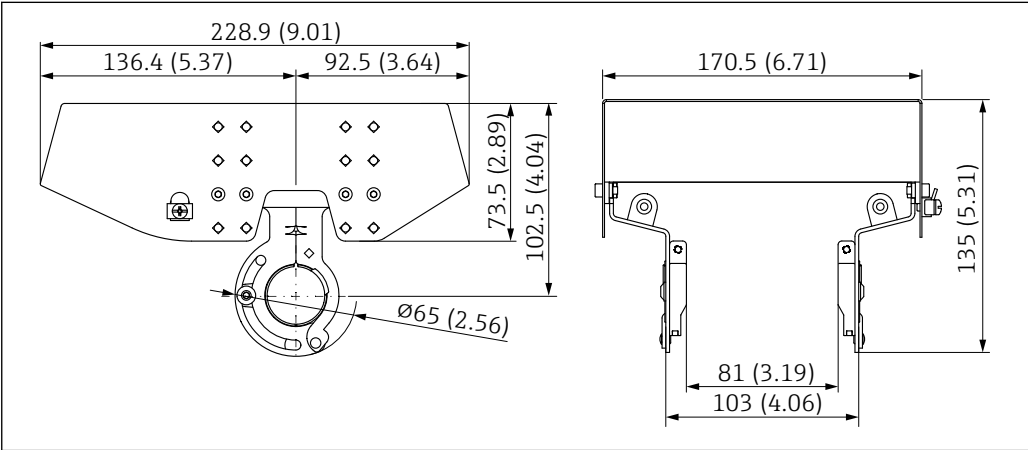
图 74 316L 防护罩 XW112 的外形尺寸示意图。测量单位 mm (in)
