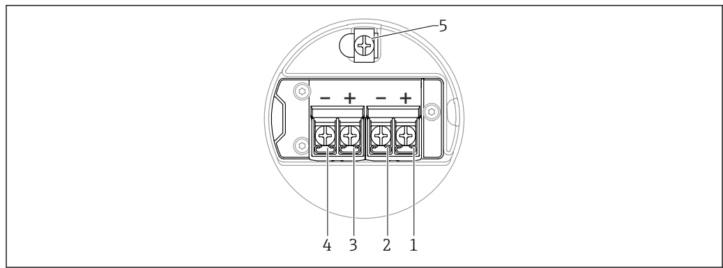
图 7 接线腔中的接线端子分配; 4 ... 20 mA HART, 开关量输出, 双腔室外壳
