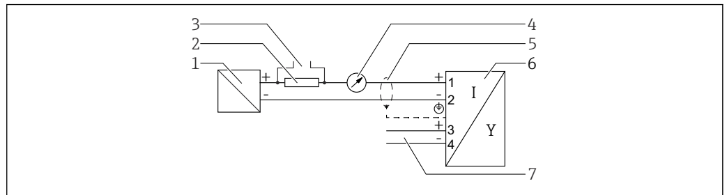
图 13 功能框图: 4 ... 20 mA HART, 开关量输出
