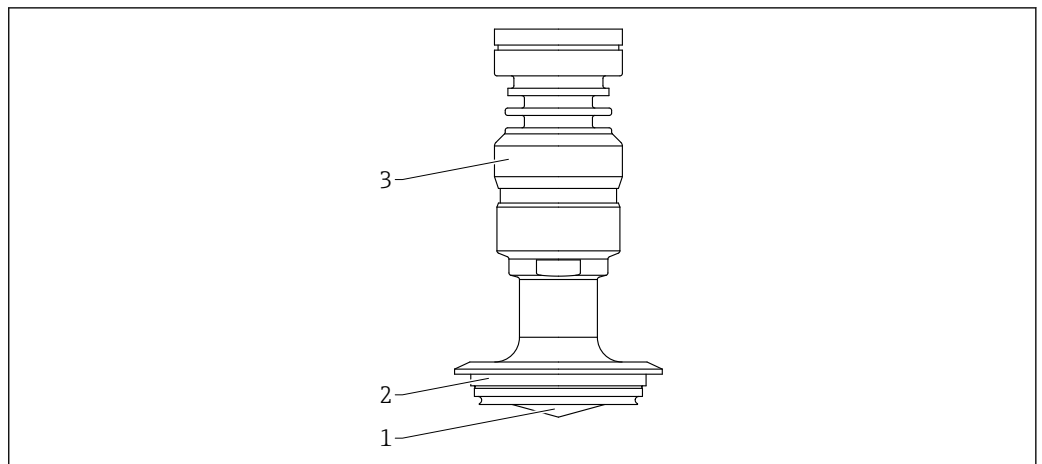
▣ 69 PEEK 涂层天线的材质；齐平安装，40 mm (1.5 in)口径，带 Varivent N DN65-162 接头
