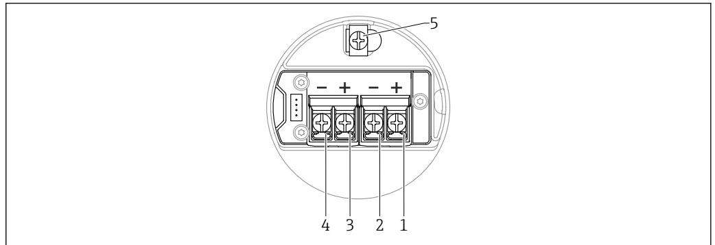
图 9 接线腔中的接线端子分配; 4 ... 20 mA HART + 4 ... 20 mA 模拟量; 双腔室外壳 (L 型)
