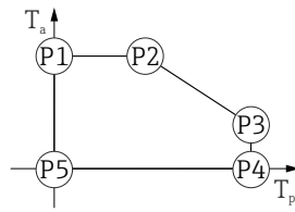
图 20 塑料外壳；过程温度范围： 0 \dots +150 \text{ }^{\circ}\text{C} ( +32 \dots +302 \text{ }^{\circ}\text{F} )，适用 CSA C/US 认证型仪表
