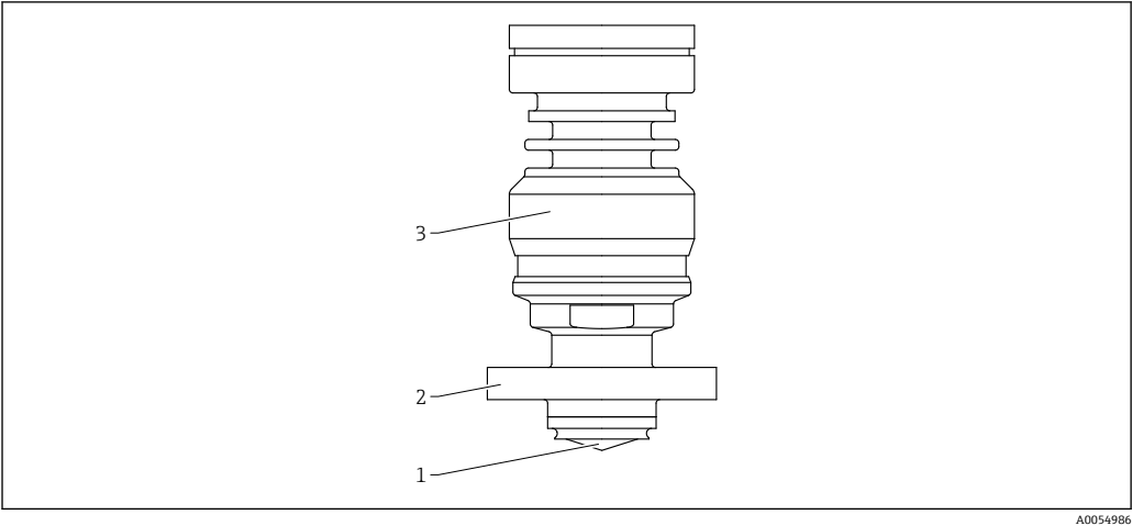
图 70 PEEK 涂层天线的材质；齐平安装，20 mm (0.75 in)口径，带 NEUMO BioControl D25 卫生型连接
