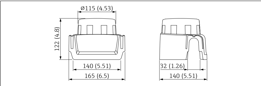
图 75 塑料防护罩 XW111 的外形尺寸示意图。测量单位 mm (in)
