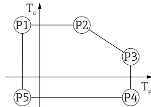
图 19 塑料外壳；过程温度范围：-10 ... +150 °C (+14 ... +302 °F)
