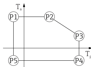
43 316L 外壳, 卫生型; 过程温度范围: -10 ... +150 °C (+14 ... +302 °F)
