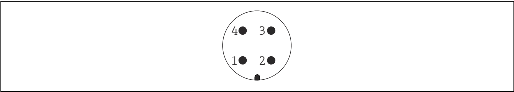
11 仪表连接插头示意图
