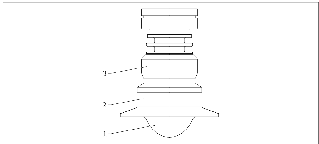
图 67 PTFE 涂层天线的材质；齐平安装，50 mm (2 in)口径，带 ISO2852 Tri-Clamp 卡箍。测量单位 mm (in)
