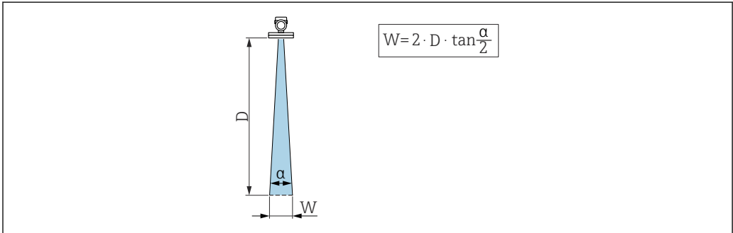
图 18 波束角 \alpha 、距离 D 和波束宽度 W 的相互关系
