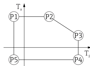
图 48 316L 外壳，卫生型；过程温度范围：-40 ... +200 °C (-40 ... +392 °F)
