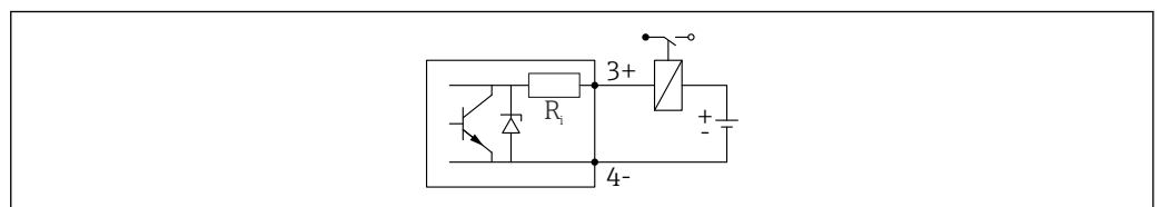
14 继电器的连接示例
