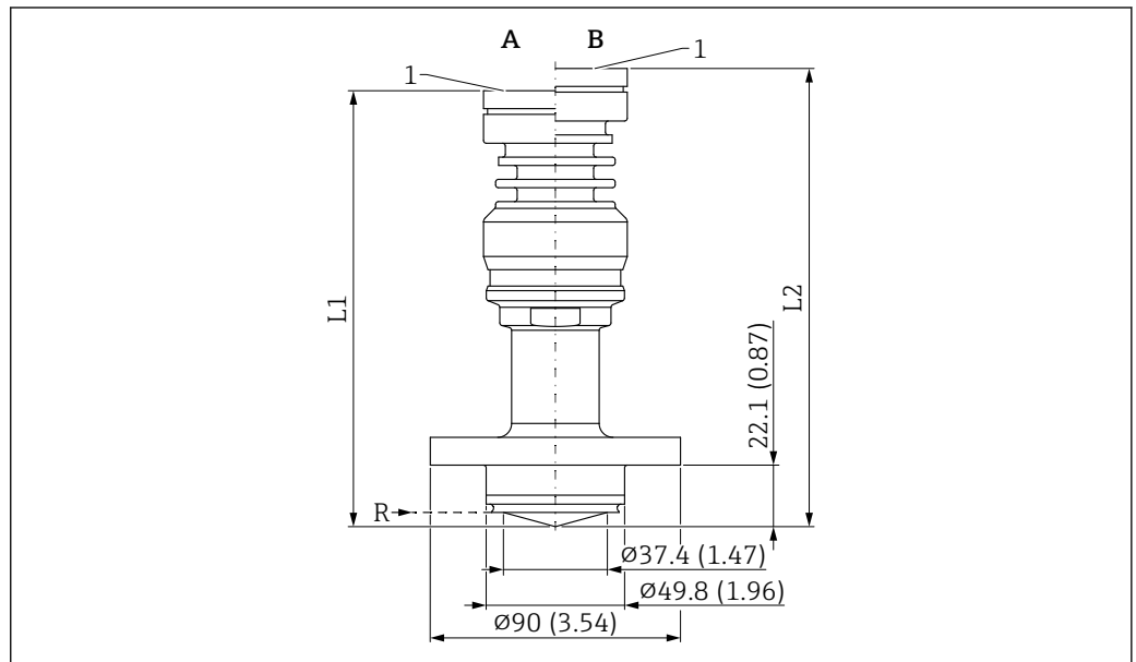
63 PEEK 涂层天线的外形尺寸示意图；齐平安装，40 mm (1.5 in) 口径，带 NEUMO BioControl D50 卫生型连接。测量单位 mm (in)
