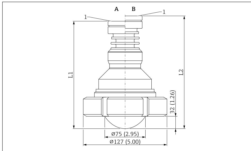
图 57 PTFE 涂层天线（齐平安装，80 mm (3 in)口径）的外形尺寸示意图；带 DIN11851 开槽螺母。测量单位 mm (in)
