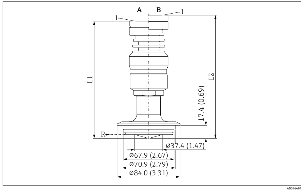
图 61 PEEK 涂层天线的外形尺寸示意图；齐平安装，40 mm (1.5 in) 口径，带 Varivent N DN65-162 接头。 测量单位 mm (in)
