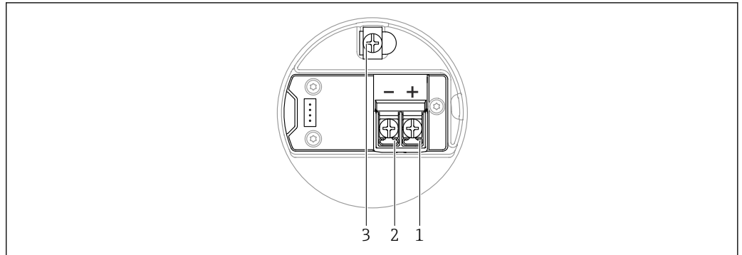
图 8 接线腔中的接线端子分配; 4 ... 20 mA HART; 双腔室外壳 (L 型)
