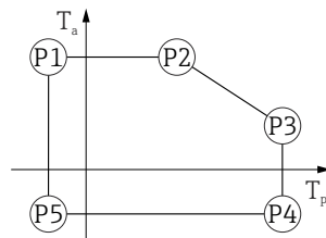
▣ 46 316L 外壳, 卫生型; 过程温度范围: -20 ... +200 °C (-4 ... +392 °F)
