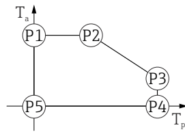
图 26 塑料外壳; 过程温度范围: 0 \dots +200 \text{ }^{\circ}\text{C} ( +32 \dots +392 \text{ }^{\circ}\text{F} ), 适用 CSA C/US 认证型仪表
