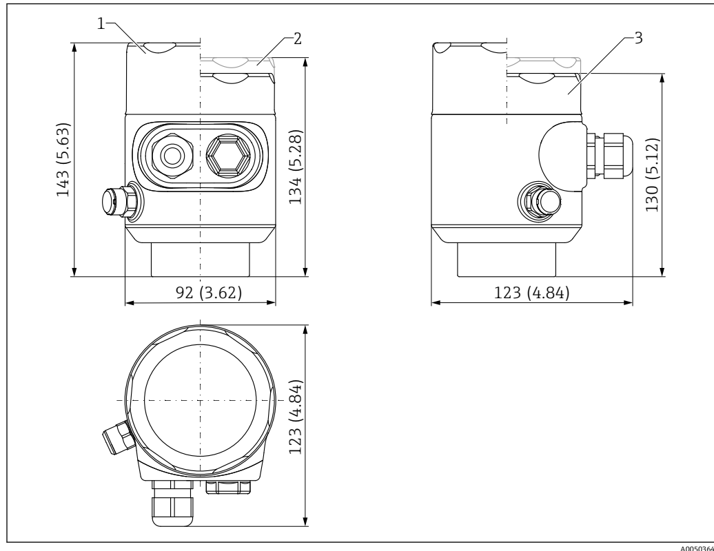
图 51 316L 单腔室外壳（卫生型）的外形尺寸示意图；包括 M20 接头和塑料插头。测量单位 mm (in)
