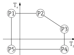
图 47 316L 外壳，卫生型；过程温度范围：-40 ... +150 °C (-40 ... +302 °F)
