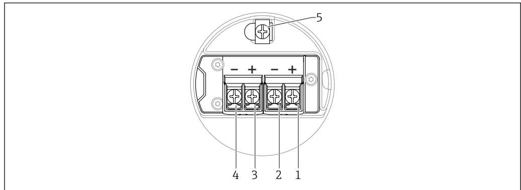
图 6 接线腔中的接线端子分配; 4 ... 20 mA HART + 4 ... 20 mA 模拟量; 双腔室外壳
