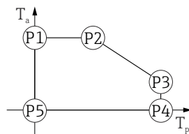
图 28 塑料外壳; 过程温度范围: 0 \dots +150 \text{ }^{\circ}\text{C} ( +32 \dots +302 \text{ }^{\circ}\text{F} ), 适用 CSA C/US 认证型仪表
