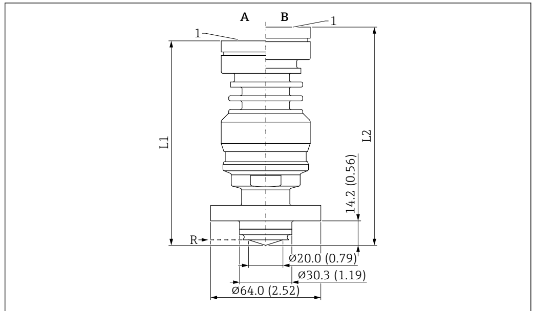
62 PEEK 涂层天线的外形尺寸示意图；齐平安装，20 mm (0.75 in) 口径，带 NEUMO BioControl D25 卫生型连接。测量单位 mm (in)
