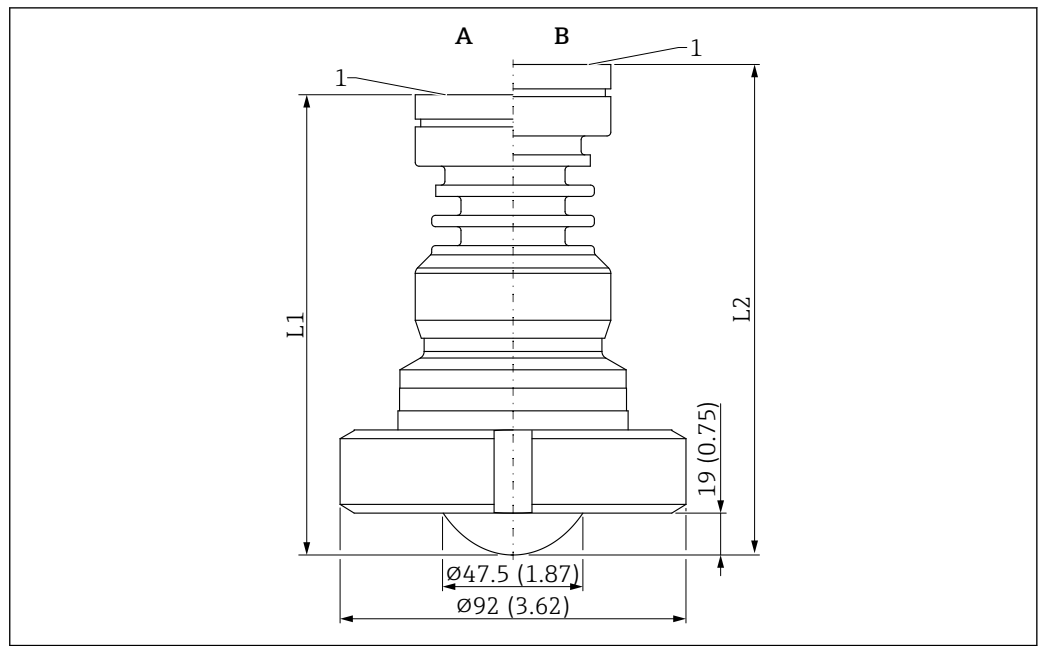
56 PTFE 涂层天线（齐平安装，50 mm (2 in)口径）的外形尺寸示意图；带 DIN11851 开槽螺母。测量单位 mm (in)
