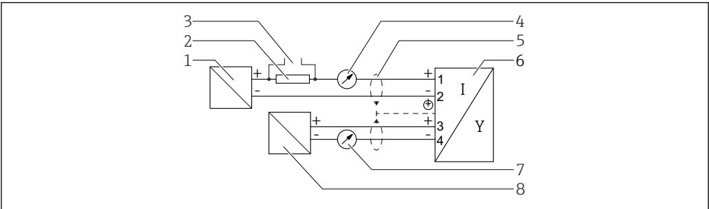
16 功能框图: 4 ... 20 mA HART + 4 ... 20 mA 模拟量
