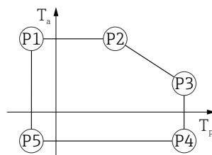
图 31 铝外壳, 带涂层; 过程温度范围: -10 \dots +150 \text{ }^{\circ}\text{C} ( +14 \dots +302 \text{ }^{\circ}\text{F} )
