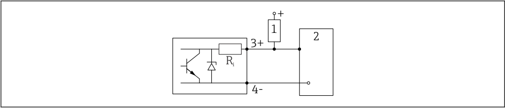
15 数字量输入的连接示例
