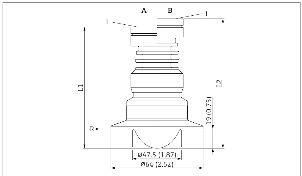
■ 58 PTFE 涂层天线（齐平安装，50 mm (2 in)口径）的外形尺寸示意图；带 ISO2852 Tri-Clamp DN51 (2")卡箍。测量单位 mm (in)
