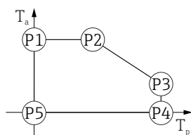
图 31 塑料外壳; 过程温度: 0 ... +280 °C (+32 ... +536 °F), 针对 CSA C/US 认证型仪表
