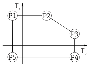
38 铝外壳，带涂层；过程温度范围：-20 ... +150 °C (-4 ... +302 °F)
