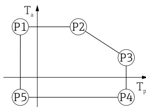
图 54 316L 外壳, 卫生型; 过程温度范围: -20 ... +150 °C (-4 ... +302 °F)
