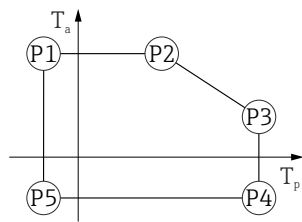
40 铝外壳，带涂层；过程温度范围：-40 ... +150 °C (-40 ... +302 °F)
