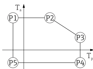
▣ 52 316L 外壳; 过程温度: -60 \dots +150 \text{ }^{\circ}\text{C} ( -76 \dots +302 \text{ }^{\circ}\text{F} )
