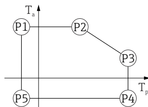
图 30 塑料外壳; 过程温度: -40 ... +280 °C (-40 ... +536 °F)
