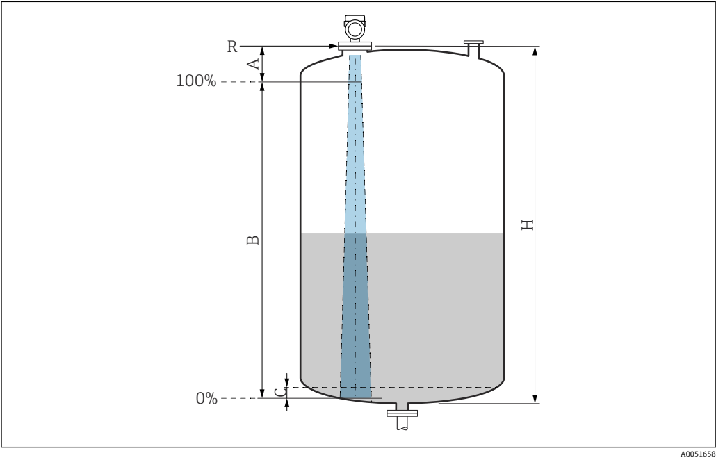
21 有效测量范围 A 天线长度 + 10 mm (0.4 in) B 有效测量范围 C 50 ... 80 mm (1.97 ... 3.15 in); 介质 \epsilon_r < 2 H 罐体高度 R 参考测量点，具体取决于天线系统
