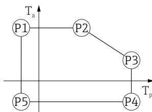
图 55 316L 外壳, 卫生型; 过程温度范围: -20 ... +200 °C (-4 ... +392 °F)
