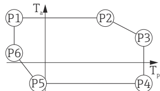
图 45 铝外壳，带涂层；过程温度：-196 ... +200 °C (-320 ... +392 °F)
