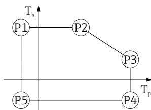
▣ 51 316L 外壳; 过程温度: -40 \dots +450 \text{ }^{\circ}\text{C} ( -40 \dots +842 \text{ }^{\circ}\text{F} )
