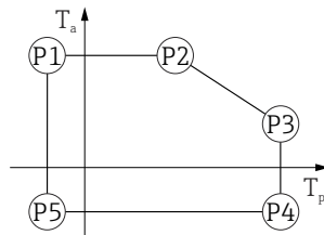
▣ 30 316L 外壳; 过程温度范围: -40 \dots +80 \text{ }^{\circ}\text{C} ( -40 \dots +176 \text{ }^{\circ}\text{F} )
