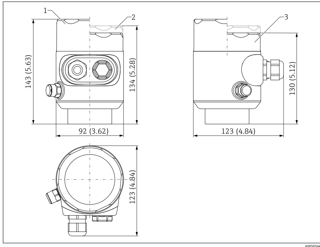
图 42 316L 单腔室外壳（卫生型）的外形尺寸示意图；包括 M20 接头和塑料插头。测量单位 mm (in)
