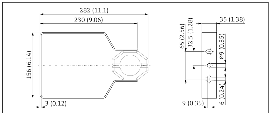
图 67 外形尺寸示意图；FMR6xB 的安装架（可调节）。测量单位 mm (in)
