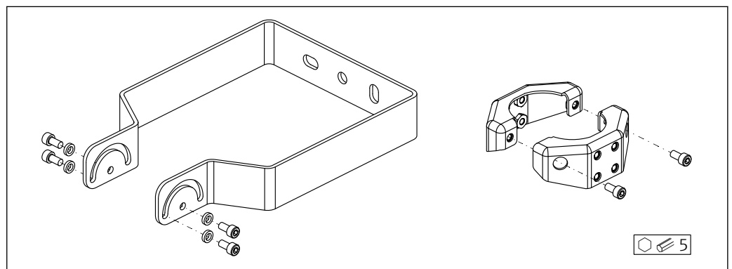
图 68 供货清单；FMR6xB 的安装架（可调节）
