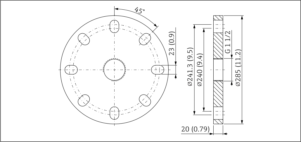
50 UNI 6"/DN150/150A 法兰的外形尺寸示意图。测量单位 mm (in)
