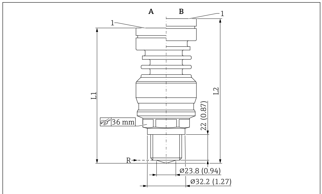
■ 56 PEEK 一体式天线 (20 mm (0.75 in) 口径) 的外形尺寸示意图; ¾"螺纹过程连接。测量单位 mm (in)
