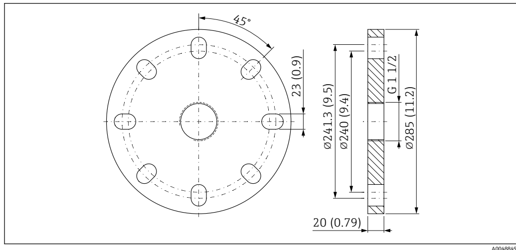
图 55 UNI 6"/DN150/150A 法兰的外形尺寸示意图。测量单位 mm (in)
