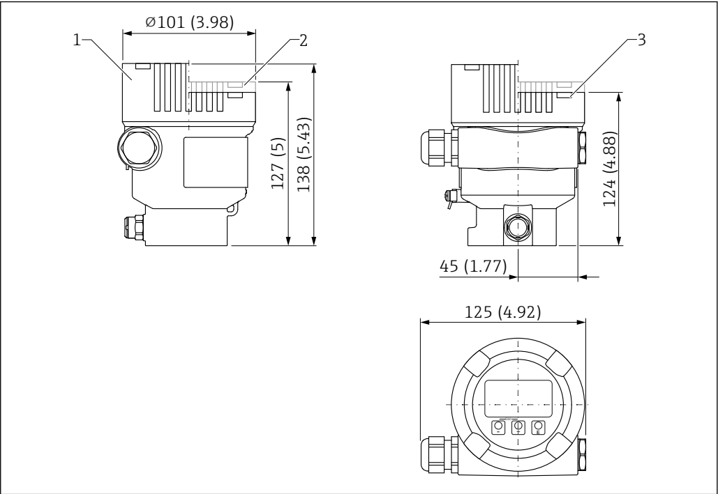
41 单腔室铝外壳（带涂层）的外形尺寸示意图；包括 M20 接头和塑料插头。测量单位 mm (in)
