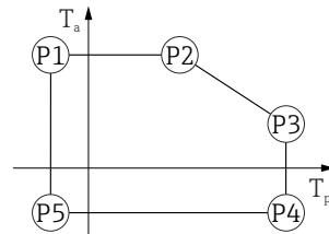
图 20 塑料外壳; 过程温度范围: -40 ... +200 °C (-40 ... +392 °F)
