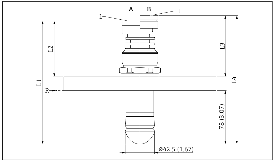
图 52 水滴型天线 (50 mm (2 in)口径) 的外形尺寸示意图; UNI 法兰过程连接。测量单位 mm (in)
