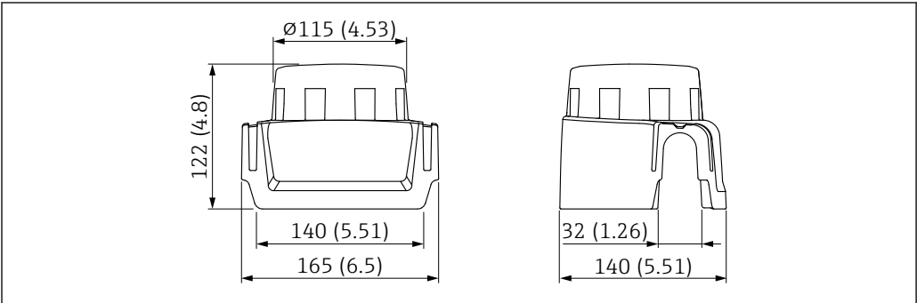
图 65 塑料防护罩 XW111 的外形尺寸示意图。测量单位 mm (in)
