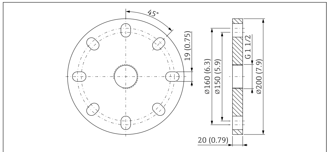
图 48 UNI 3"/DN80/80A 法兰的外形尺寸示意图。测量单位 mm (in)
