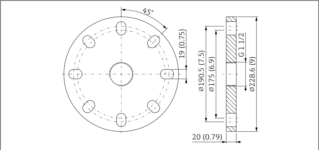
49 UNI 4"/DN100/100A 法兰的外形尺寸示意图。测量单位 mm (in)
