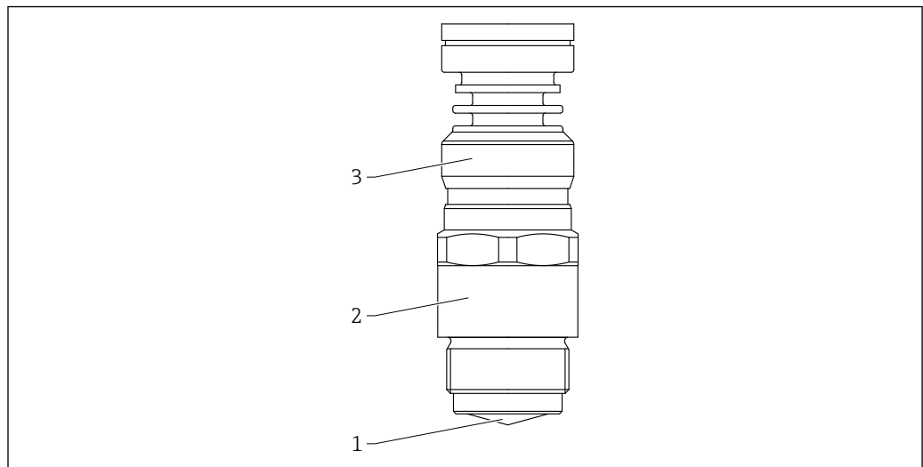
图 61 一体式天线 (40 mm (1.5 in) 口径) 的材质
