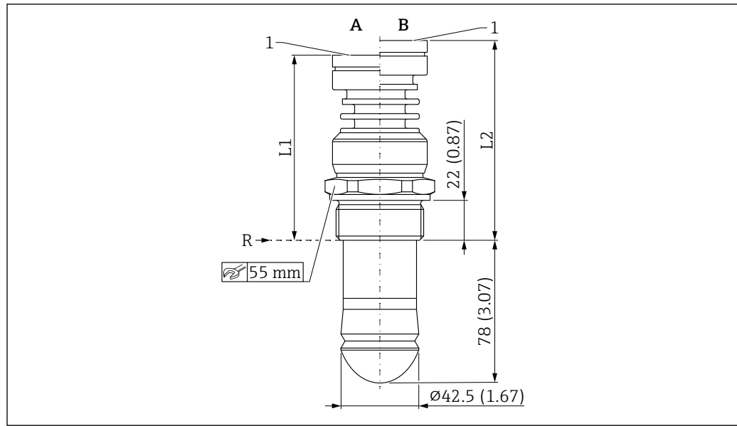
图 51 水滴型天线 (50 mm (2 in)口径) 的外形尺寸示意图，螺纹过程连接
