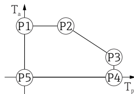
图 15 塑料外壳; 过程温度范围: 0 \dots +80 \text{ }^{\circ}\text{C} ( +32 \dots +176 \text{ }^{\circ}\text{F} ), 适用 CSA C/US 认证型仪表
