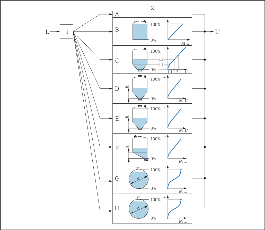
图 50 线性化：将物位和（相关）界面高度转换成体积或重量；转换取决于容器形状。
