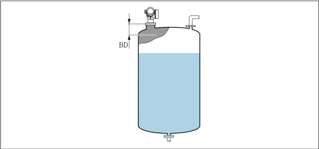
48 液体测量时的盲区距离 (BD)
