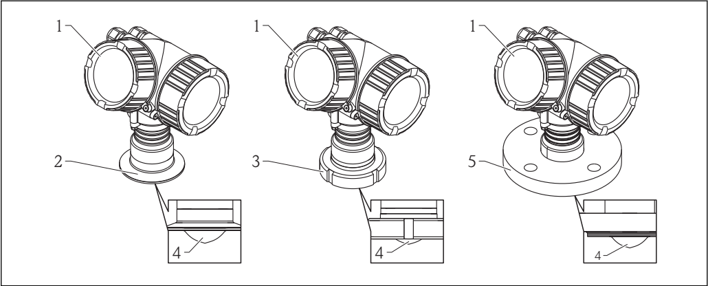
图 2 Micropilot FMR52 (26 GHz) 的结构示意图
