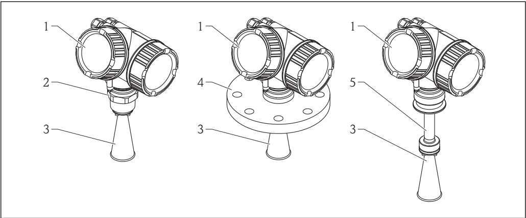
图 1 Micropilot FMR51 (26 GHz) 的结构示意图
