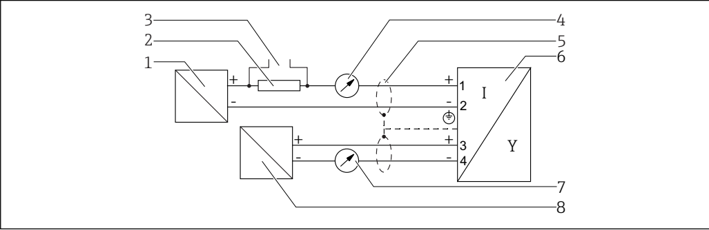
15 接线图: 两线制; 4...20 mA HART, 4...20 mA
