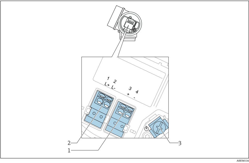
图 16 接线端子分配：四线制；4...20 mA HART (10.4 ... 48 V DC )
