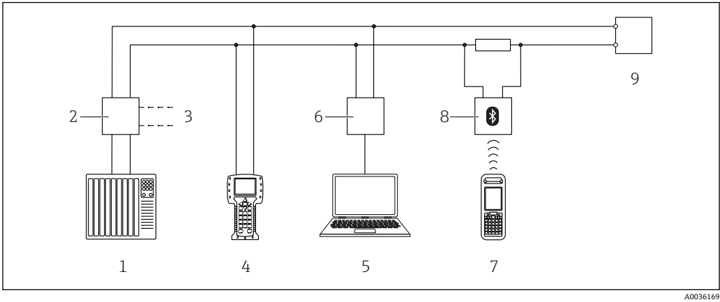
图 27 通过 HART 通信进行远程操作
