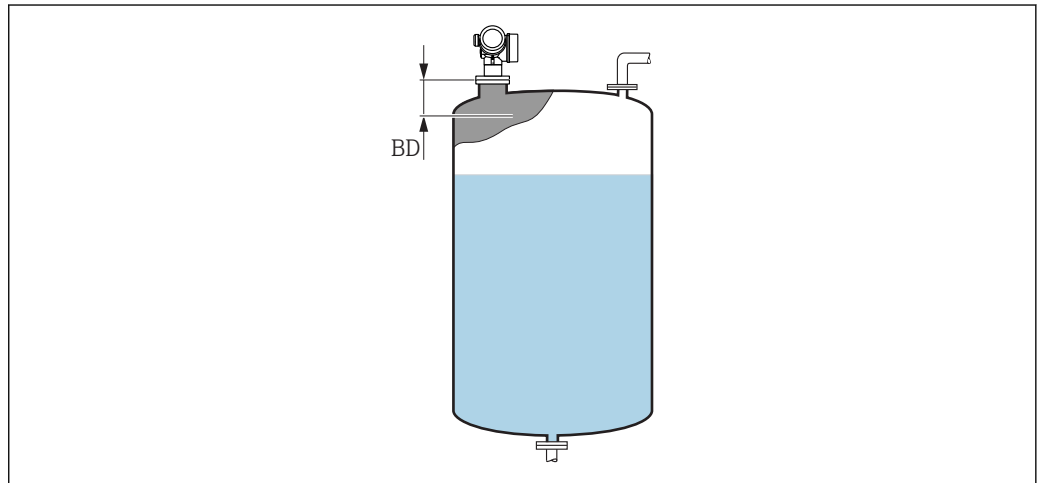
图 52 液体测量时的盲区距离 (BD)
