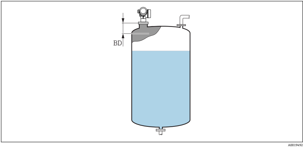
49 液体测量时的盲区距离 (BD)
