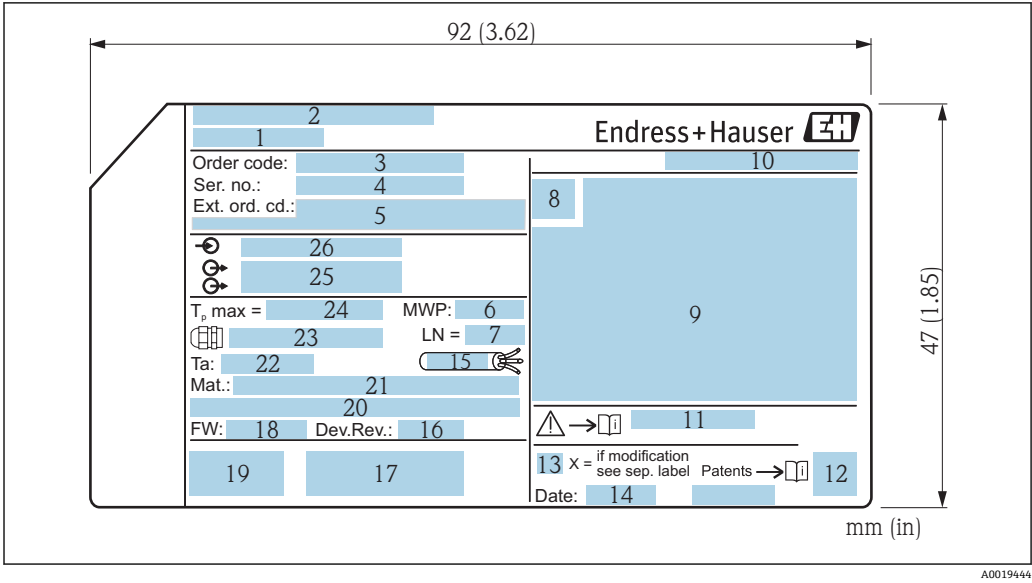
3 Micropilot 的铭牌示意图
