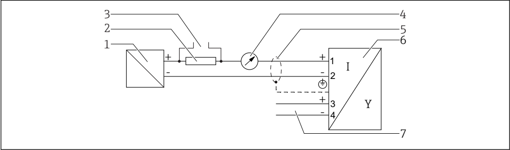
13 接线图：两线制；4...20 mA HART，开关量输出
