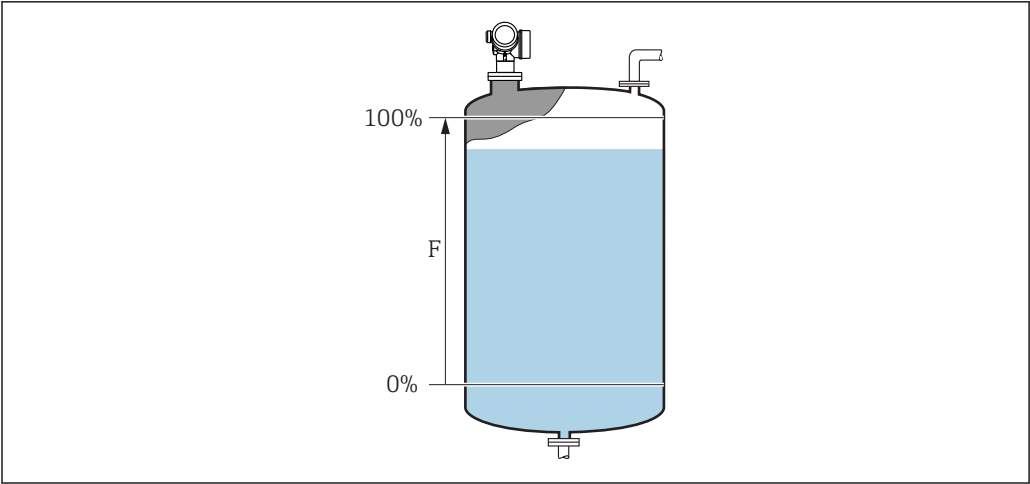
46 液位测量时的满标 (F)
