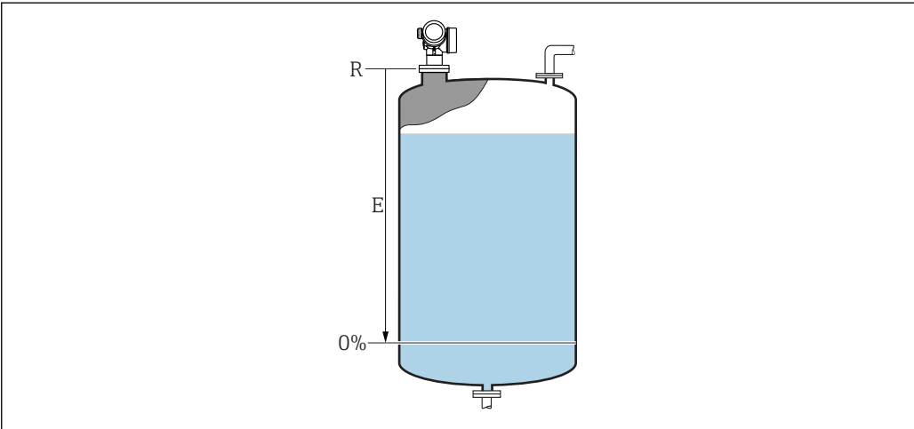
☑ 45 液位测量时的空标 (E)
