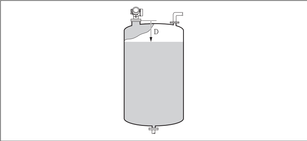
图 48 液位测量时的距离
