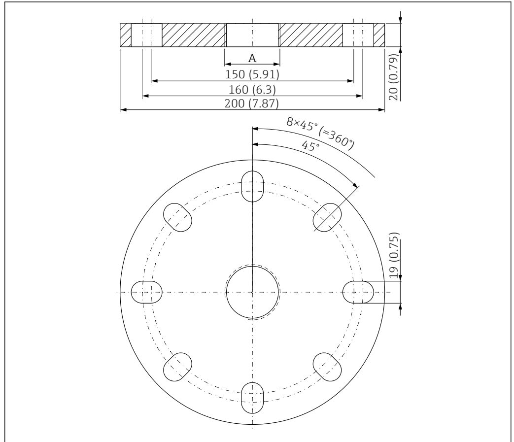
图 39 UNI 3"/DN80/80 法兰的外形尺寸示意图。测量单位 mm (in)
