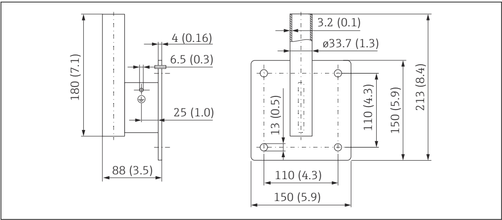
图 34 墙装架的外形尺寸。测量单位 mm (in)
