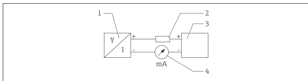
图 7 HART 连接功能框图
