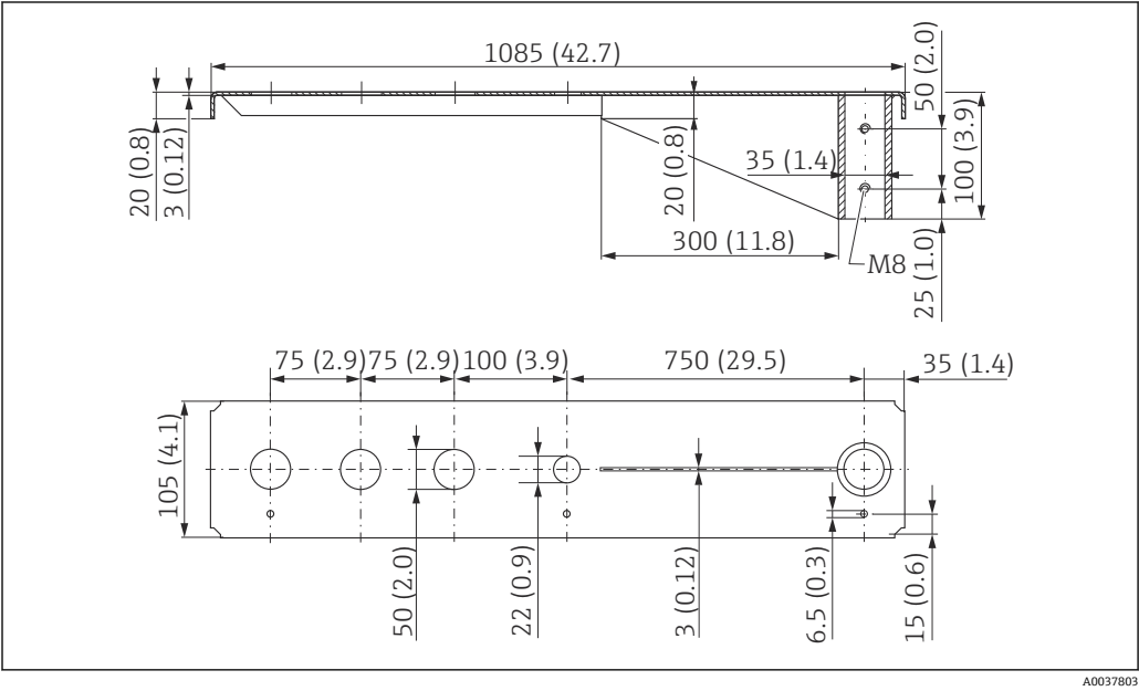
31 1000 mm 旋转悬臂的外形尺寸（安装在 G 1½"传感器天线端过程连接上）。测量单位 mm (in)
