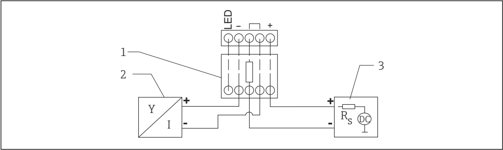
图 10 HART 设备连接安装有 HART 通信电阻的回路显示仪（无背光显示）的功能框图
