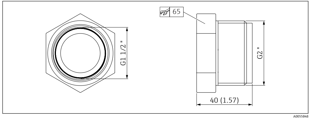
图 24 UNI 转接头的外形尺寸
