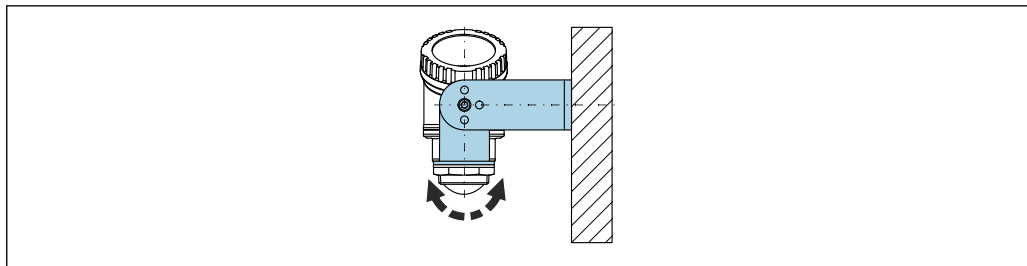
5 使用安装架安装（可调节）
