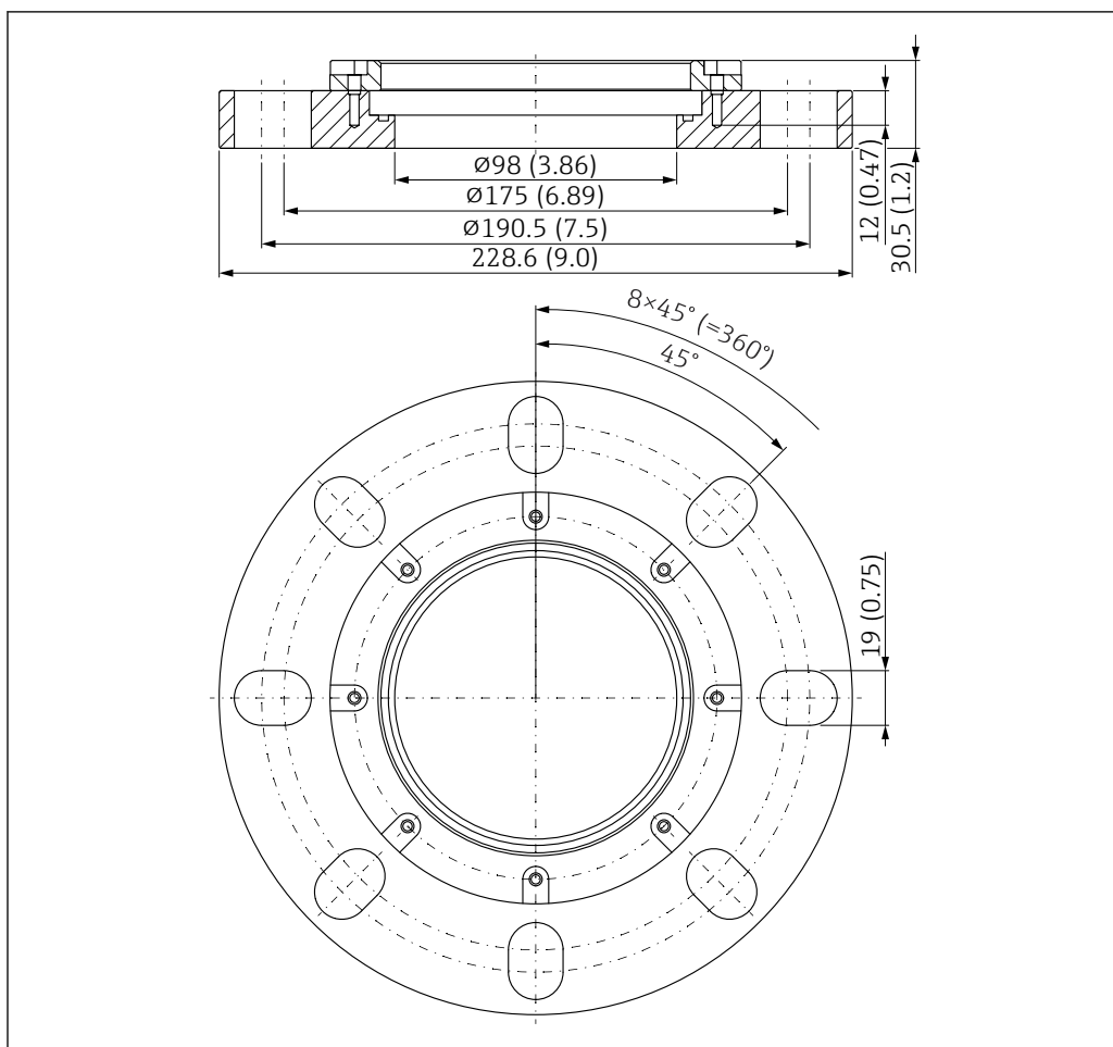
图 36 UNI 4"/DN100/100 松套法兰的外形尺寸示意图。测量单位 mm (in)
