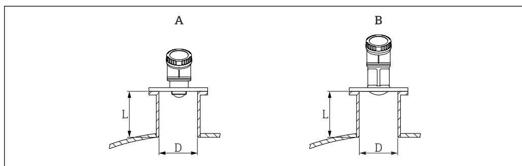
图 3 安装在安装短管中
