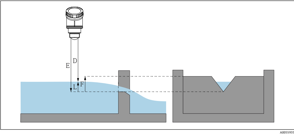
图 20 实例：V 形槽口测量堰
