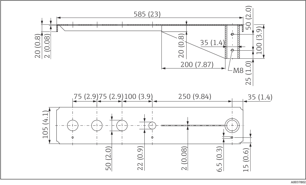
30 500 mm 旋转悬臂的外形尺寸（安装在 G 1½"传感器天线端过程连接上）。测量单位 mm (in)
