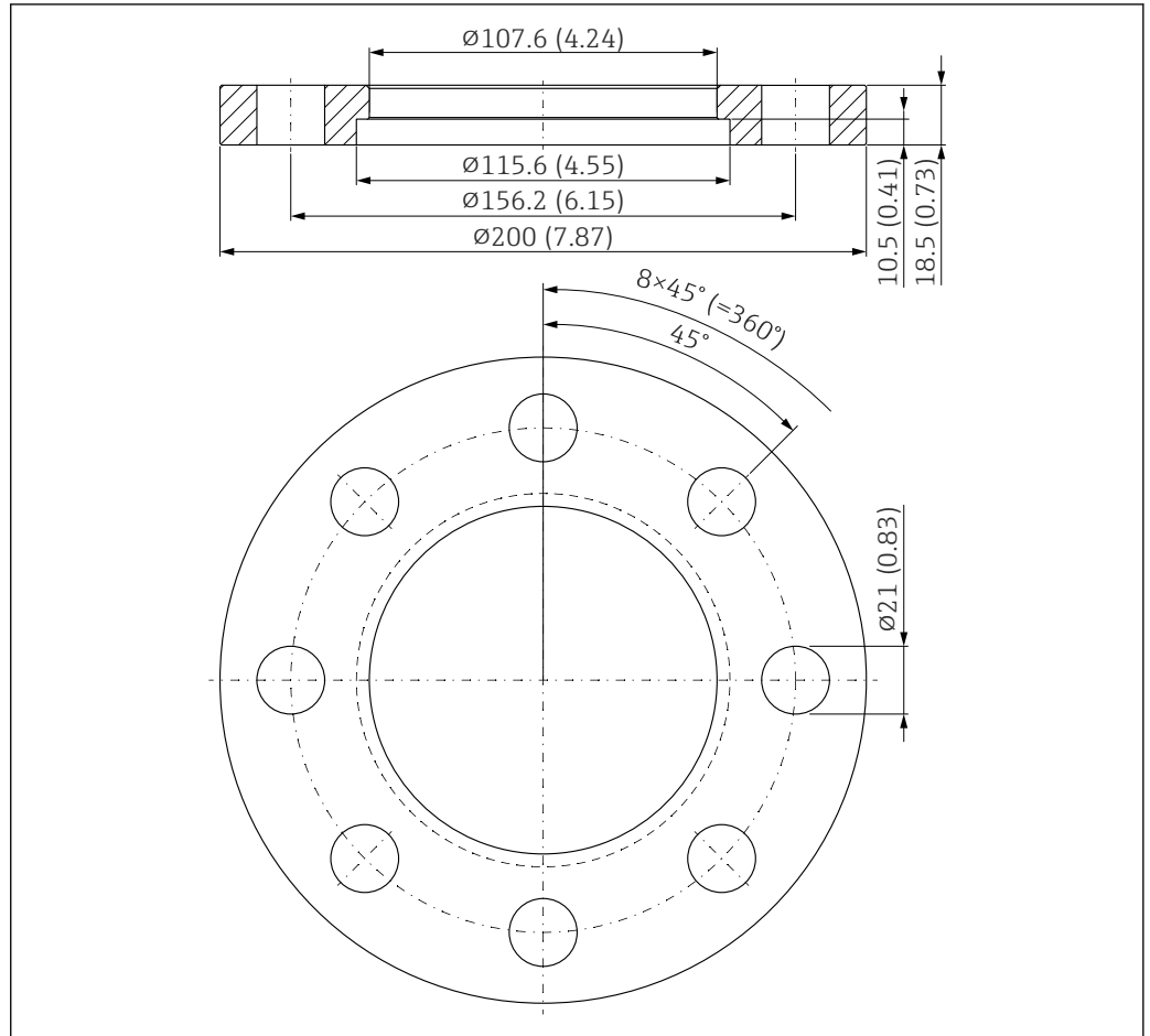
图 35 UNI 3"/DN80/80 松套法兰的外形尺寸示意图。测量单位 mm (in)
