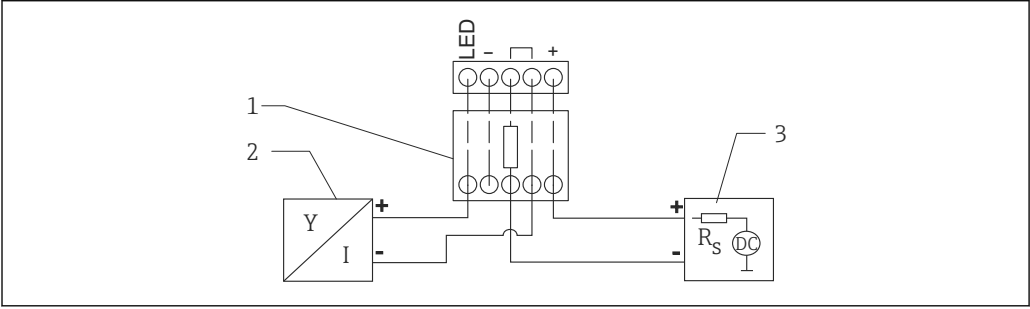
图 11 HART 设备连接安装有 HART 通信电阻的回路显示仪（带背光显示）的功能框图
