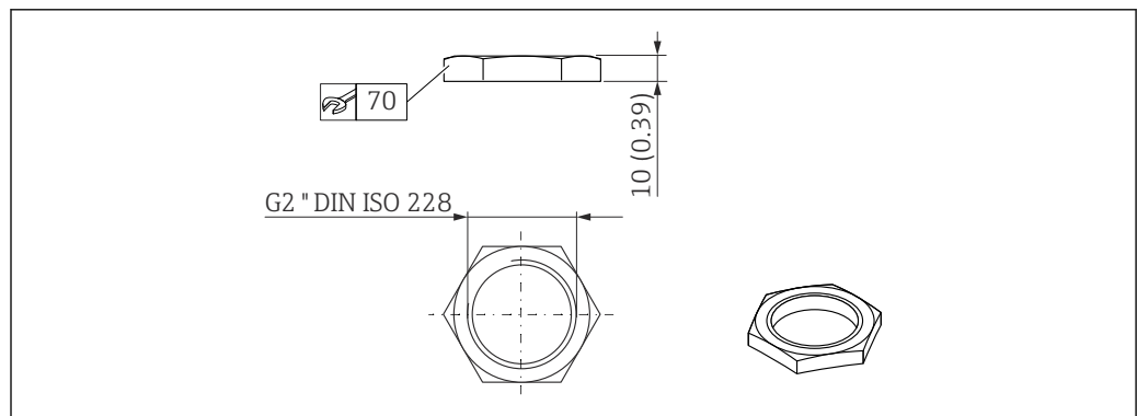
图 23 锁紧螺母的外形尺寸。测量单位 mm (in)
