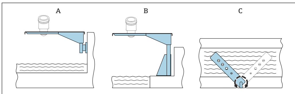
6 使用悬臂安装（可旋转）
