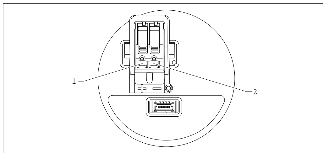
图 12 接线端子分配
