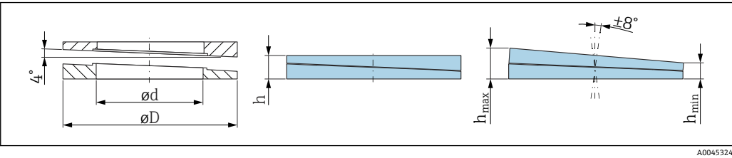
41 外形尺寸
