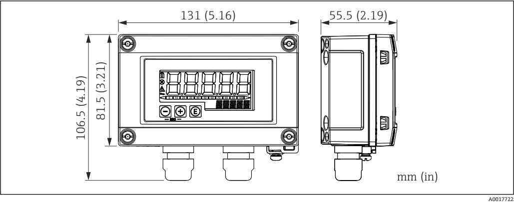
42 RIA15（现场型外壳）的外形尺寸。测量单位 mm (in)
