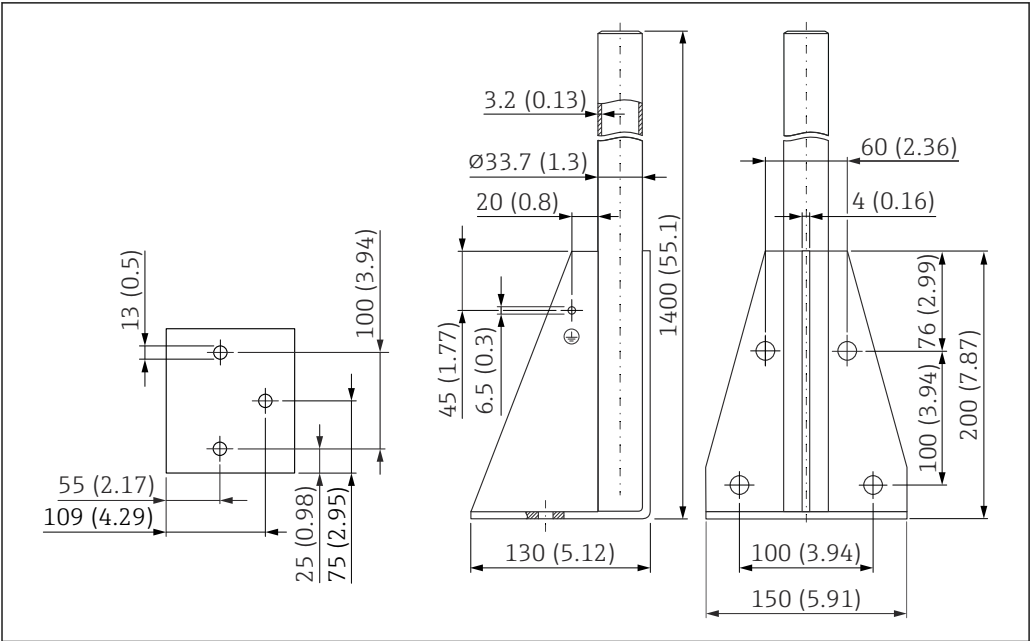
图 33 外形尺寸。测量单位 mm (in)
