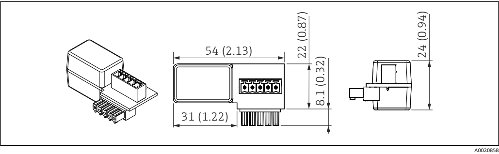
43 HART 通信电阻的外形尺寸。测量单位 mm (in)
