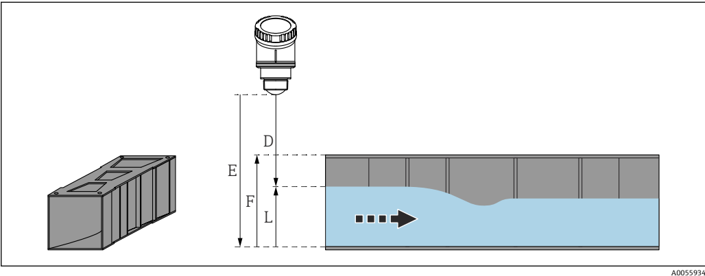
图 19 实例：文丘里水槽
