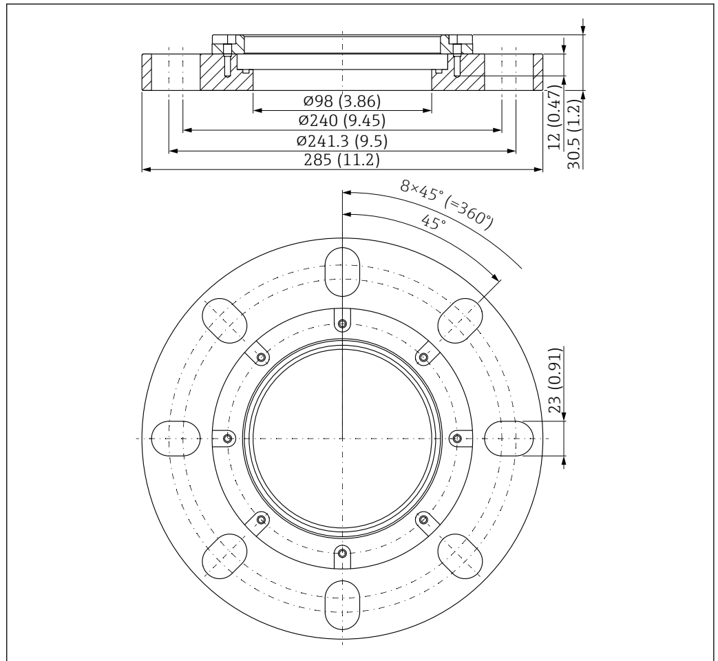
图 37 UNI 6"/DN150/150 松套法兰的外形尺寸示意图。测量单位 mm (in)
