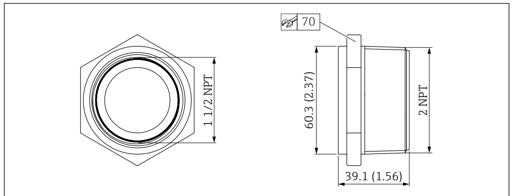
图 25 UNI 转接头的外形尺寸
