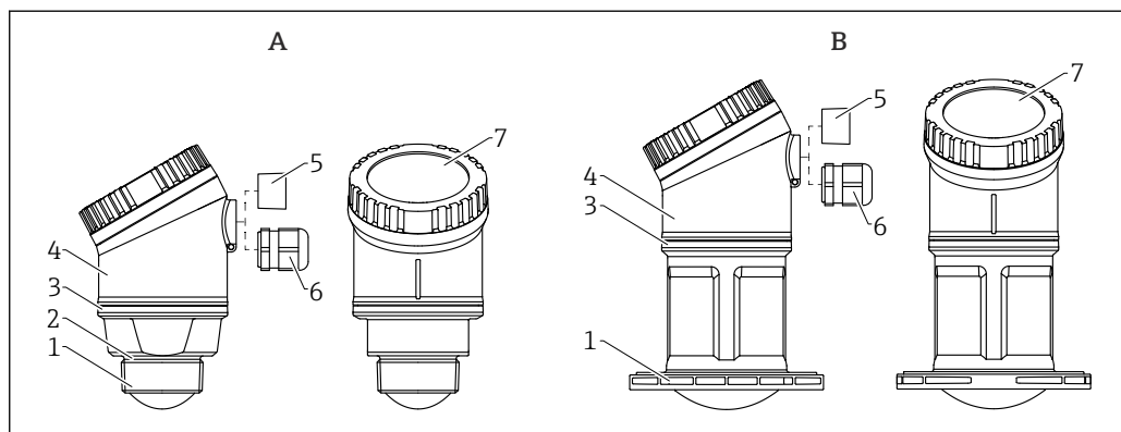
图 1 设备设计
