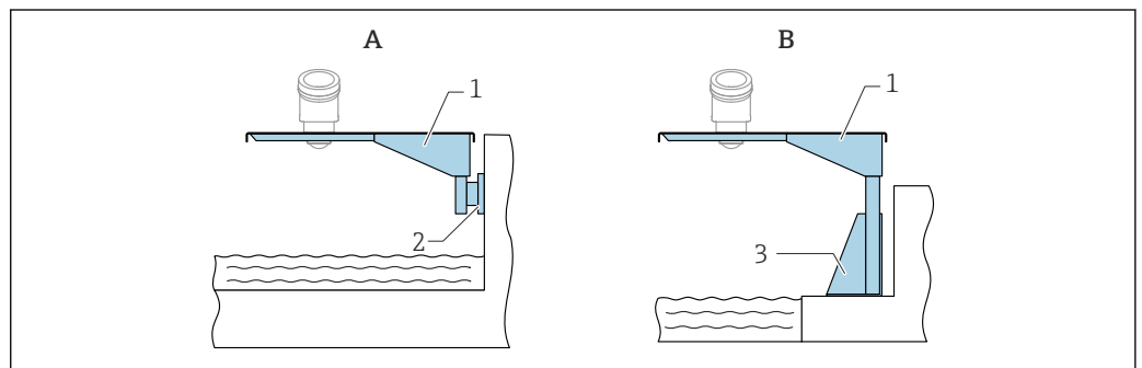
图 29 传感器天线端过程连接的安装方式
