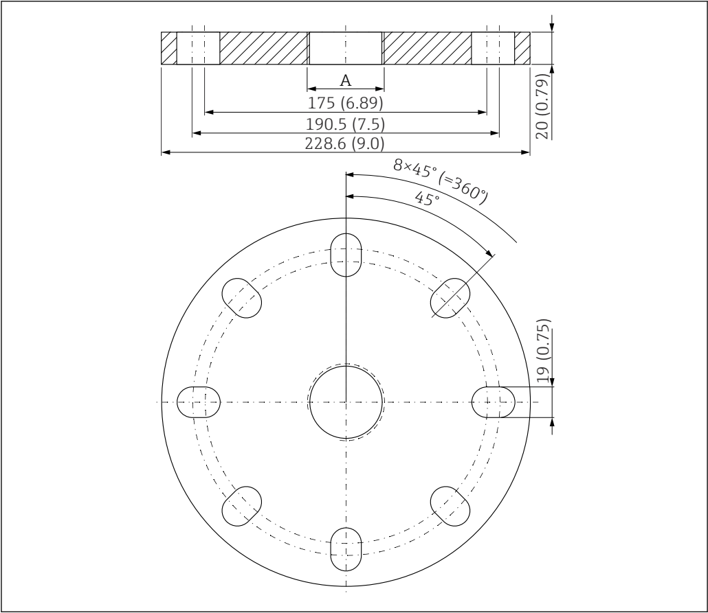
图 40 UNI 4"/DN100/100 法兰的外形尺寸示意图。测量单位 mm (in)
