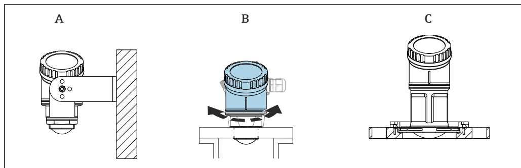
图 2 安装在墙壁上或安装短管中
