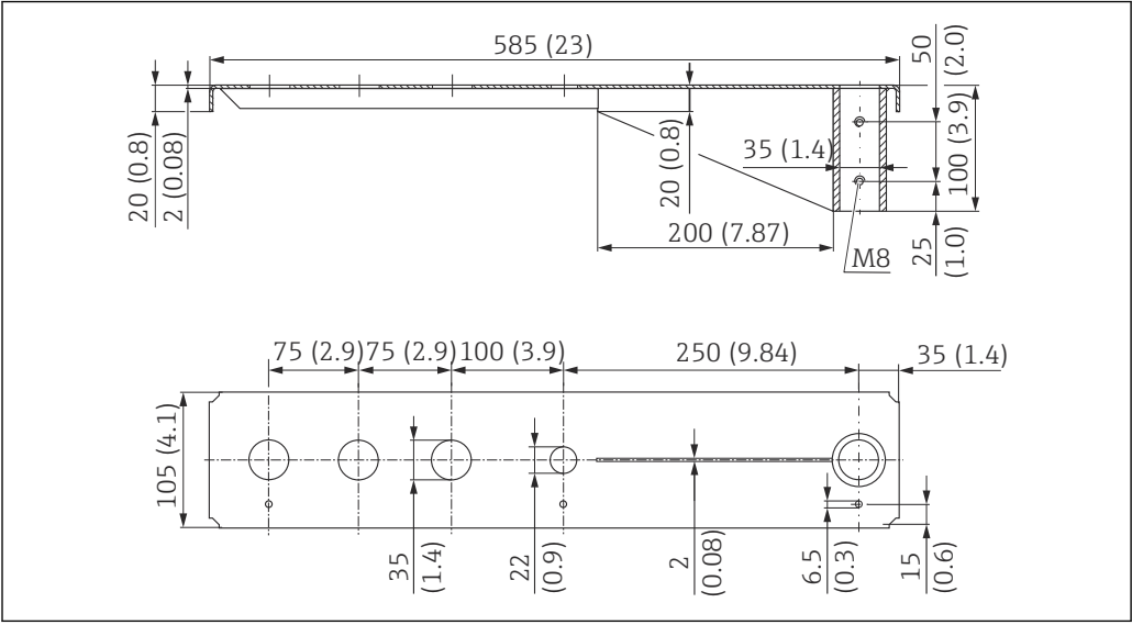
40 500 mm 旋转悬臂的外形尺寸（安装在传感器电缆入口过程连接上）。测量单位 mm (in)
