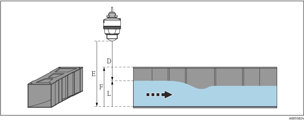
图 23 实例：文丘里水槽
