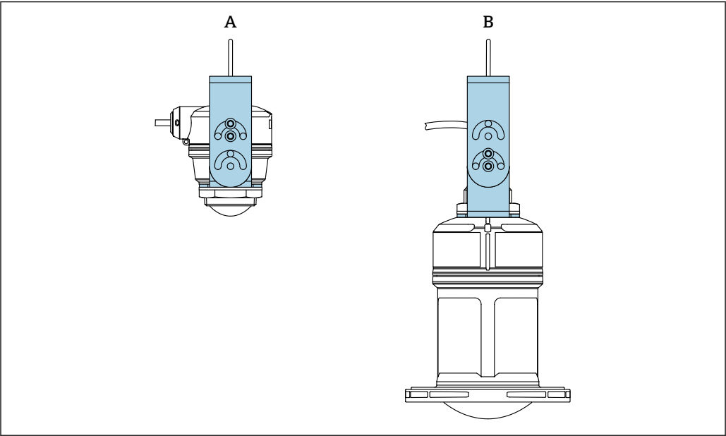
图 7 缆绳悬挂安装 A 使用安装架（可调节）进行缆绳悬挂安装，用于 40 mm (1.5 in) 口径天线 B 使用安装架（可调节）进行缆绳悬挂安装，用于 80 mm (3 in) 口径天线
