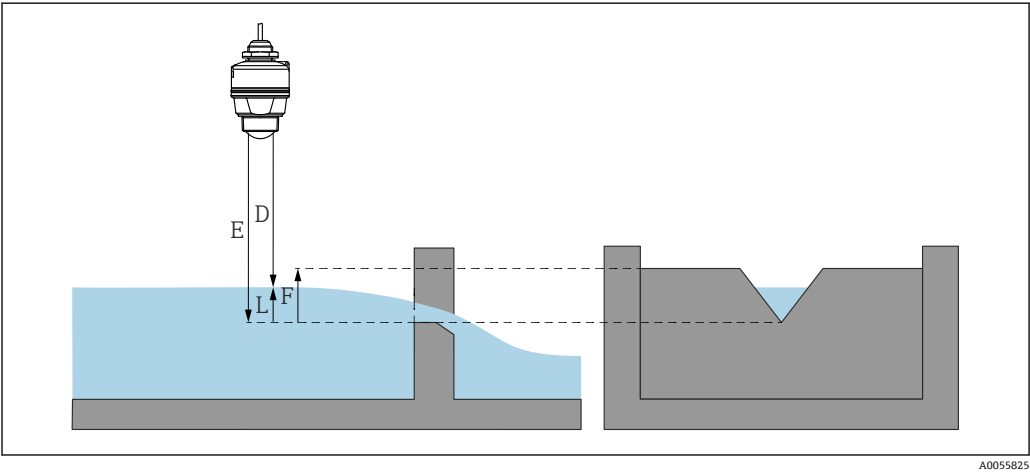
图 24 实例：V 形槽口测量堰
