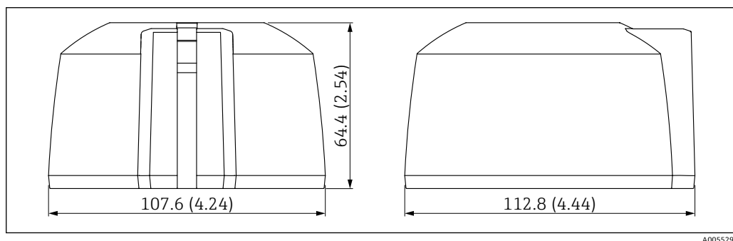
图 26 G1/NPT1 防护罩的外形尺寸（顶部电缆入口）。测量单位 mm (in)
