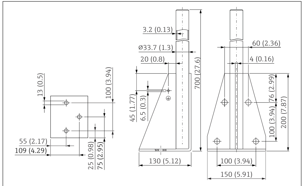
图 45 外形尺寸。测量单位 mm (in)
