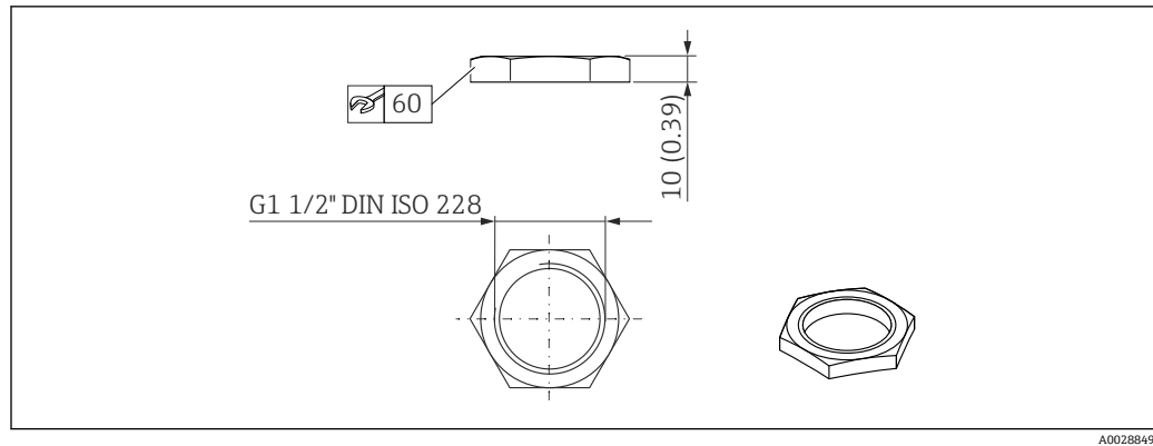
图 28 锁紧螺母的外形尺寸。测量单位 mm (in)
