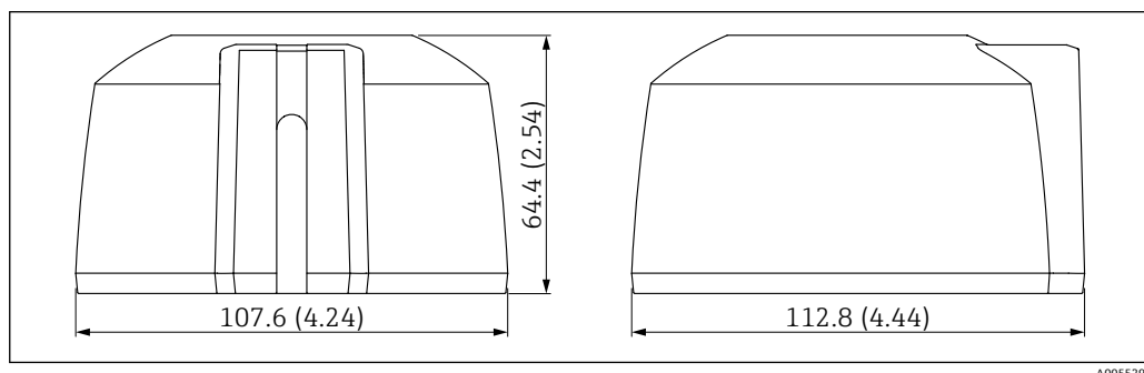
图 27 防护罩的外形尺寸（侧面电缆入口）。测量单位 mm (in)
