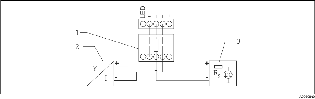
图 15 HART 设备连接安装有 HART 通信电阻的回路显示仪（带背光显示）的功能框图
