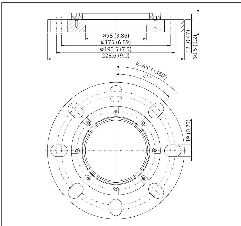
图 51 UNI 4"/DN100/100 松套法兰的外形尺寸示意图。测量单位 mm (in)
