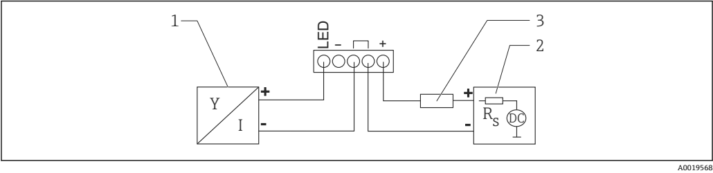
图 13 HART 设备连接 RIA15 回路显示仪（带背光显示）的功能框图
