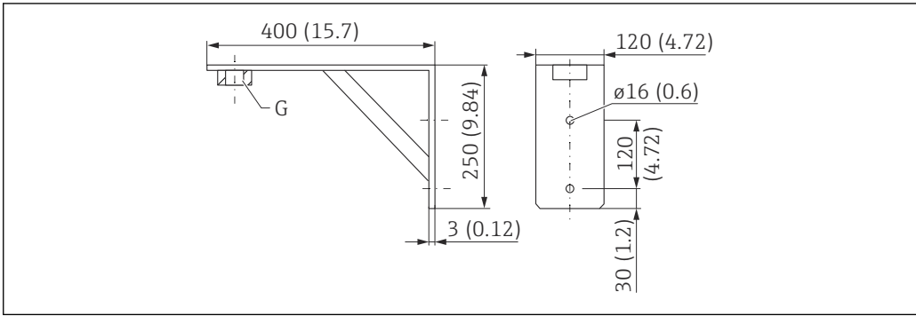
图 38 安装架的外形尺寸示意图。测量单位 mm (in)
