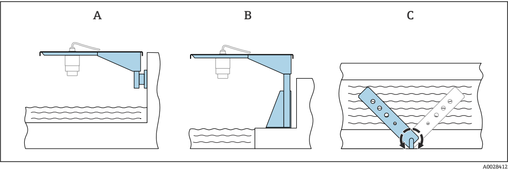
图 8 使用悬臂安装（可旋转） A 使用悬臂和墙装架安装（侧视图） B 使用悬臂和安装架安装（侧视图） C 悬臂可以旋转（例如在水渠正上方定位设备）（俯视图）
