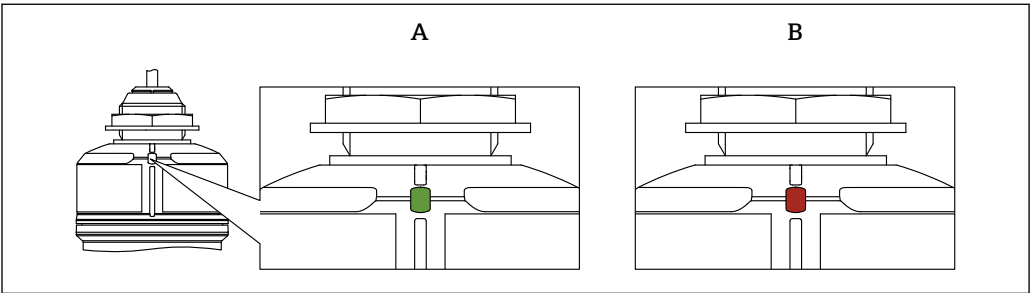
图 25 设备上的 LED 指示灯
