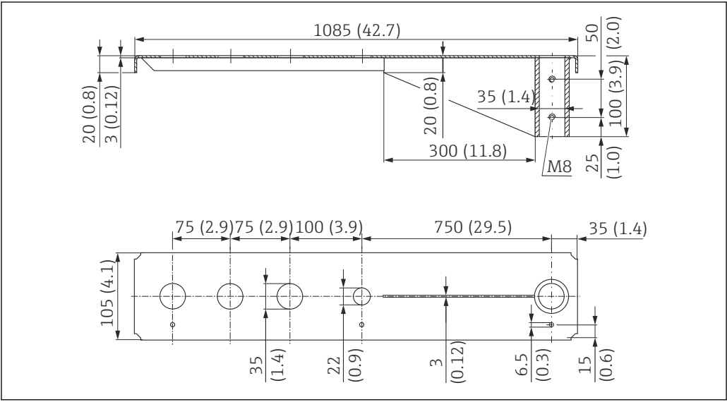
41 1000 mm 旋转悬臂的外形尺寸（安装在传感器电缆入口过程连接上）。测量单位 mm (in)
