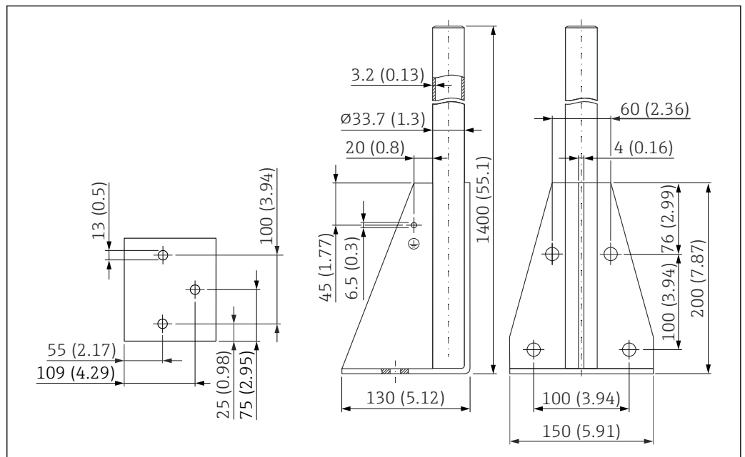
图 46 外形尺寸。测量单位 mm (in)
