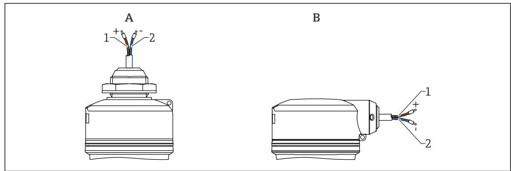
图 10 电缆分配
