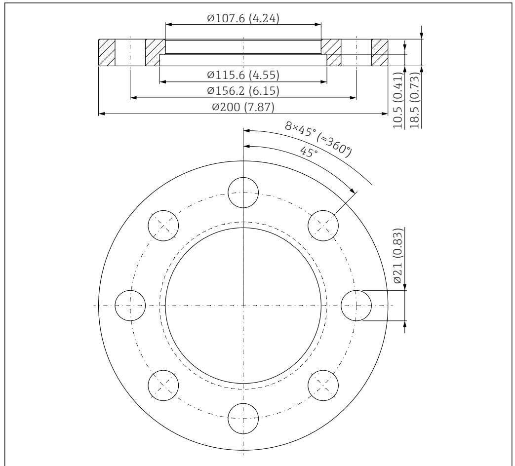
50 UNI 3"/DN80/80 松套法兰的外形尺寸示意图。测量单位 mm (in)
