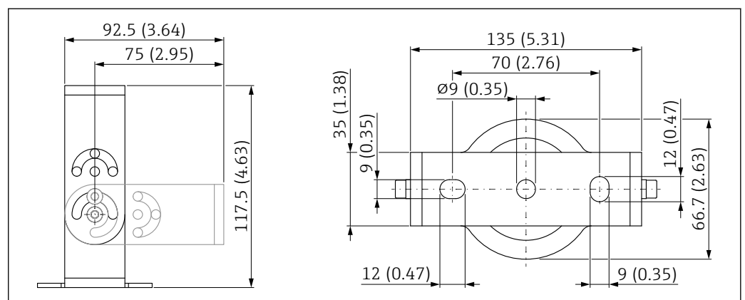
图 35 安装架的外形尺寸示意图。测量单位 mm (in)
