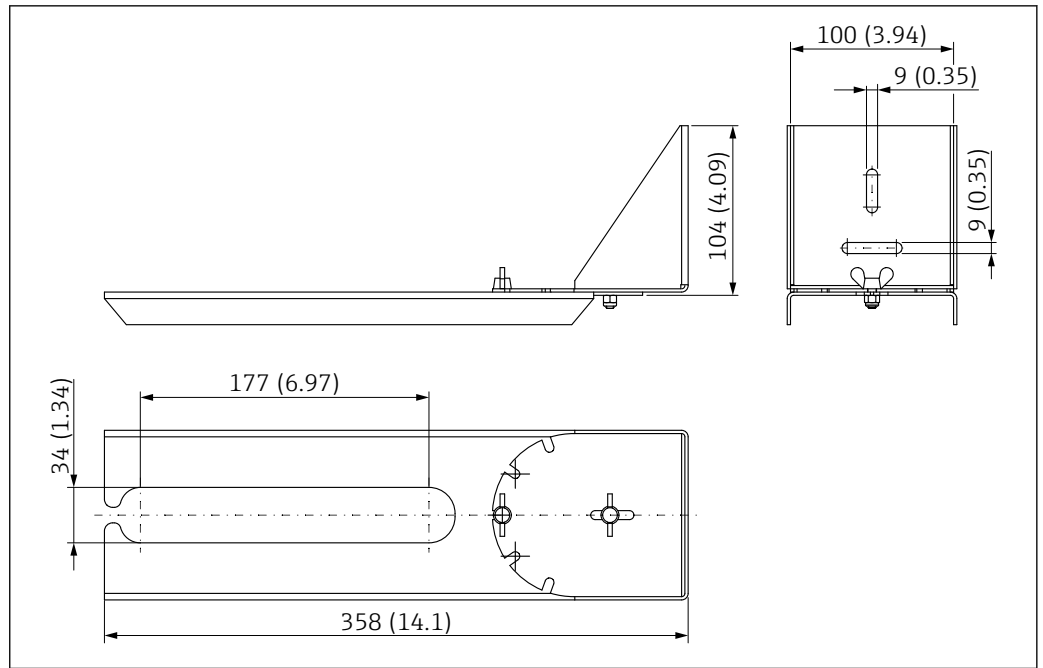
48 旋转安装架的外形尺寸。测量单位 mm (in)
