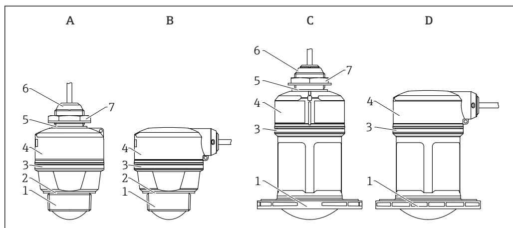
图 1 设备设计
