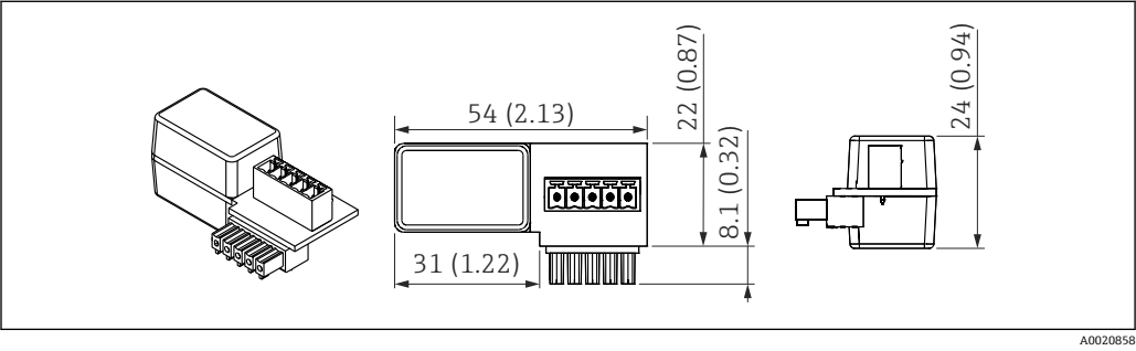
58 HART 通信电阻的外形尺寸。测量单位 mm (in)
