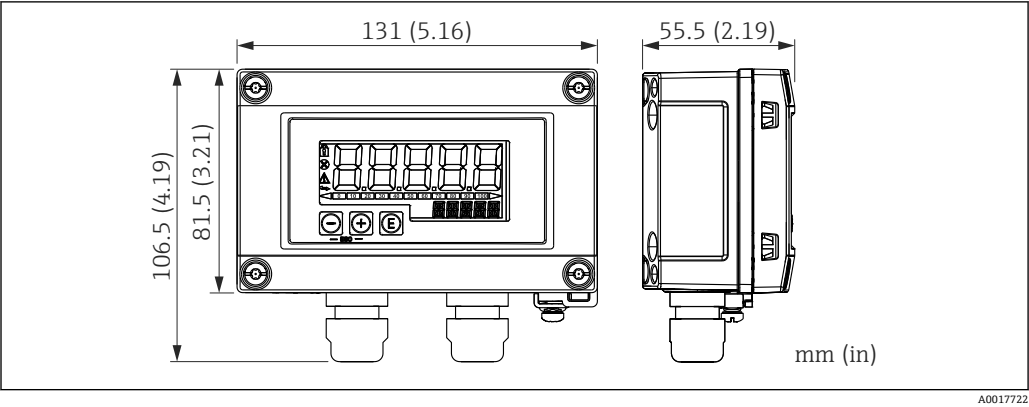
57 RIA15（现场型外壳）的外形尺寸。测量单位 mm (in)
