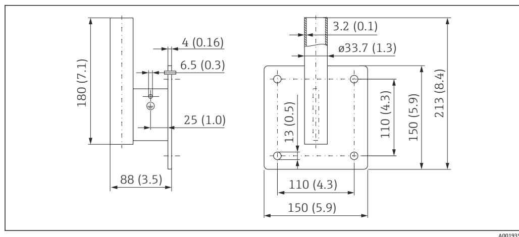
图 47 墙装架的外形尺寸。测量单位 mm (in)
