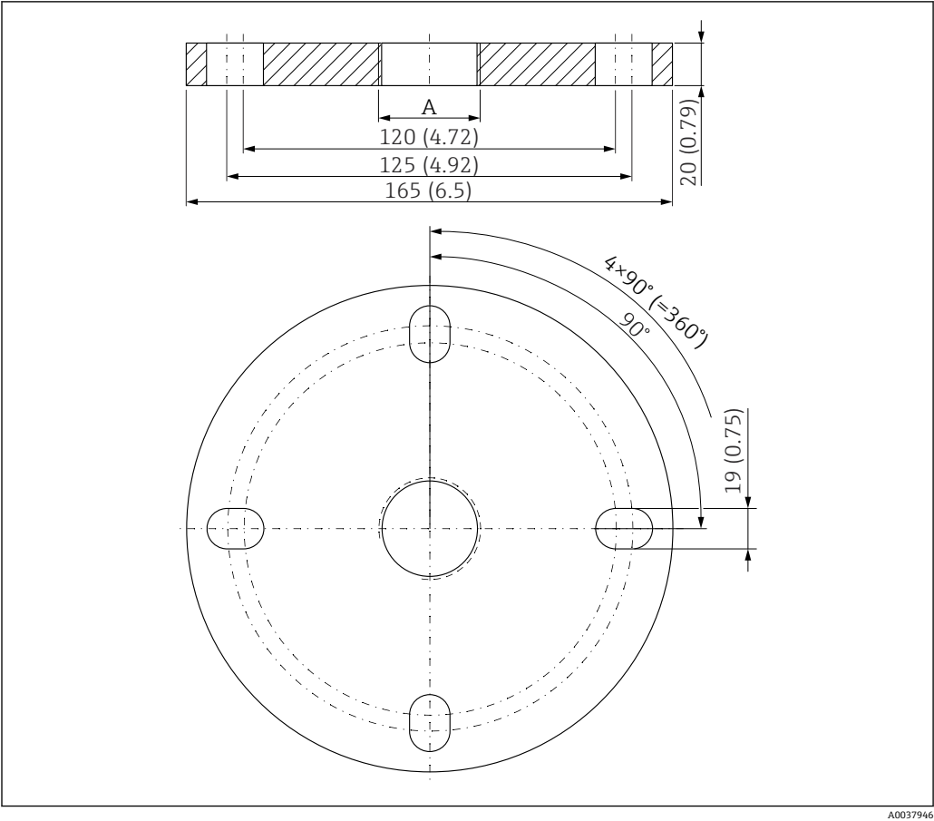
53 UNI 2"/DN50/50 法兰的外形尺寸示意图。测量单位 mm (in)
