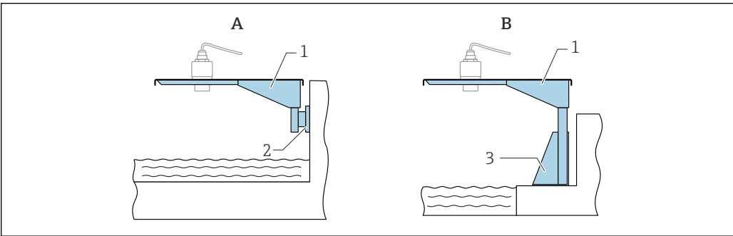
图 42 传感器天线端过程连接的安装方式
