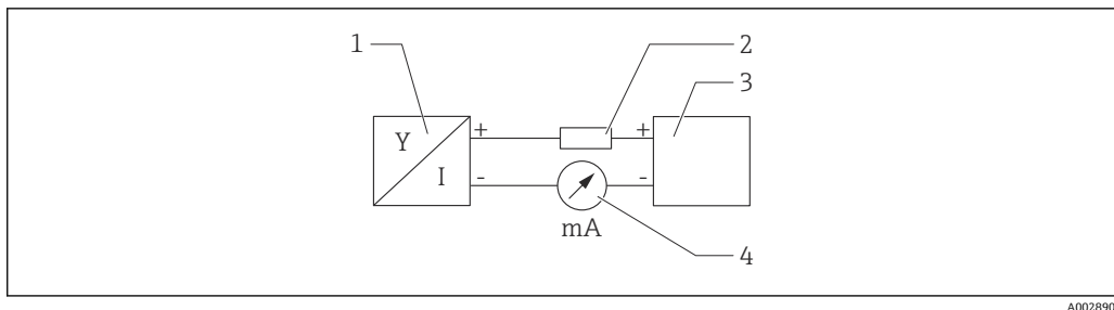
图 11 HART 连接功能框图
