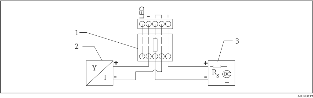
图 14 HART 设备连接安装有 HART 通信电阻的回路显示仪（无背光显示）的功能框图
