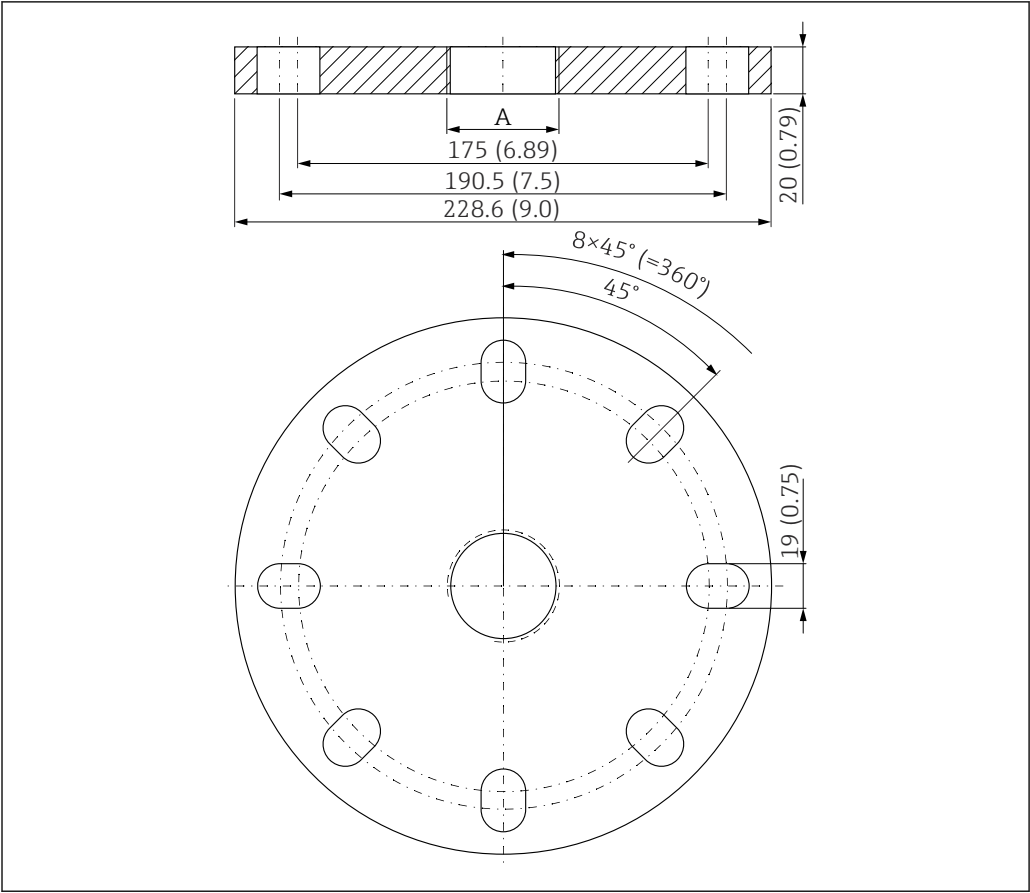
55 UNI 4"/DN100/100 法兰的外形尺寸示意图。测量单位 mm (in) A 传感器连接（产品选型表中的“天线端过程连接”或“电缆入口过程连接”）
