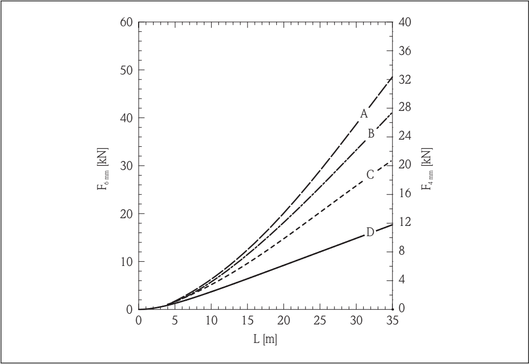
图 5 张力负载与物位 (L) 关系曲线图; 6 mm (0.24 in)和 4 mm (0.16 in)缆式探头, 石英砂料仓; 光滑金属壁
