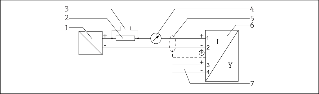
17 接线图：两线制；4...20 mA HART，开关量输出
