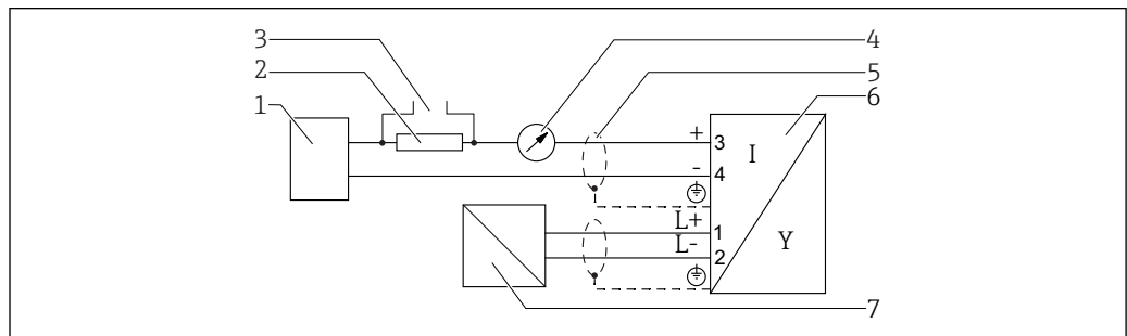
图 21 接线端子分配：四线制；4...20 mA HART (10.4 ... 48 V DC )
