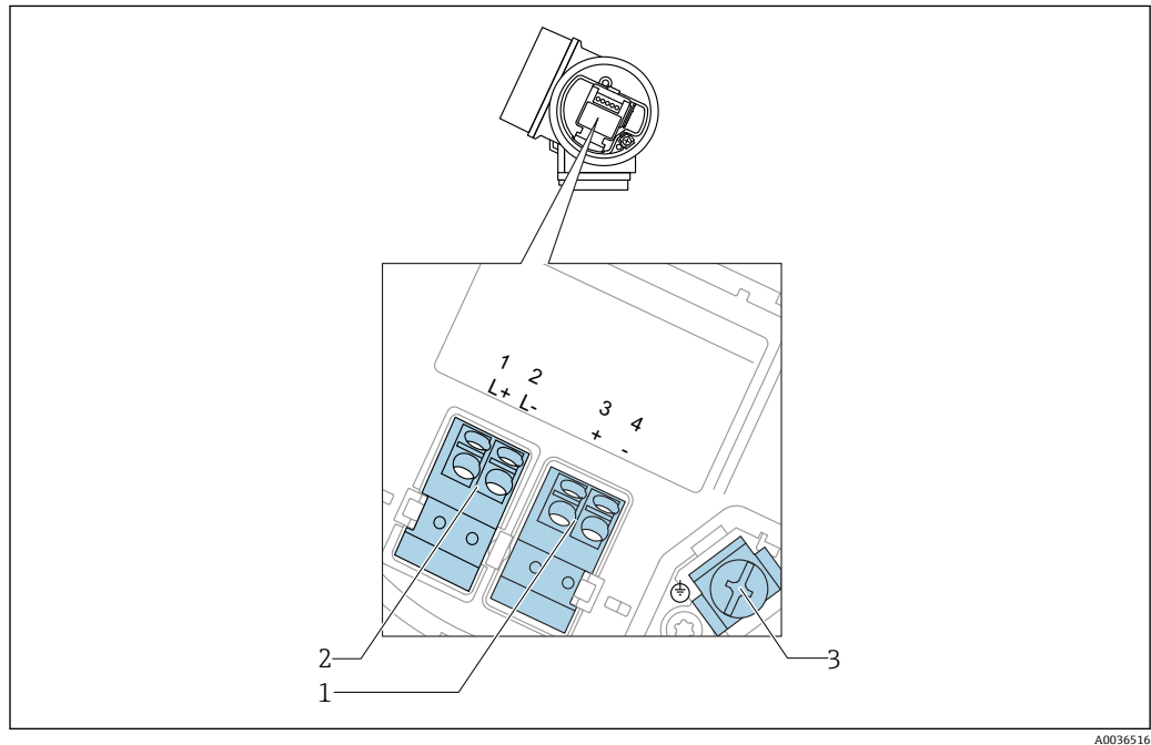
图 20 接线端子分配：四线制；4...20 mA HART (10.4 ... 48 V DC )
