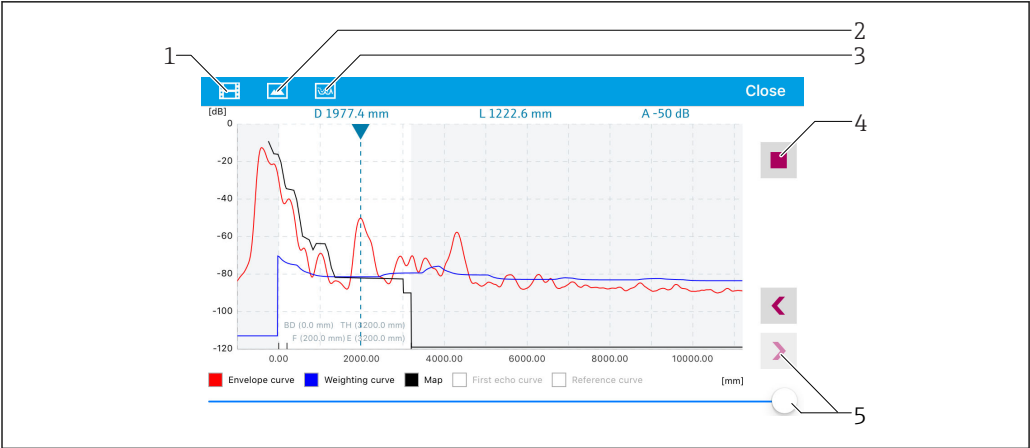
41 在 SmartBlue 中显示包络线; IoS 视图
