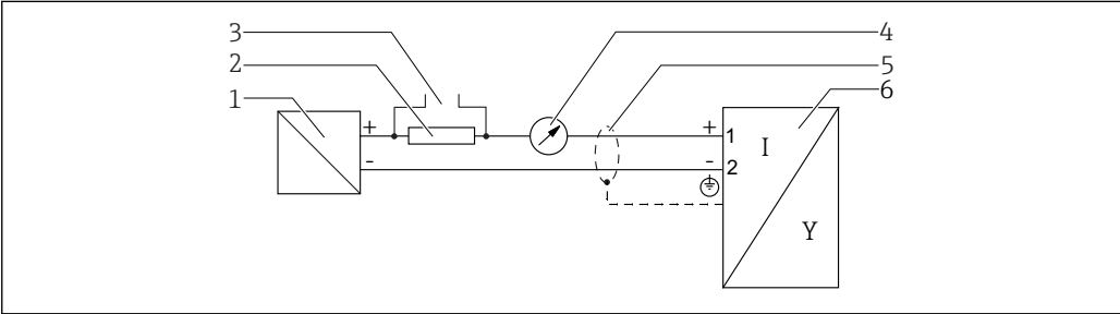
15 接线图: 两线制; 4...20 mA HART
