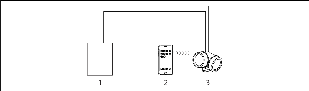
图 30 通过 SmartBlue (app) 操作
