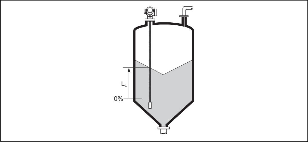
52 料位测量时的料位
