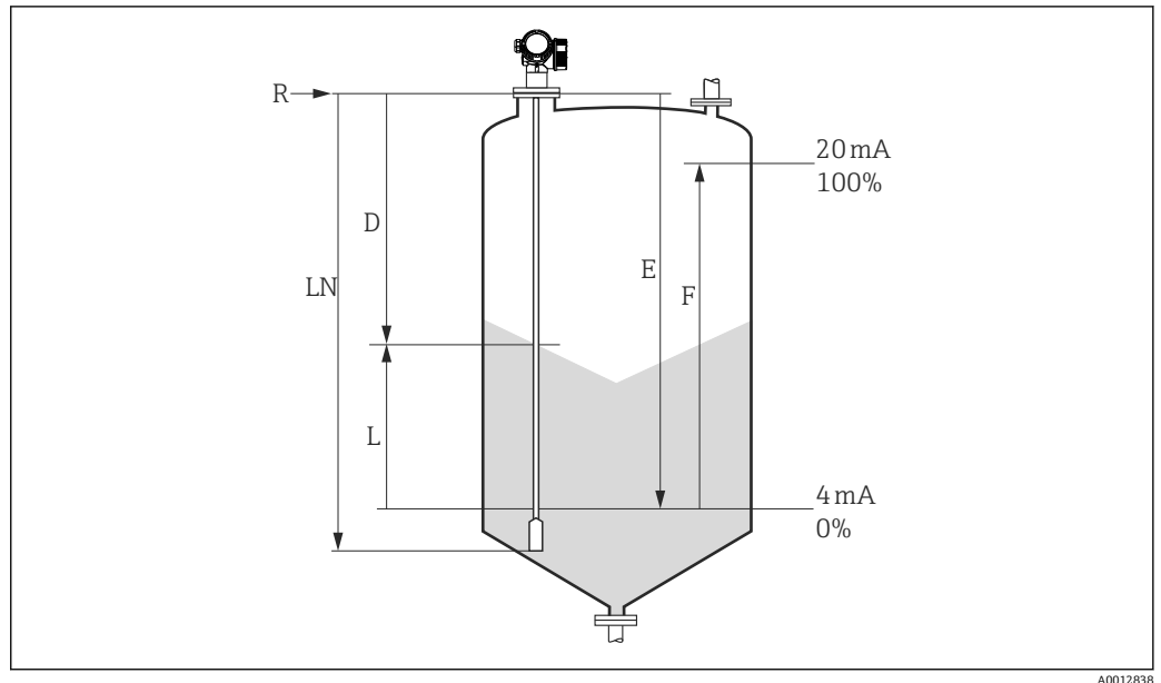
图 43 料位测量时的设置参数
