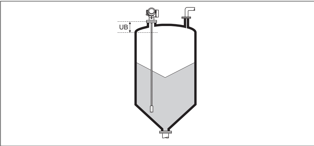
☰ 54 料位测量的盲区距离 (UB)
