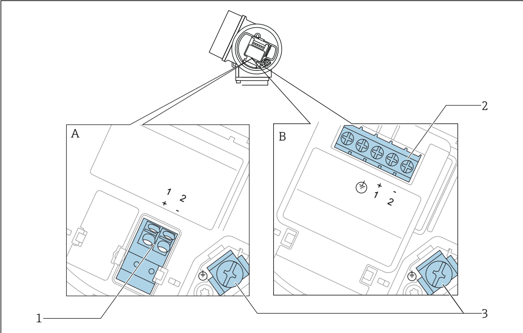
14 接线端子分配: 两线制; 4...20 mA HART
