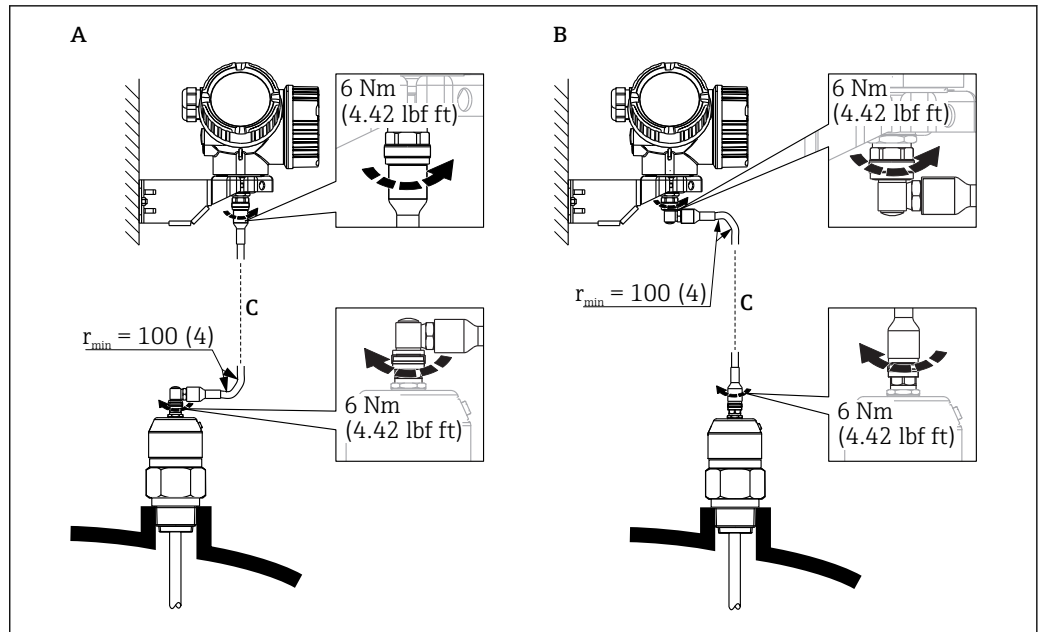
图 13 连接电缆。可选下列方式：
