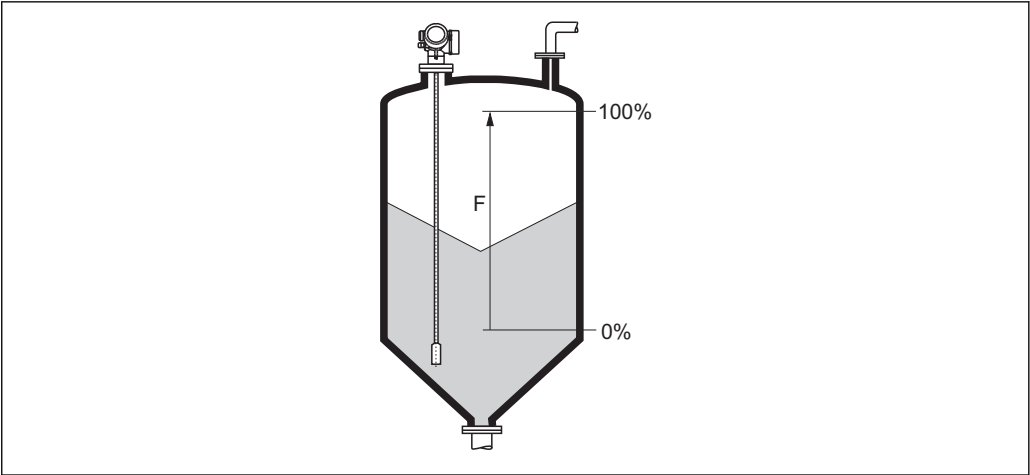
51 料位测量时的满标 (F)
