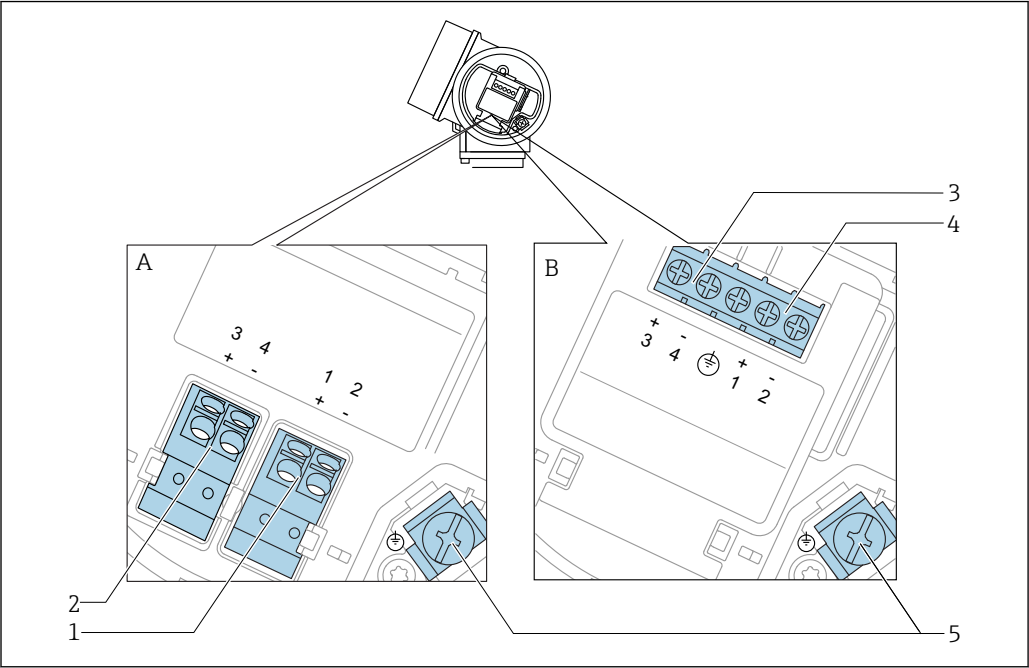
16 接线端子分配：两线制；4...20 mA HART，开关量输出
