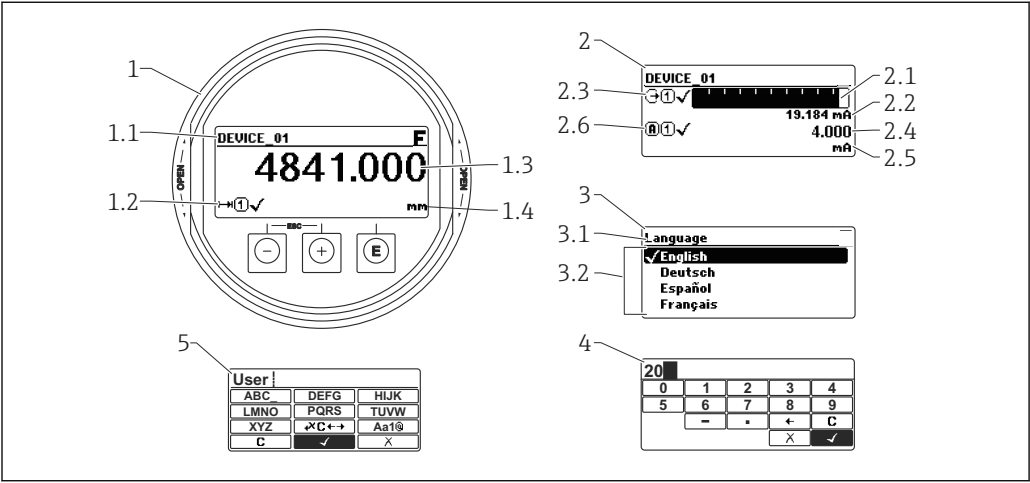
图 33 进行现场操作时显示与操作单元的显示界面
