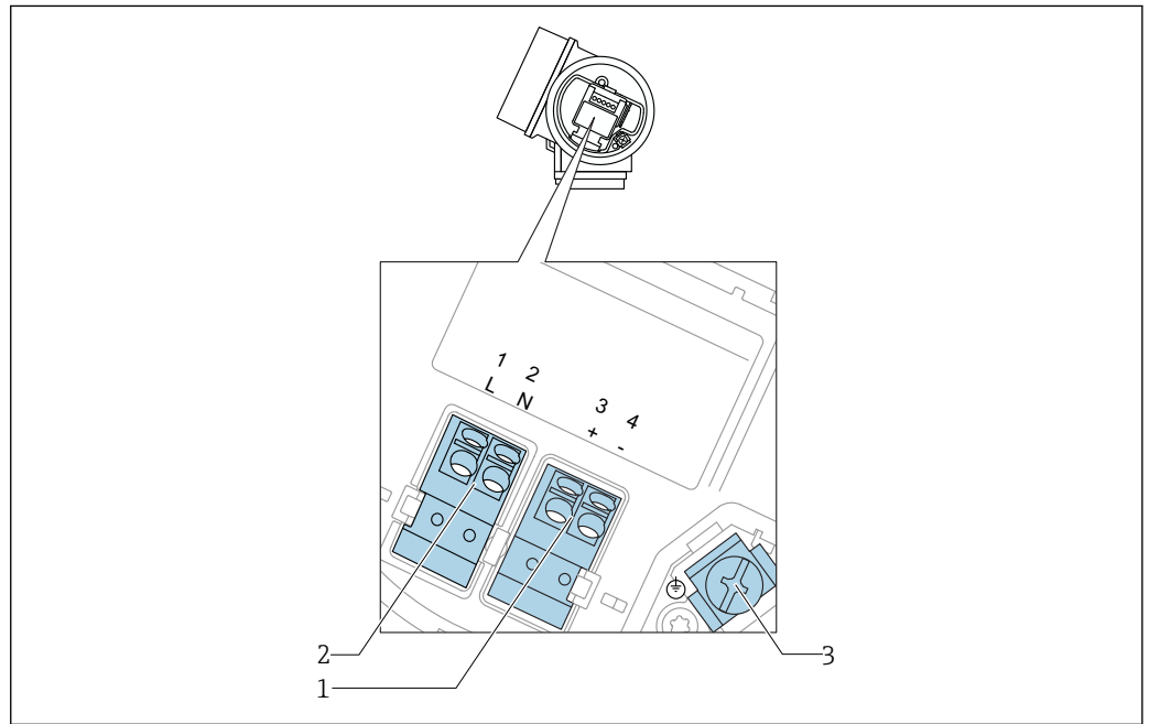
图 22 接线端子分配: 四线制; 4...20 mA HART (90 ... 253 V AC )
