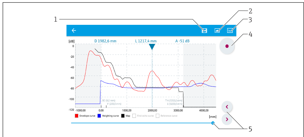
40 在 SmartBlue 中显示包络线； Android 视图
