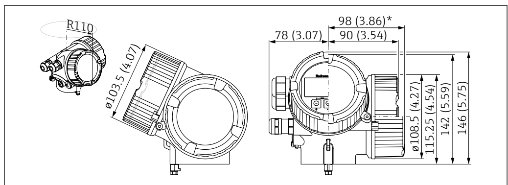
33 GT18 外壳 (316 L)。测量单位 mm (in)
