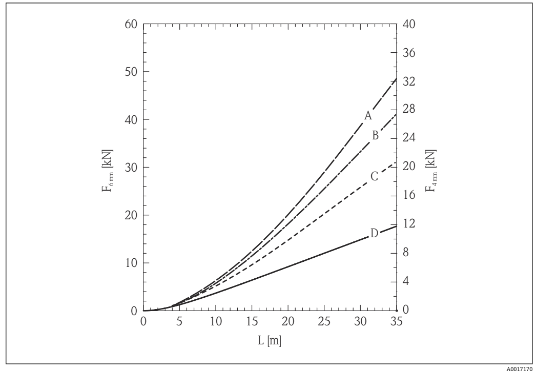
图 26 张力负载与物位 (L) 关系曲线图; 6 mm (0.24 in) 和 4 mm (0.16 in) 缆式探头, 石英砂料仓; 光滑金属仓壁
