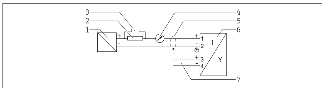
图 9 功能框图: 4 ... 20 mA HART, 开关量输出
