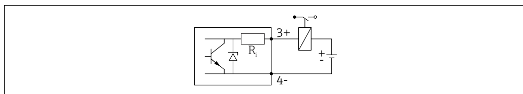
10 继电器的连接示例
