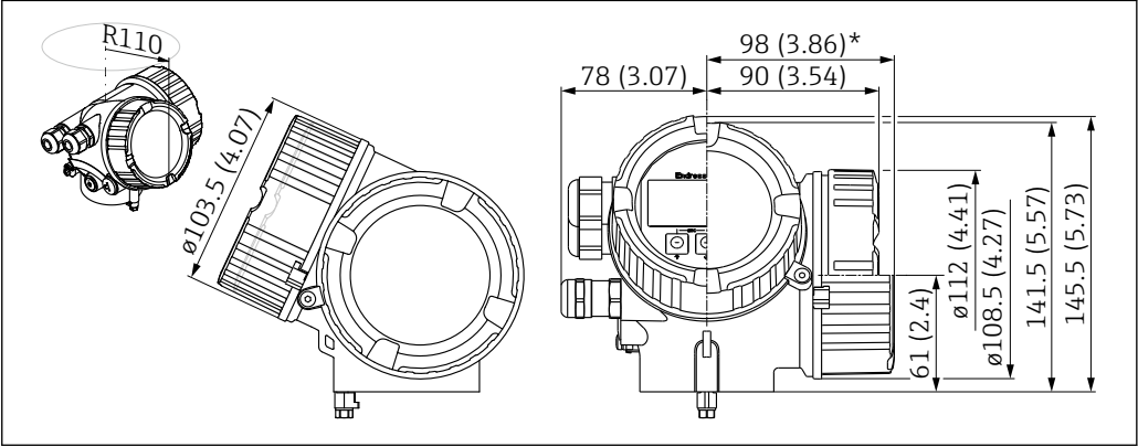
31 GT20 外壳（铝，带涂层）。测量单位 mm (in)
