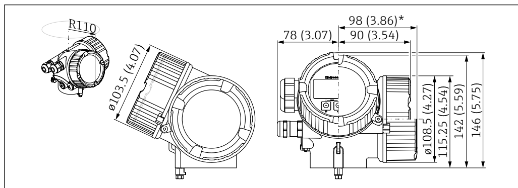
29 GT18 外壳 (316 L)。测量单位 mm (in)
