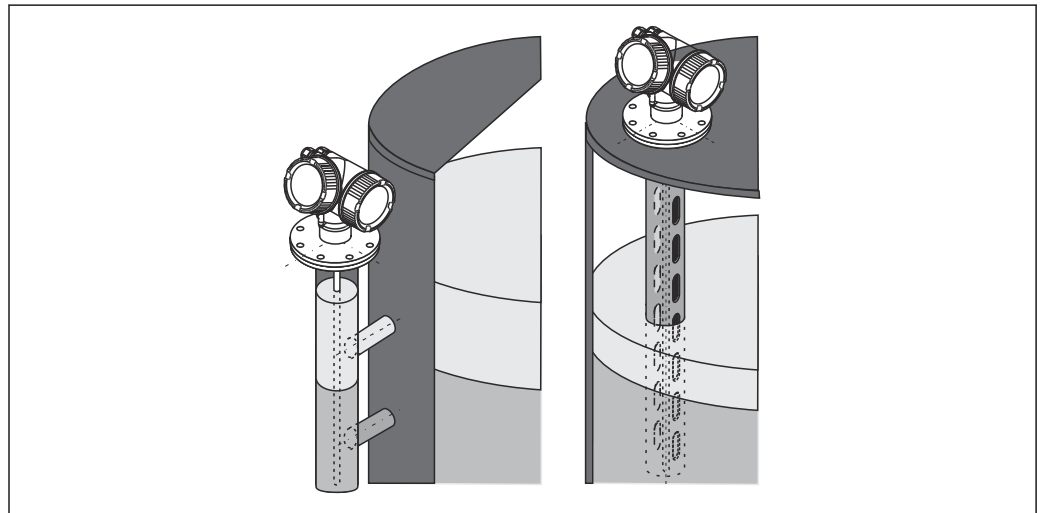
图 27 Levelflex FMP55 的安装位置
