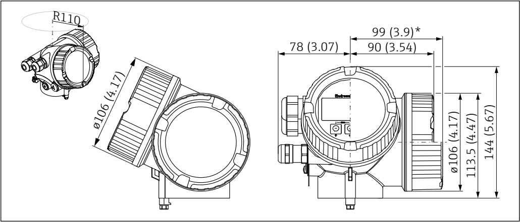
30 GT19 外壳（塑料 PBT）。测量单位 mm (in)
