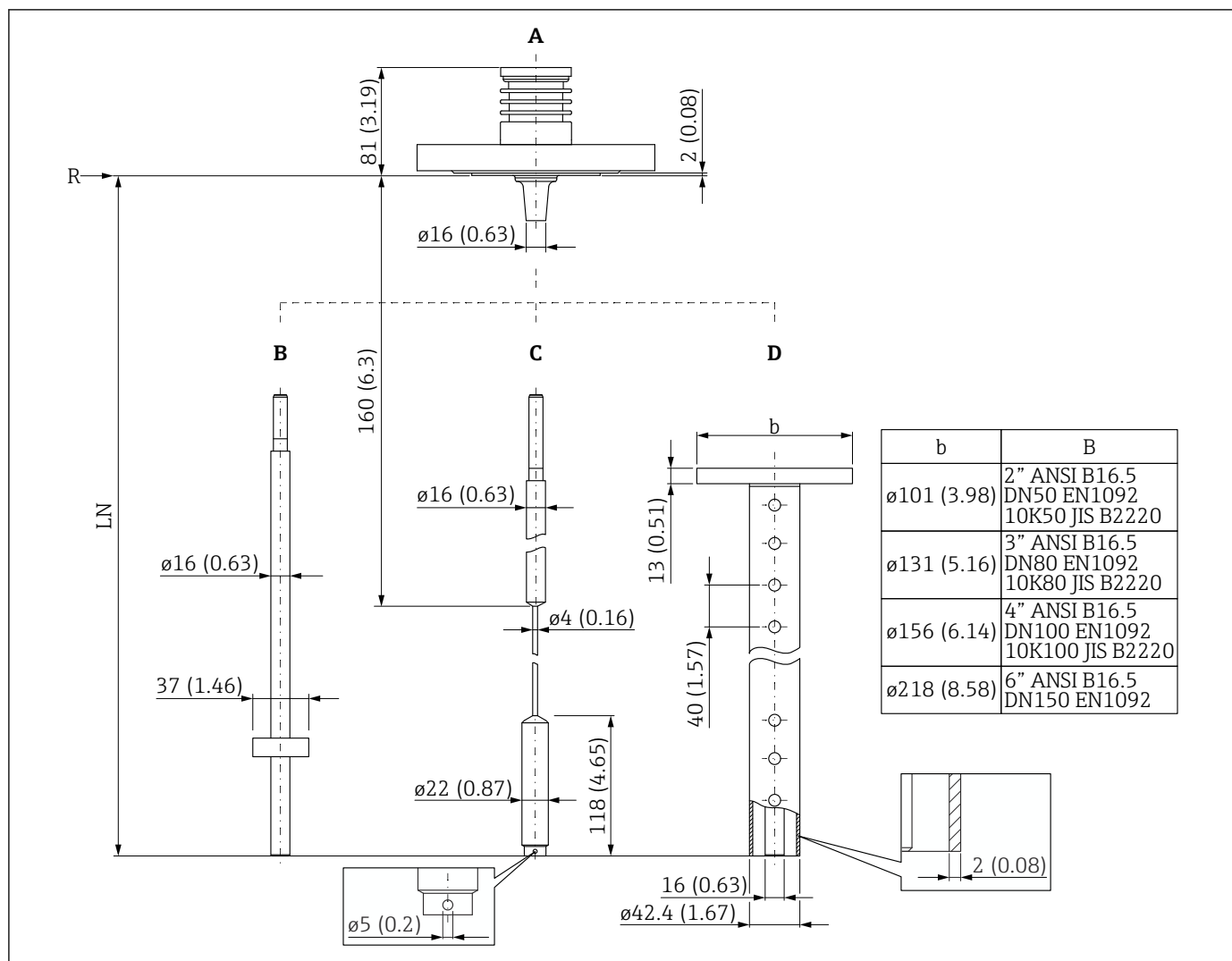
34 FMP55: 过程连接和探头。测量单位 mm (in)
