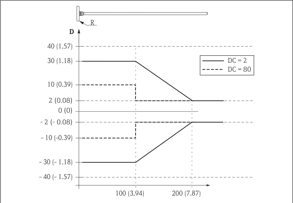
26 探头顶部出现的测量误差; 单位: mm (in)
