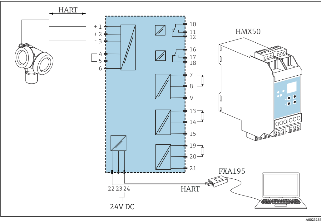
图 21 HART 回路转换器 HMX50 的接线图（图例：无源两线制设备，连接电流输出，用作电源）
