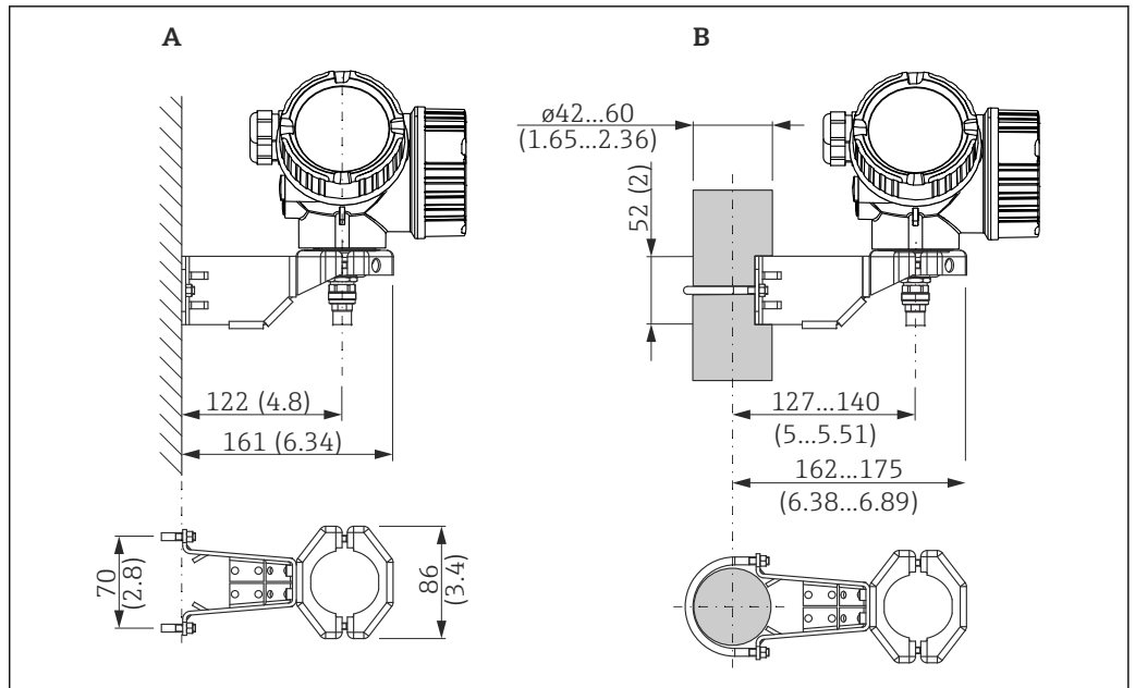
50 电子腔外壳安装架; 单位: mm (in)
