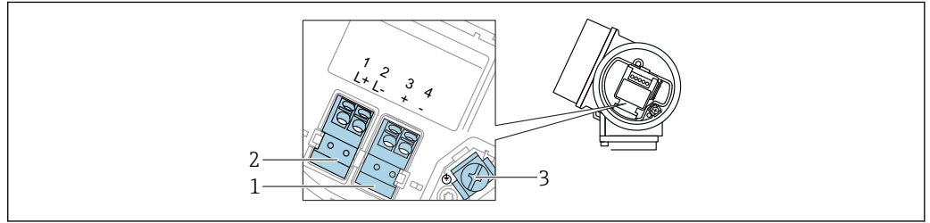
15 接线端子分配，四线制：4 ... 20 mA HART (10.4 ... 48 V DC )
