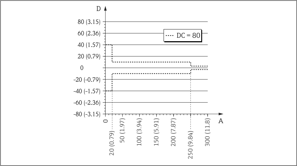
25 缆式探头底部附近的测量误差
