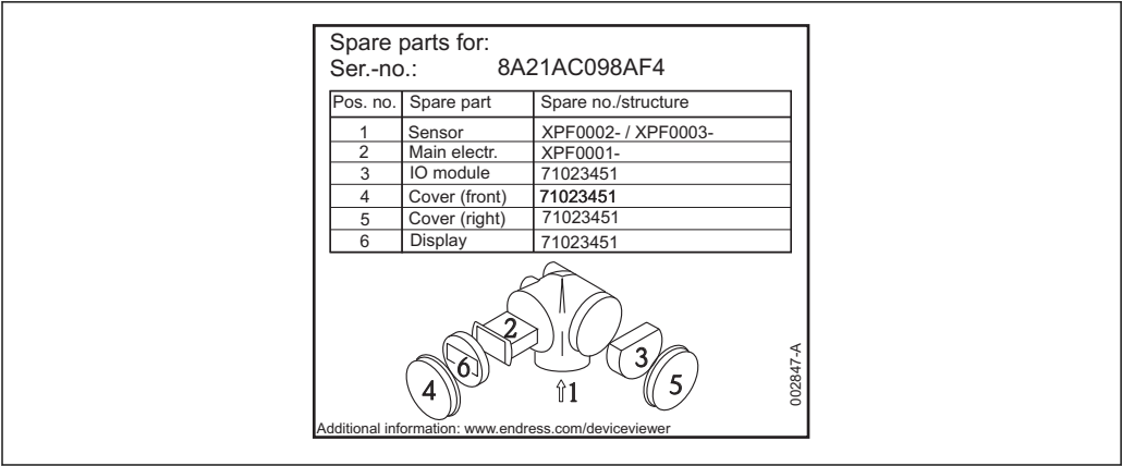
图 26 接线腔外壳内的备件铭牌示意图
