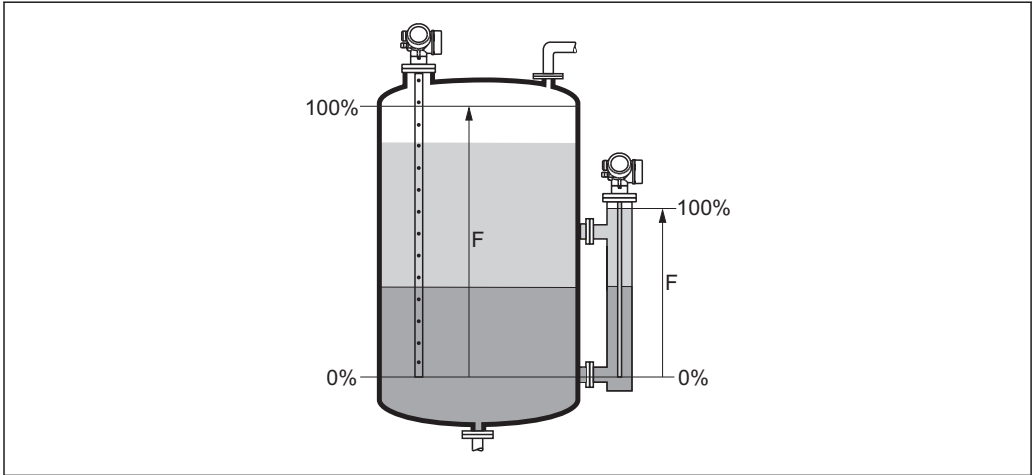
30 界面测量时的满标 (F)
