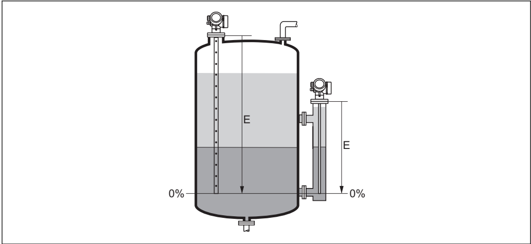
29 界面测量时的空标 (E)
