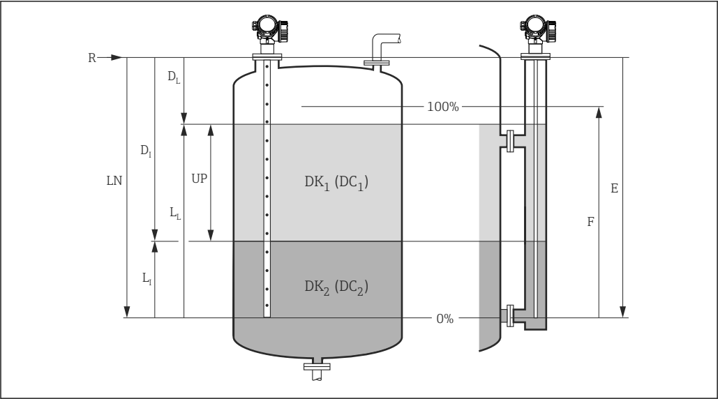
图 23 界面测量时的设置参数
