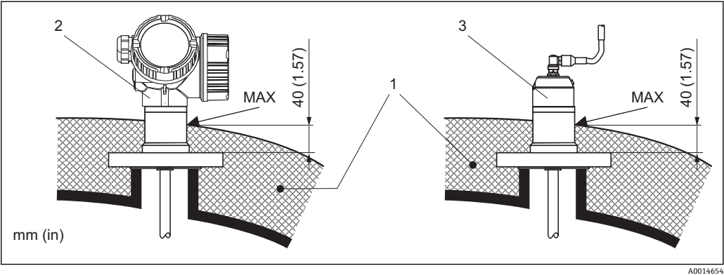
5 带法兰过程连接的 FMP55
