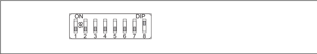
图 21 软件地址设定实例：开关 8 拨至“ON (开)”位置；通过操作菜单设置地址(设置→设备地址)
