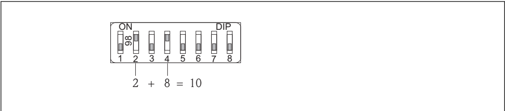
图 20 硬件地址设定实例：开关 8 拨至“OFF (关)”位置；通过开关 1...7 设置地址。
