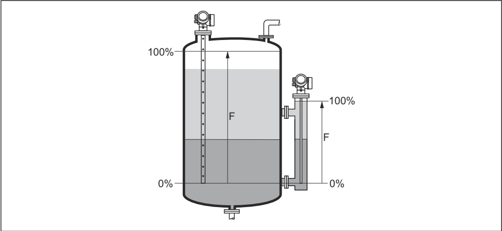
42 界面测量时的满标 (F)
