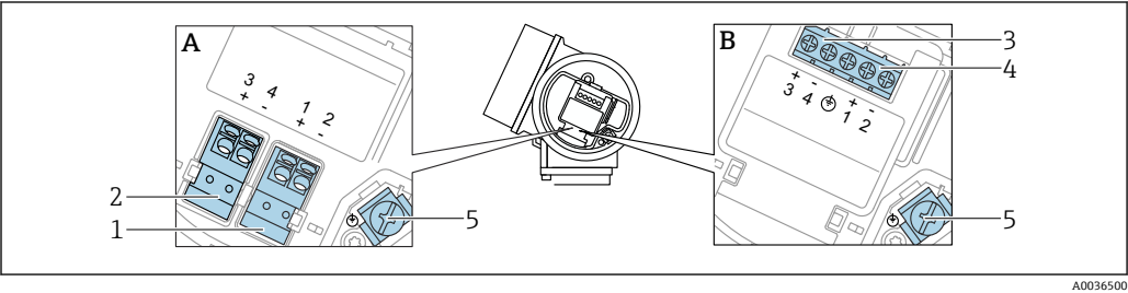
图 12 接线端子分配，两线制：4 ... 20 mA HART，4 ... 20 mA
