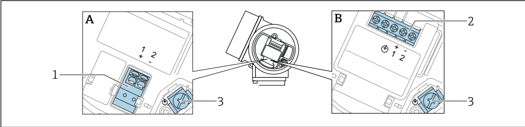
图 8 接线端子分配，两线制：4 ... 20 mA HART
