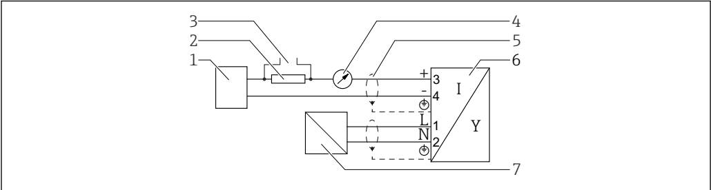
图 17 接线图：四线制：4 ... 20 mA HART (90 ... 253 V AC )
