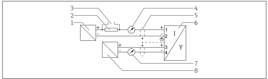
图 13 接线图：两线制：4 ... 20 mA HART, 4 ... 20 mA
