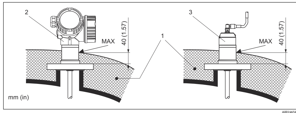
图 5 法兰过程连接
