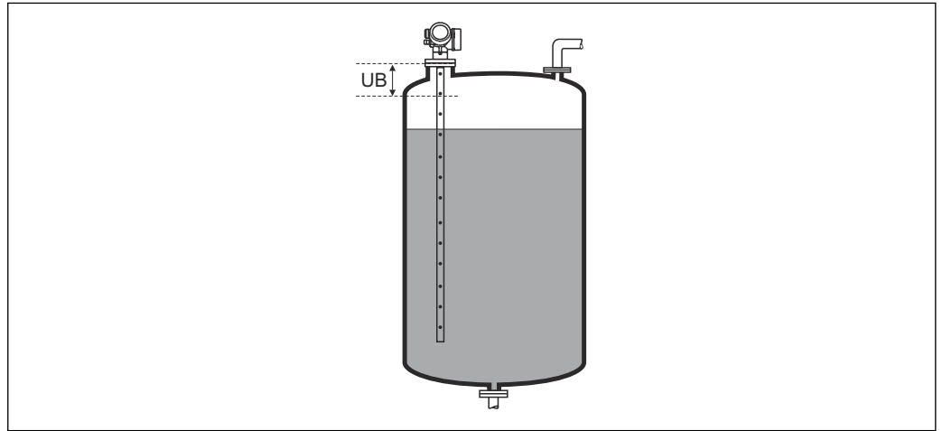
图 47 液位测量的盲区距离 (UB)
