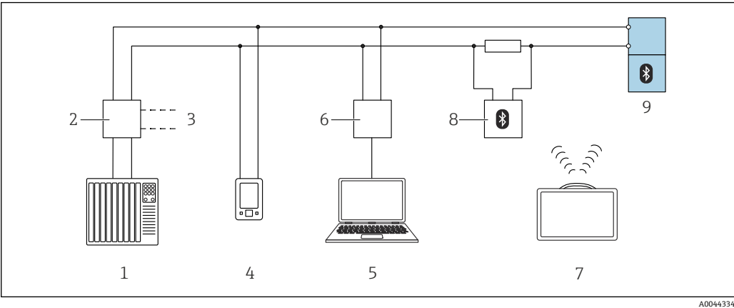
图 28 通过 HART 通信实现远程操作
