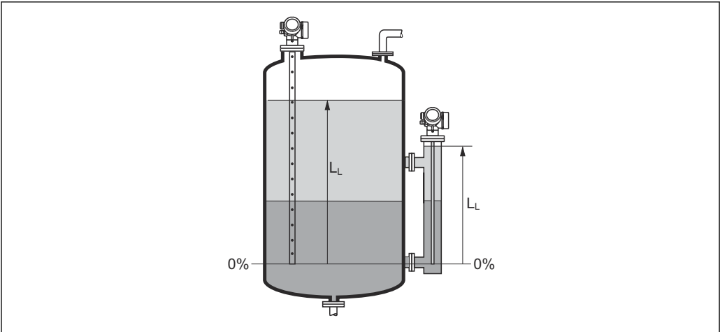
43 界面测量时的液位
