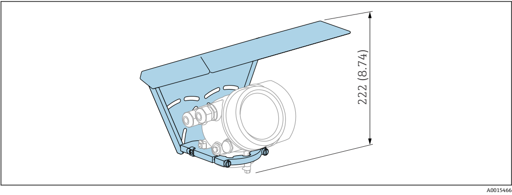
图 38 高度。测量单位 mm (in)
