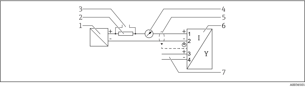
图 11 接线图：两线制：4 ... 20 mA HART，开关量输出
