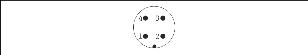
21 M12 插头的针脚分配
