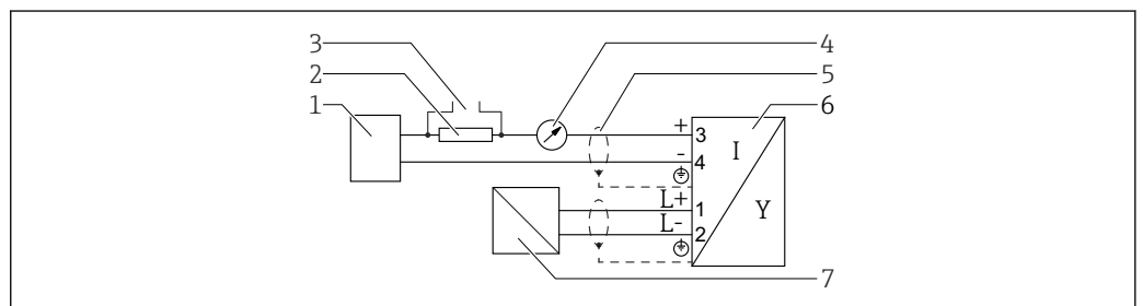
图 15 接线图：四线制：4 ... 20 mA HART (10.4 ... 48 V DC )
