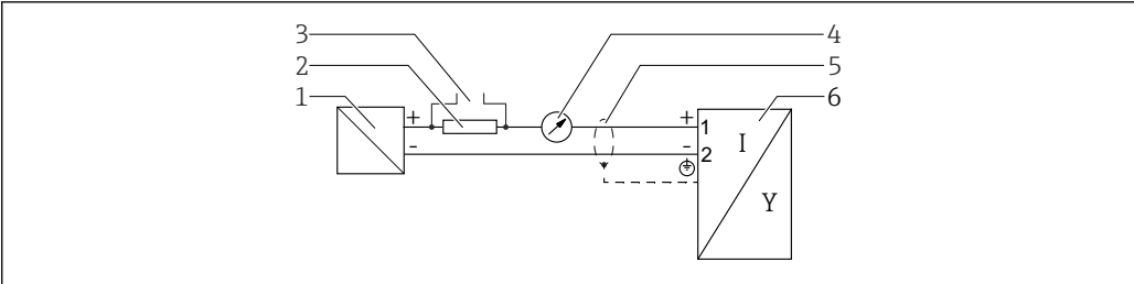
图 9 接线图：两线制：4 ... 20 mA HART
