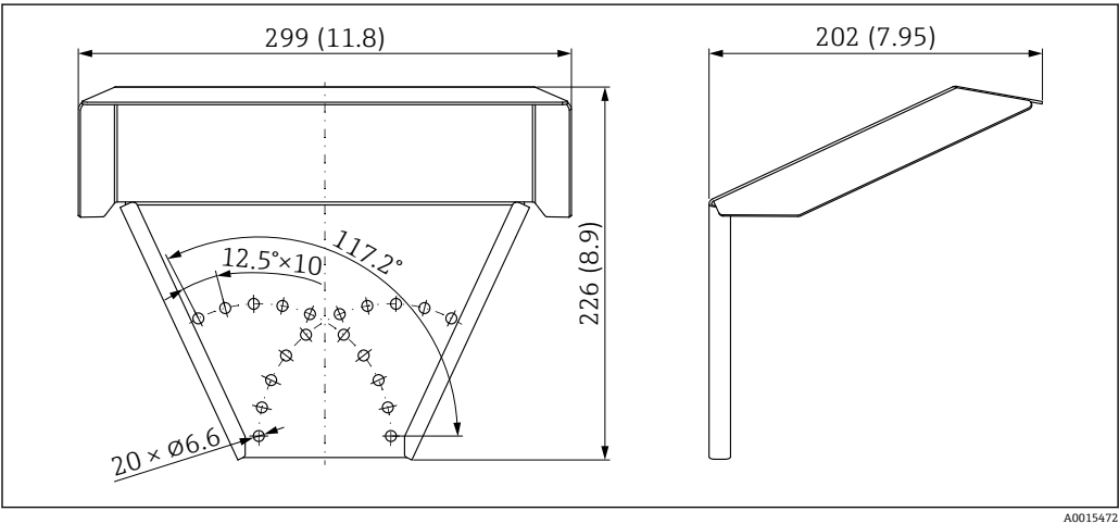
图 39 外形尺寸。测量单位 mm (in)
