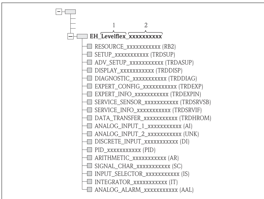
图 18 连接建立后的组态设置程序的典型显示界面
