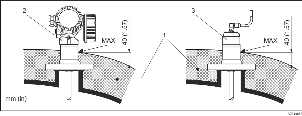
图 4 法兰过程连接
