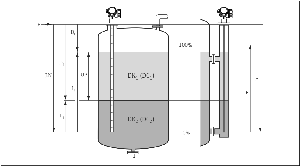
图 24 界面测量设置参数
