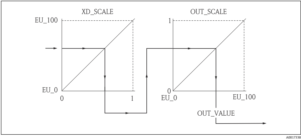
图 23 按比例转换 AI 块中的测量值
