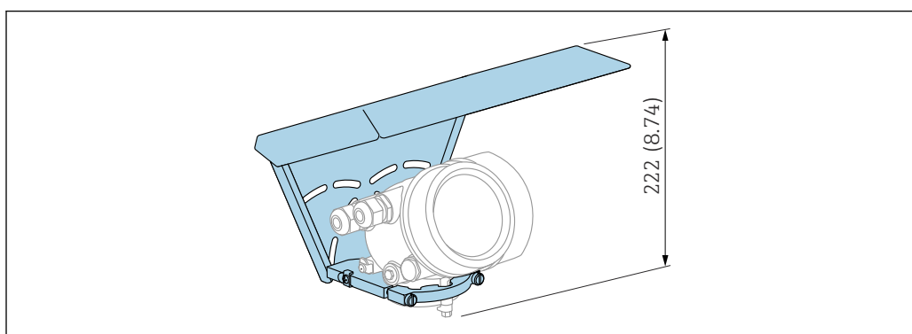
图 30 高度。测量单位 mm (in)
