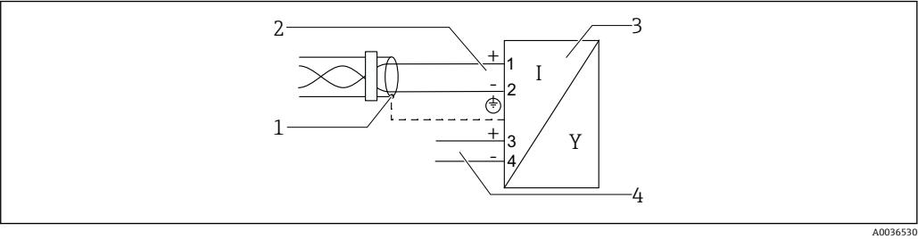
图 9 功能框图：PROFIBUS PA / FOUNDATION Fieldbus
