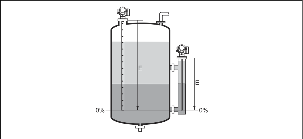
51 界面测量时的空标 (E)
