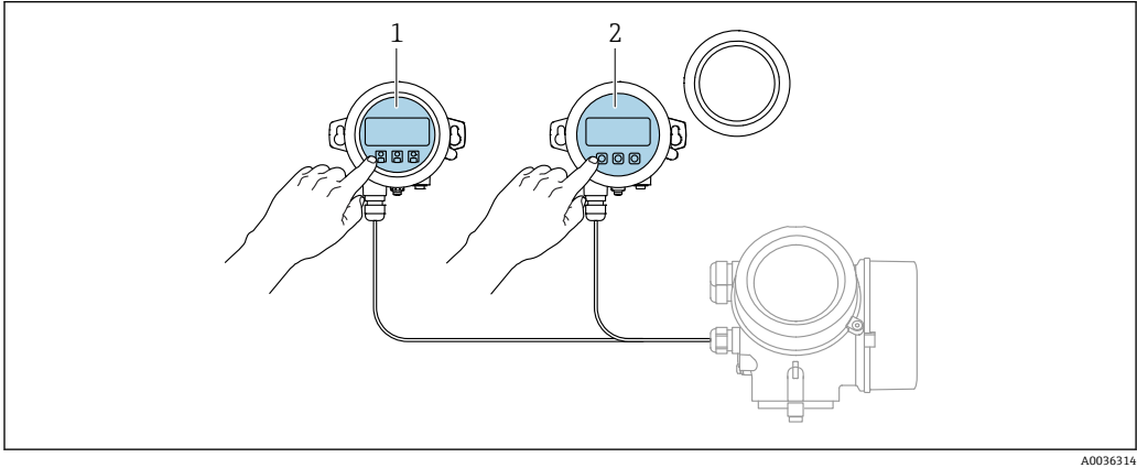
图 29 FHX50 的操作选项
