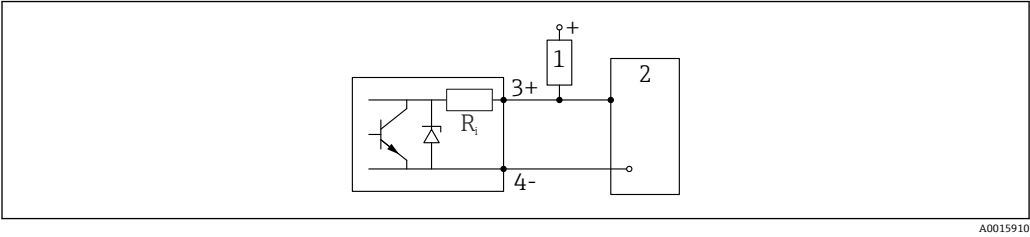
图 17 数字量输入的连接示例
