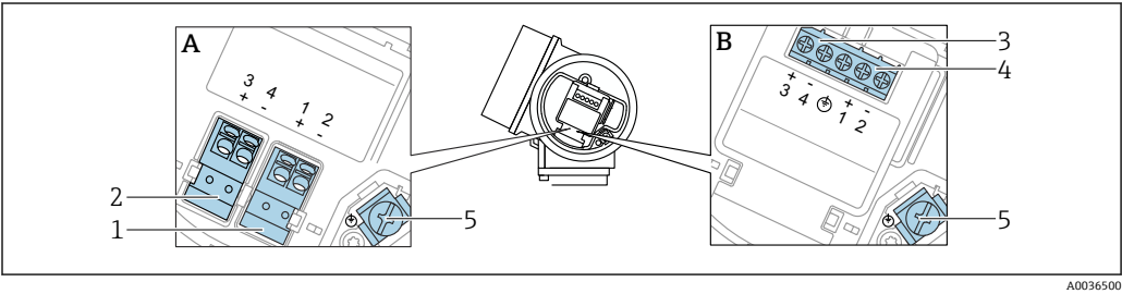
图 18 接线端子分配，两线制：4 ... 20 mA HART，4 ... 20 mA
