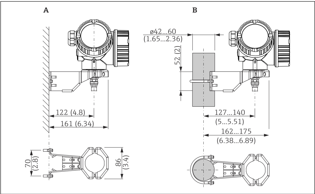
图 46 电子腔外壳安装架; 单位: mm (in)
