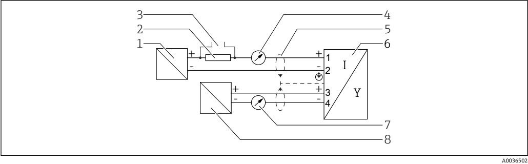
图 19 功能框图：4 ... 20 mA HART + 4 ... 20 mA 模拟量
