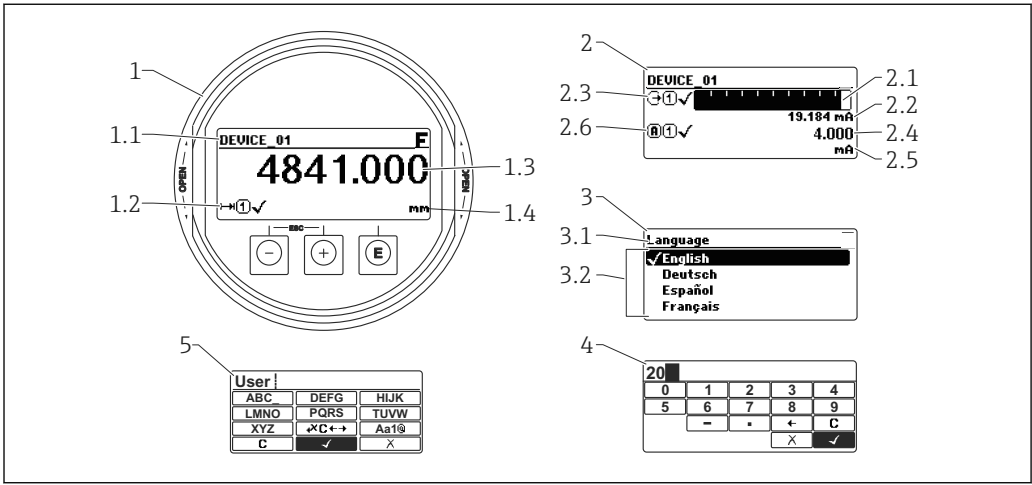
图 17 进行现场操作时显示与操作单元的显示界面
