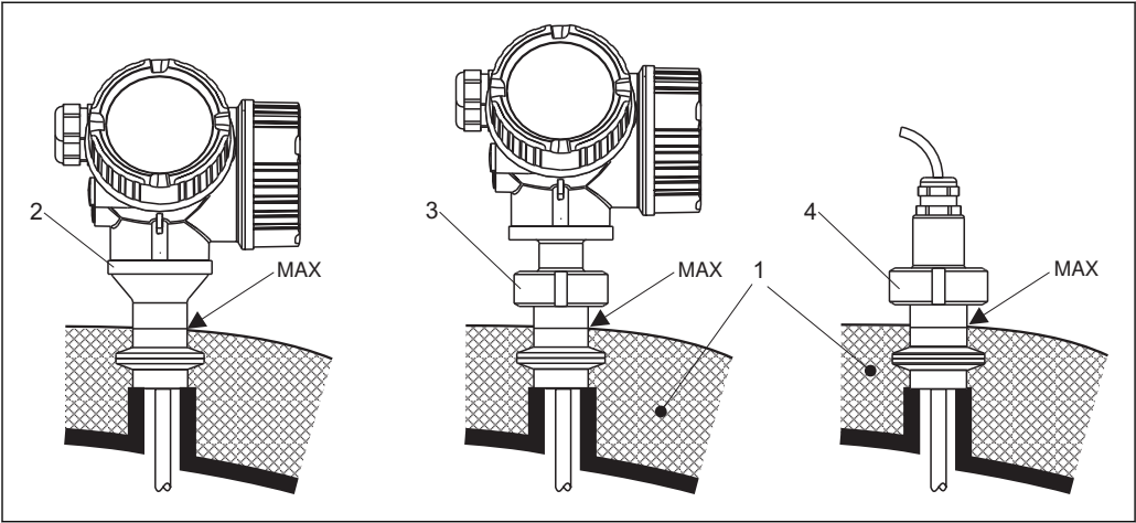
图 5 带卫生型过程连接的 FMP53
