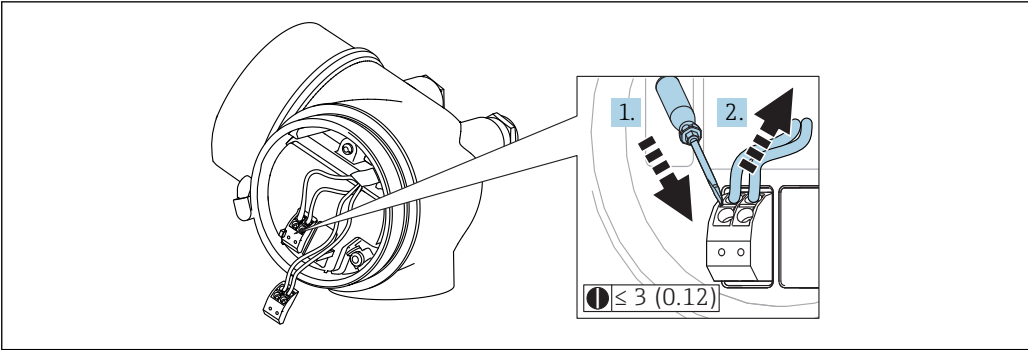
图 13 单位: mm (in)
