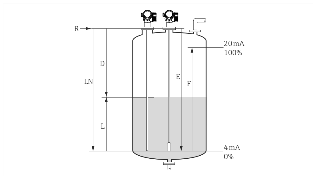
图 22 液位测量时的设置参数
