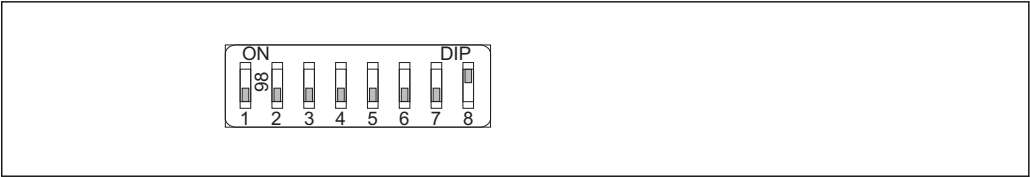
图 20 软件地址设定实例：开关 8 拨至“ON (开)”位置；通过操作菜单设置地址(设置→设备地址)
