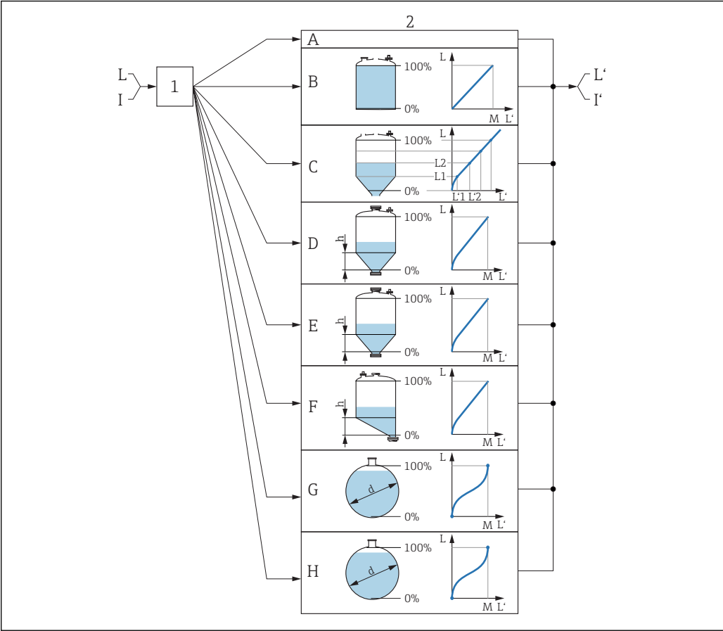
33 线性化：将物位和（相关）界面高度转换成体积或重量；转换取决于容器形状。
