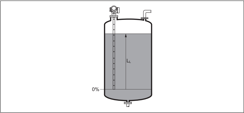
30 液位测量时的液位
