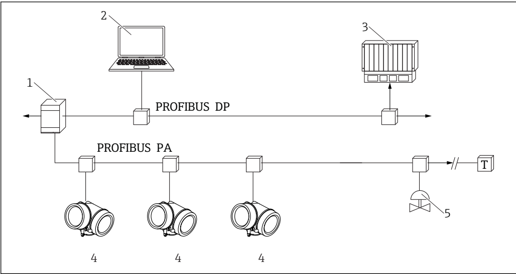
图 15 通过 PROFIBUS PA 网络进行远程操作
