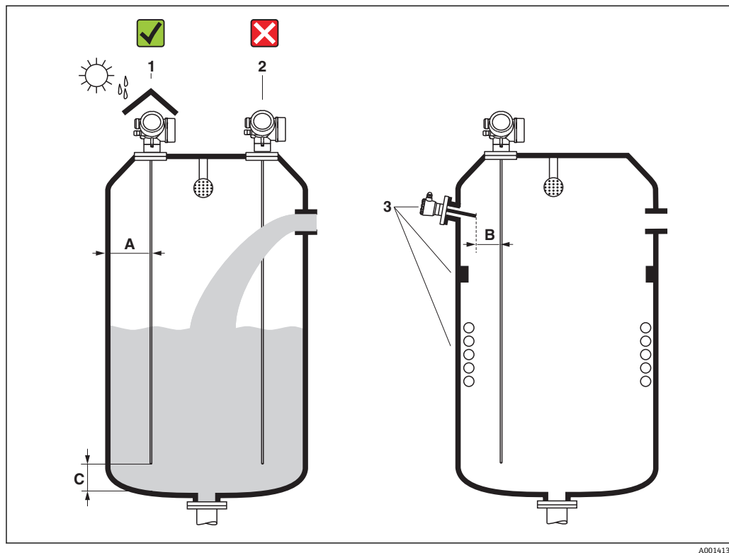
图 4 Levelflex 的安装要求
