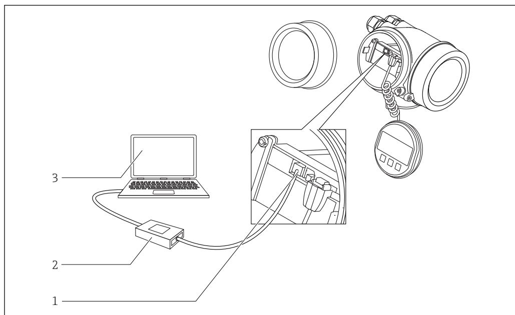
图 16 DeviceCare/FieldCare, 使用服务接口 (CDI)
