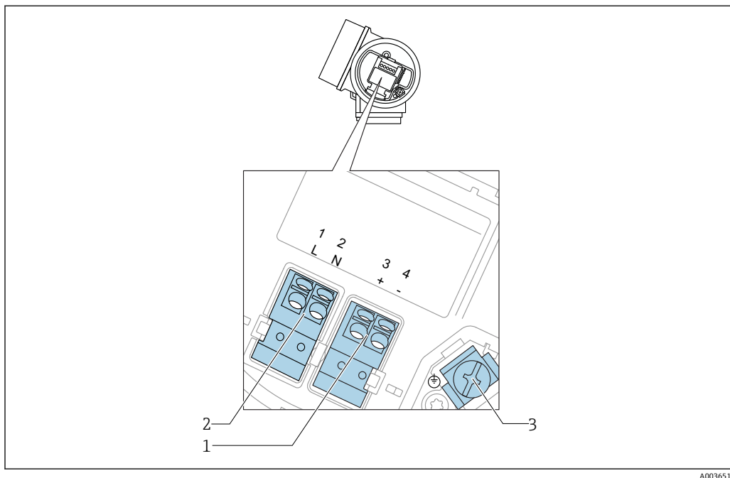
图 7 接线端子分配：四线制；4...20 mA HART (90 ... 253 V AC )
