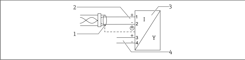
9 接线图: PROFIBUS PA / FOUNDATION Fieldbus
