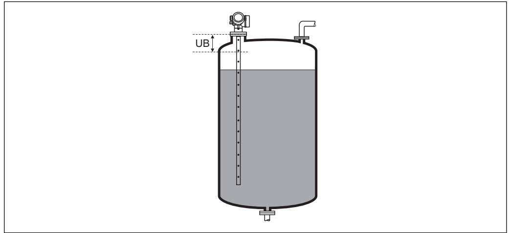
图 35 液位测量的盲区距离 (UB)
