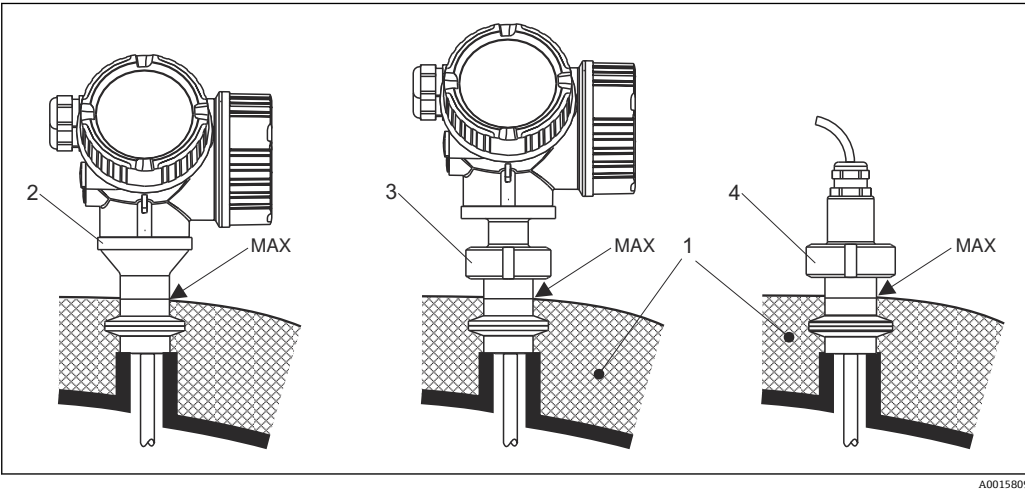
图 4 卫生型过程连接
