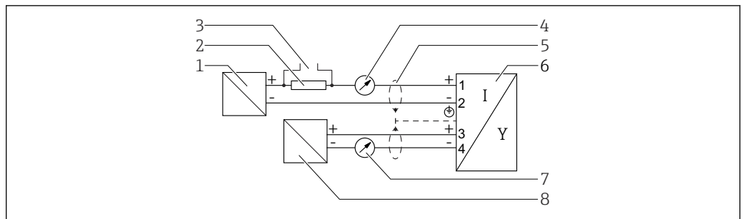
图 13 功能框图：4 ... 20 mA HART + 4 ... 20 mA 模拟量
