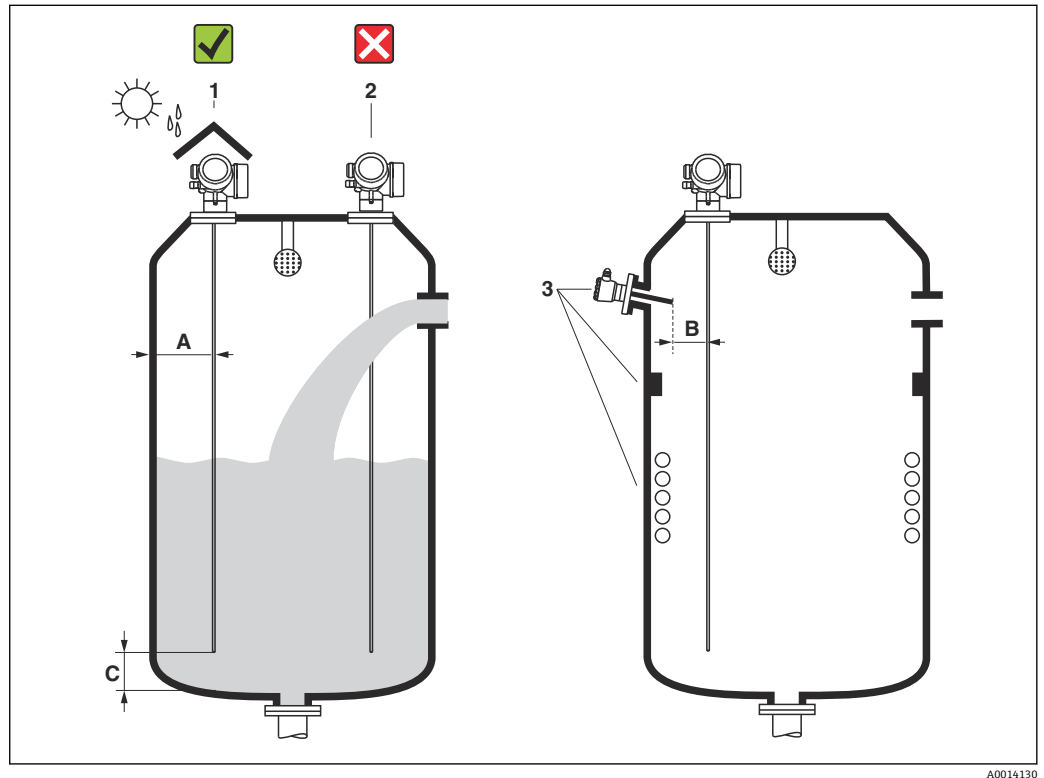
图 3 安装位置
