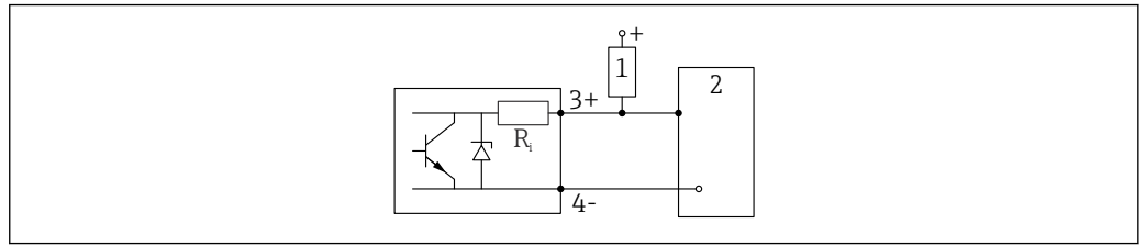
图 11 数字量输入的连接示例
