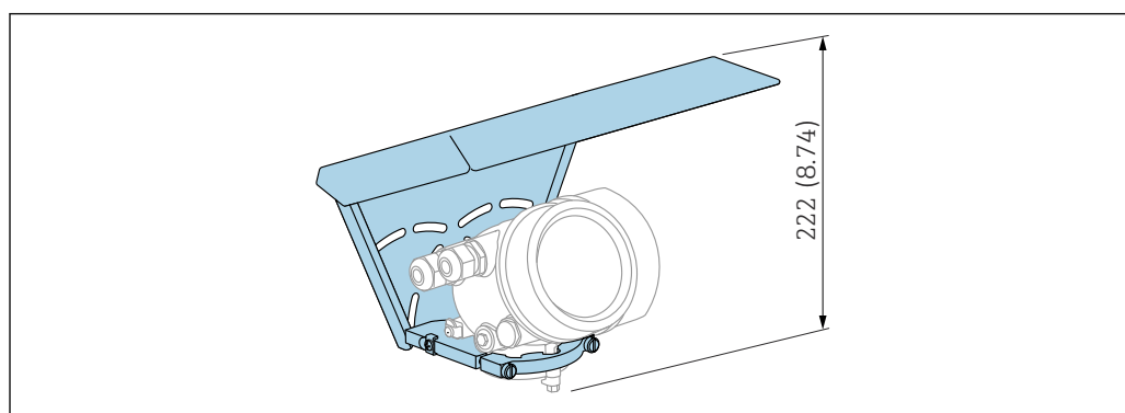
图 36 高度。测量单位 mm (in)
