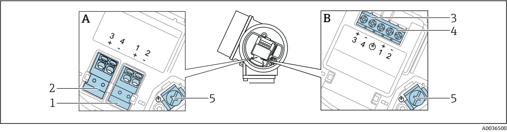
图 8 接线端子分配，两线制：4 ... 20 mA HART，开关量输出
