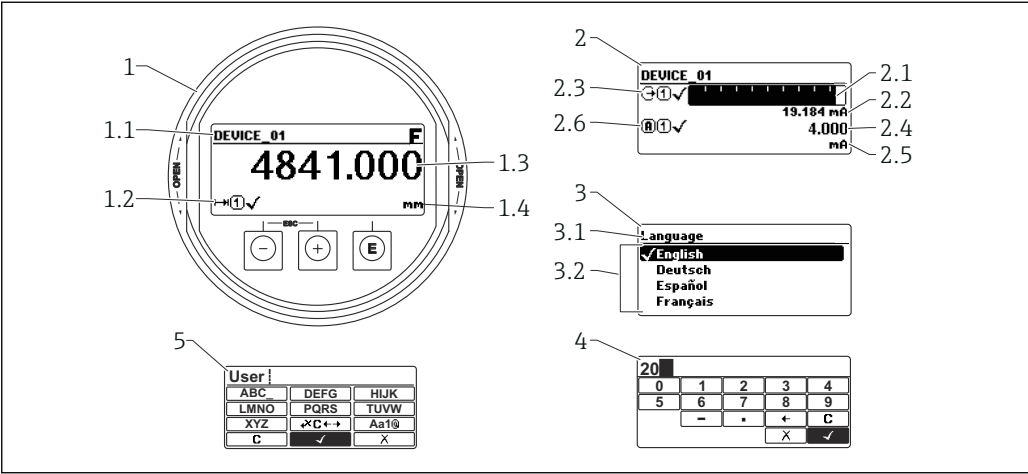
图 26 显示与操作单元的显示格式
