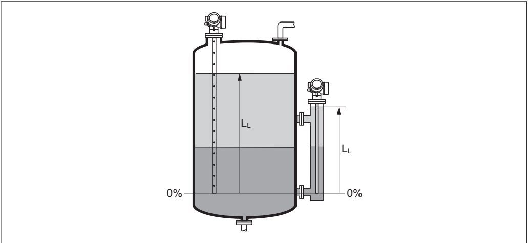
41 界面测量时的液位
