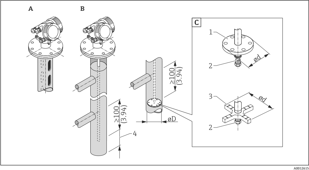
图 6 单位: mm (in) A 安装在导波管中 B 安装在旁通管中 C 对中环或对中盘 1 物位测量时的金属对中盘 (316L) 2 固定螺丝; 扭矩为 25 Nm ± 5 Nm 3 界面测量时的非金属对中盘 (PEEK、PFA) 4 探头末端与旁通管下端面间的最小距离; 参见下表
