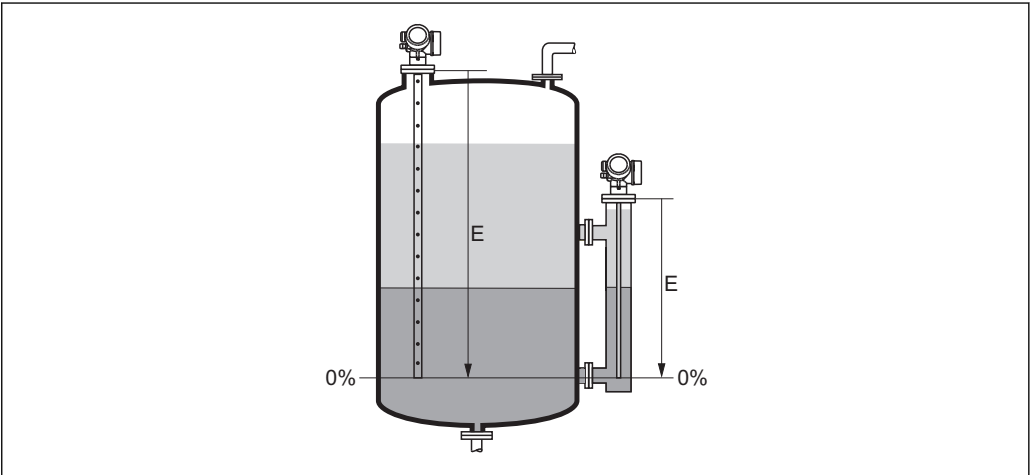
37 界面测量时空标 (E)
