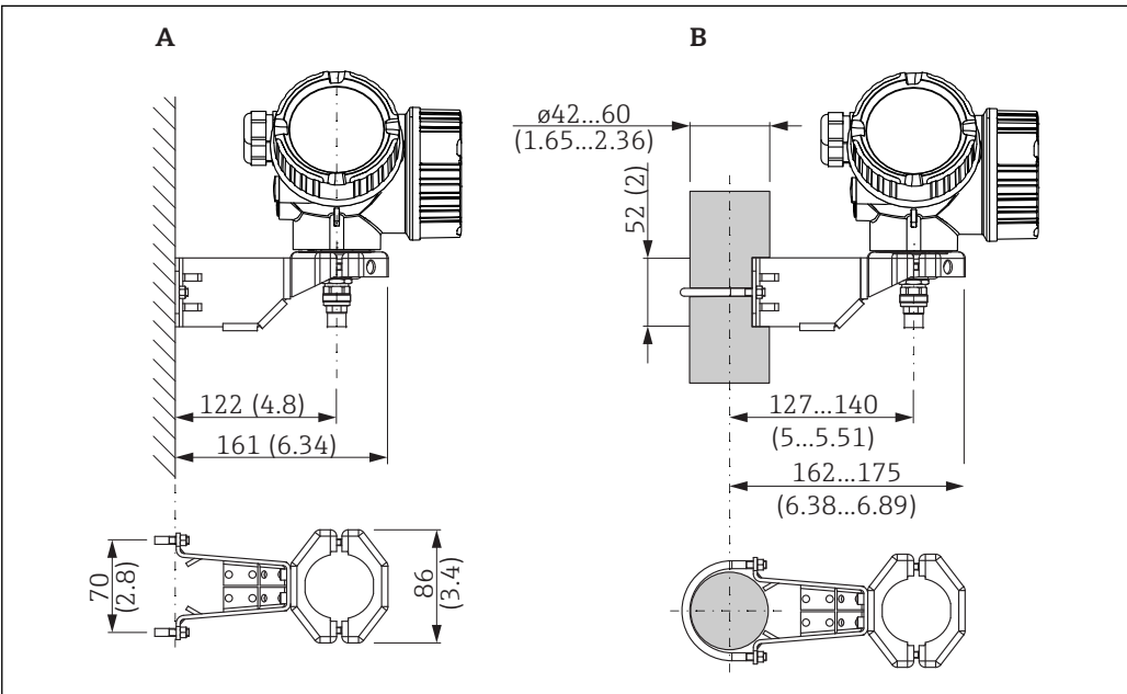
图 11 使用安装支架安装电子腔外壳；单位：mm (in)
