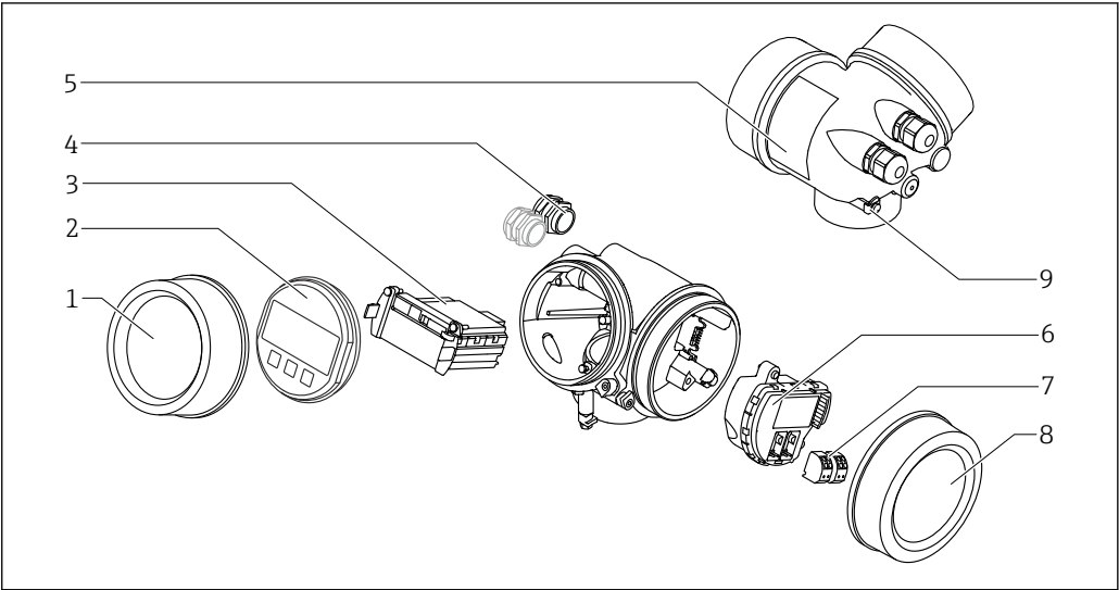
图 2 电子腔外壳结构示意图 1 电子腔盖 2 显示模块 3 主要电子模块 4 缆塞 (1 个或 2 个, 与仪表型号相关) 5 铭牌 6 I/O 电子模块 7 接线端子 (可插拔的压簧式接线端子) 8 接线腔盖 9 接地端
