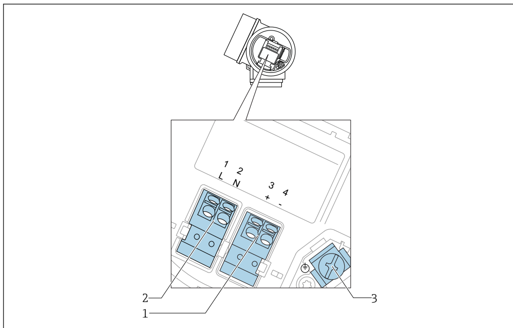
图 13 接线端子分配：四线制；4...20 mA HART (90 ... 253 V AC )
