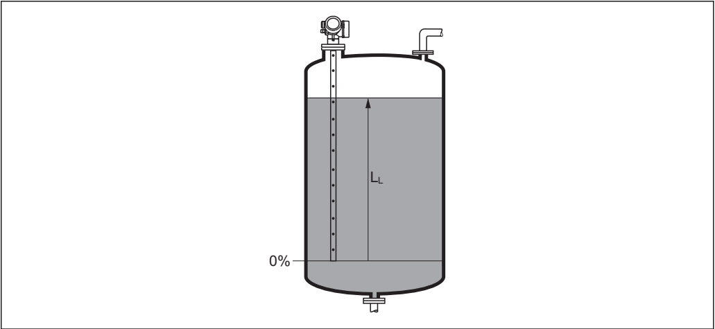
40 液位测量时的液位
