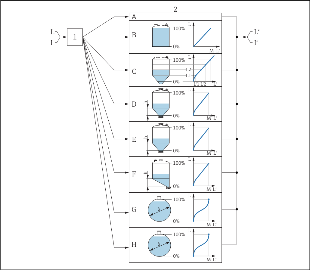
图 45 线性化：将物位和（相关）界面高度转换成体积或重量；转换取决于容器形状。
