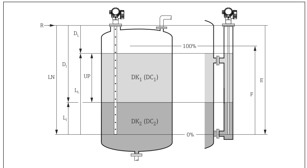
图 29 界面测量时的设置参数
