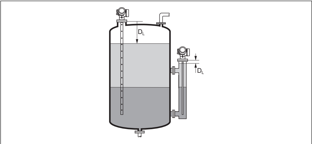
43 界面测量时的距离
