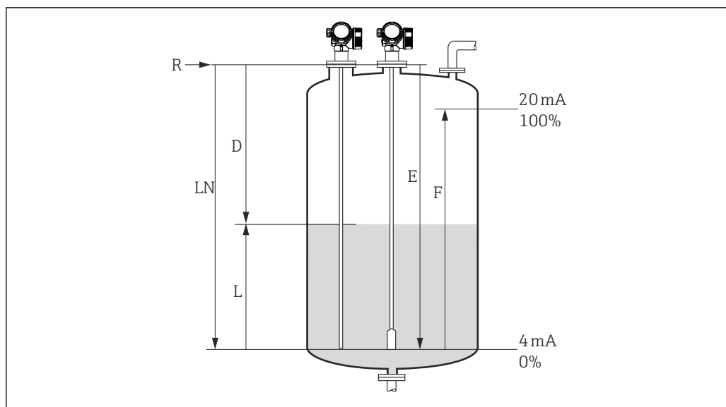
图 28 液位测量时的设置参数
