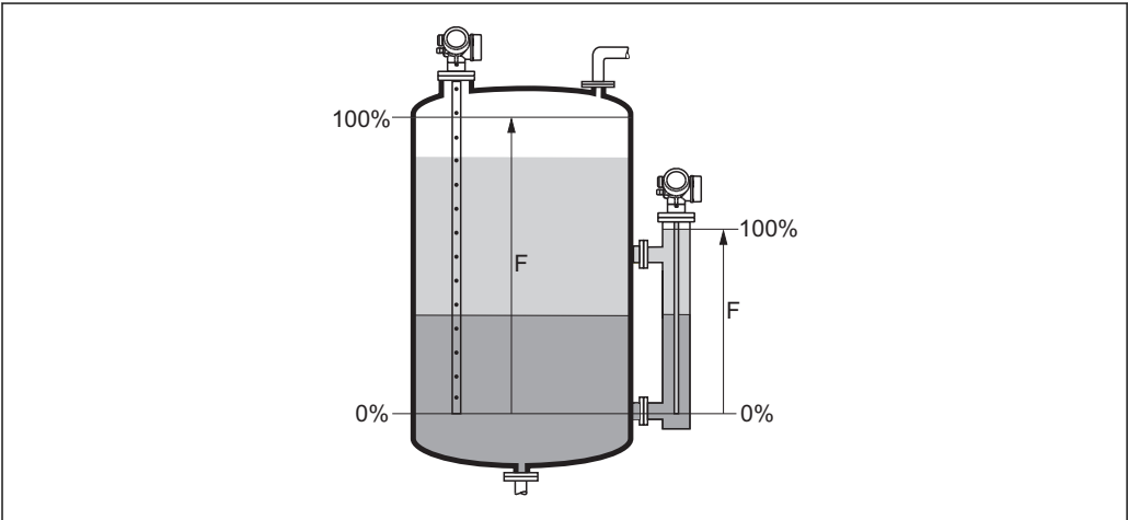
39 界面测量时的满标 (F)
