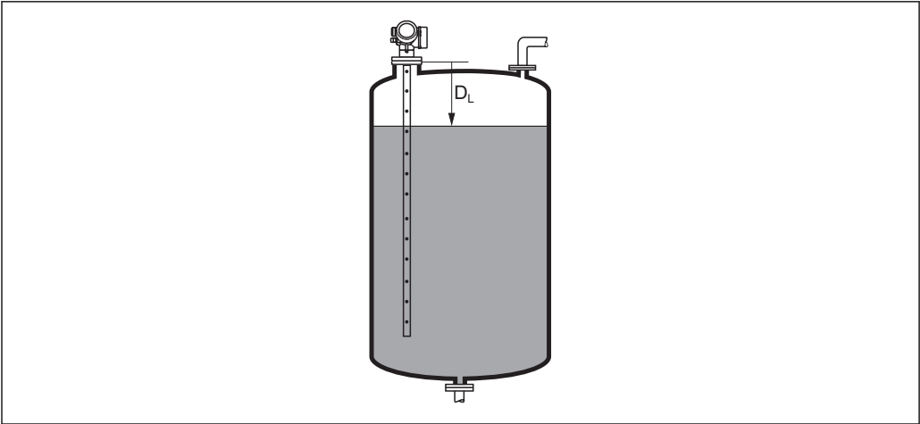
42 液位测量时的距离
