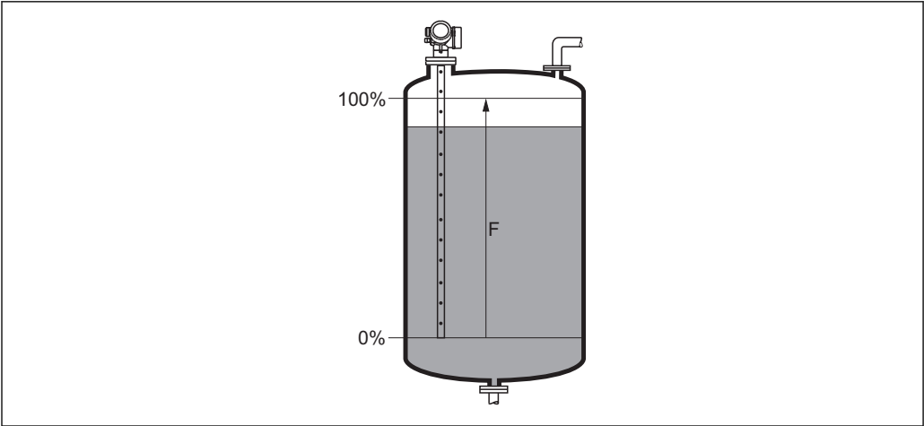
38 液位测量时的满标 (F)
