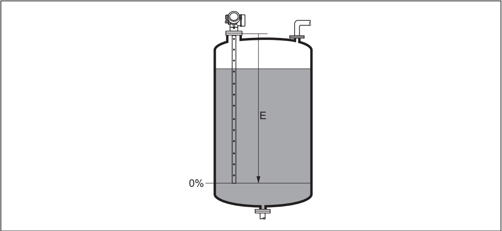
36 液位测量时空标 (E)
