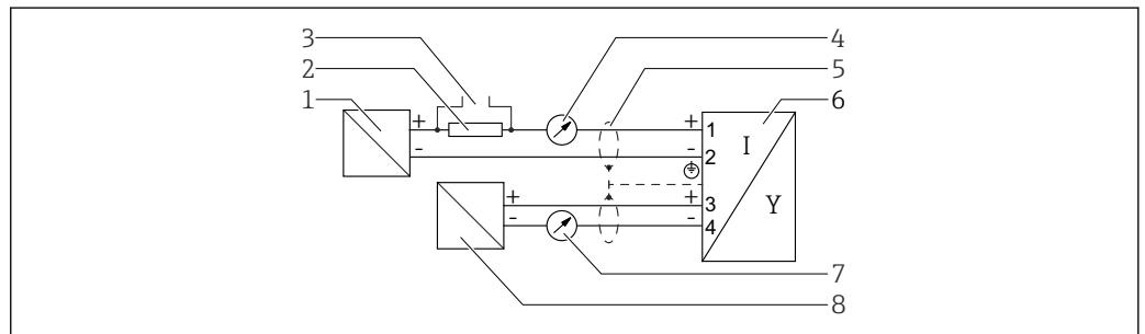
图 12 功能框图：4 ... 20 mA HART + 4 ... 20 mA 模拟量
