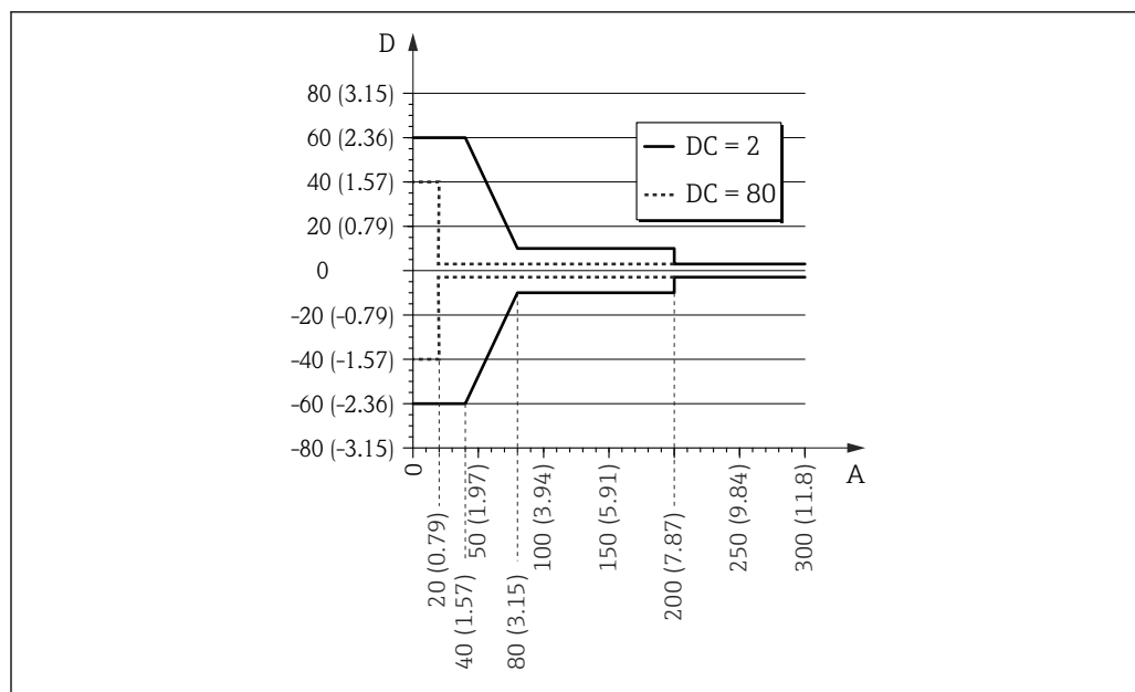
图 21 杆式探头和同轴探头底部附近的测量误差
