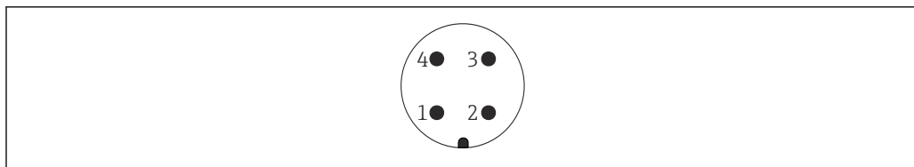
图 19 M12 插头的针脚分配
