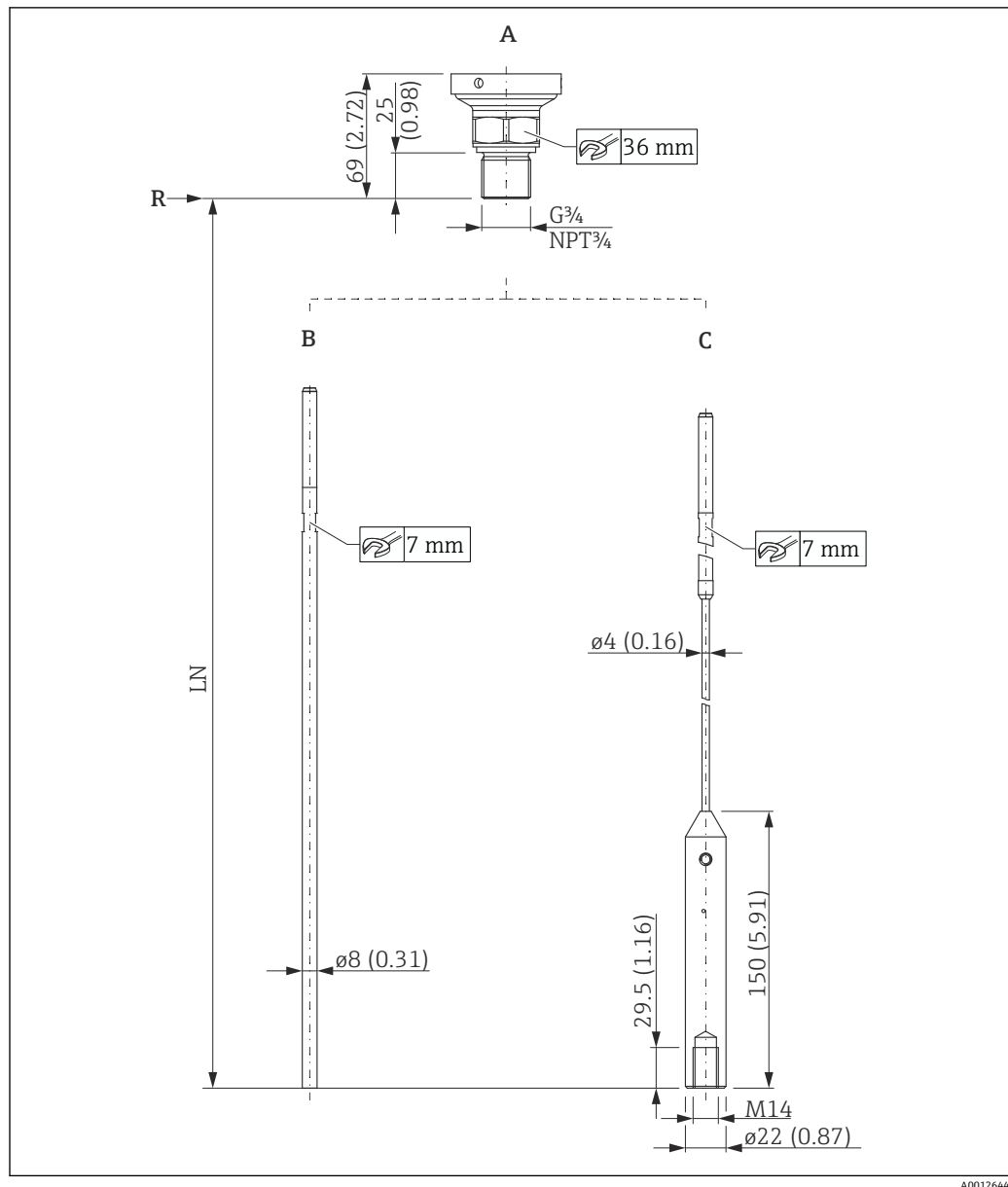
31 FMP50: 过程连接和探头。测量单位 mm (in)
