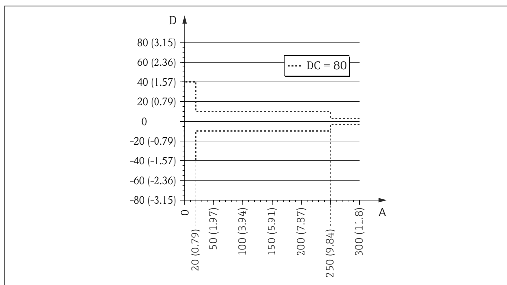
图 22 缆式探头底部附近的测量误差
