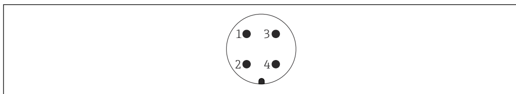
图 20 7/8"插头的针脚分配
