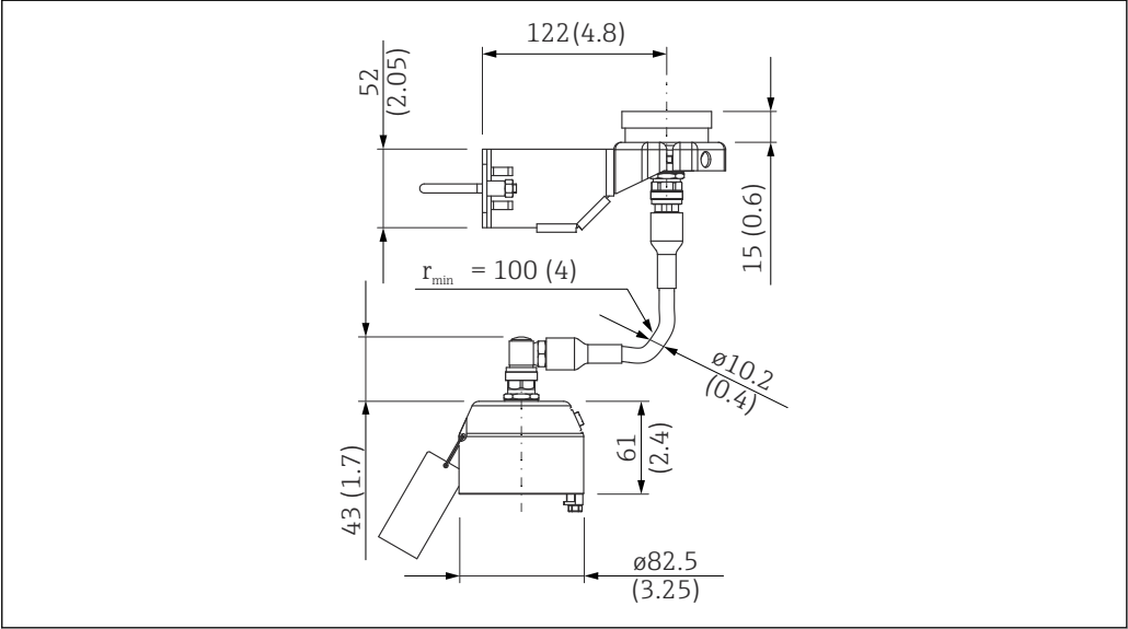
30 分体式探头连接件；连接电缆长度为订购长度。测量单位 mm (in)
