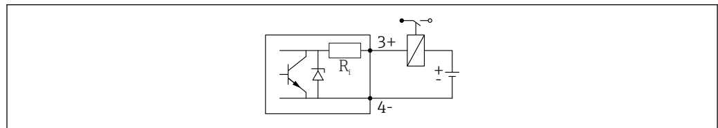
图 9 继电器的连接示例
