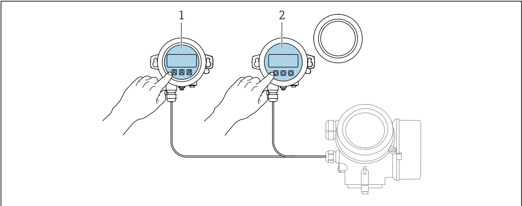
35 FHX50 的操作选项 1 显示与操作单元 SD03，光敏键操作，可以在玻璃盖板外部操作 2 显示与操作单元 SD02，按键操作；必须打开盖板
