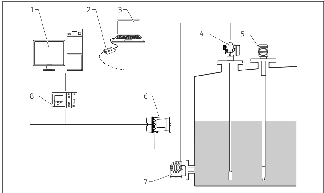
图 40 完整测量系统包括:
