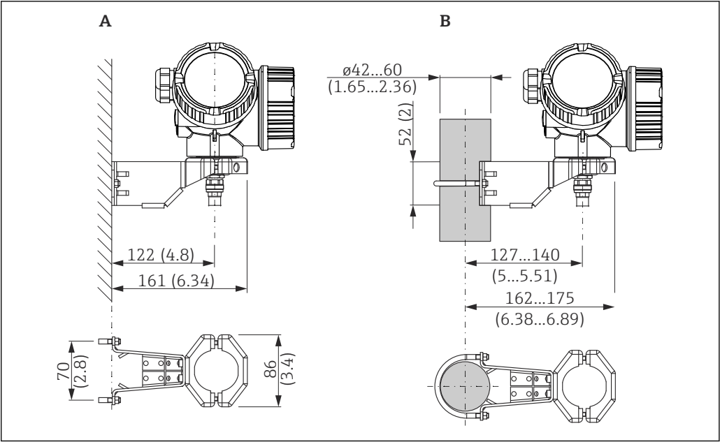
29 电子腔外壳安装架。测量单位 mm (in)
