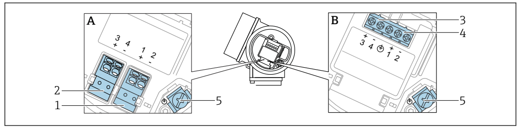
图 11 接线端子分配，两线制：4 ... 20 mA HART，4 ... 20 mA
