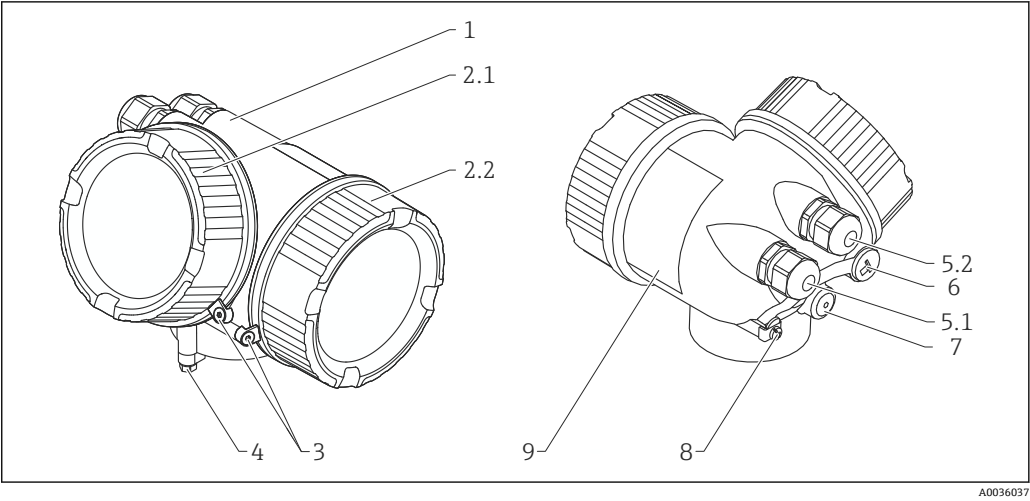
33 材质：GT20 外壳
