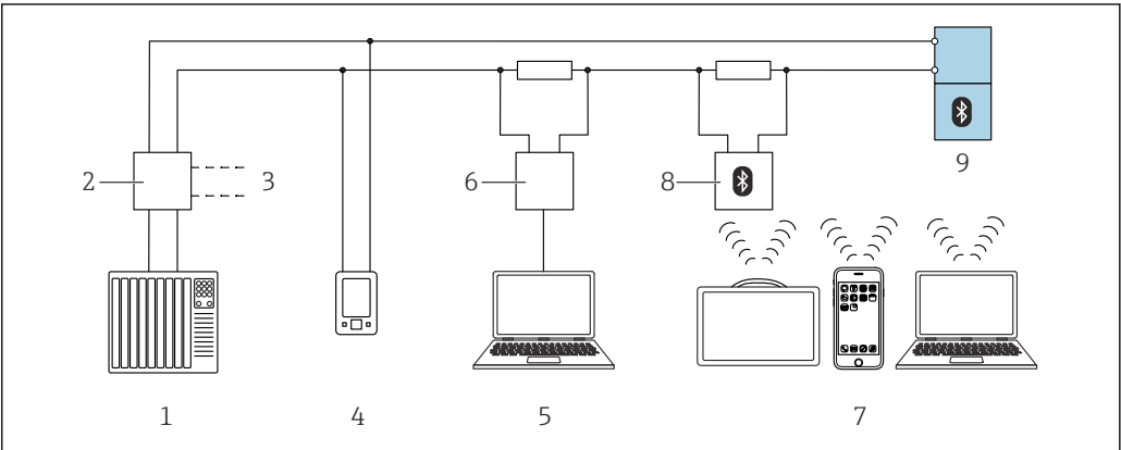
36 通过 HART 通信实现远程操作
