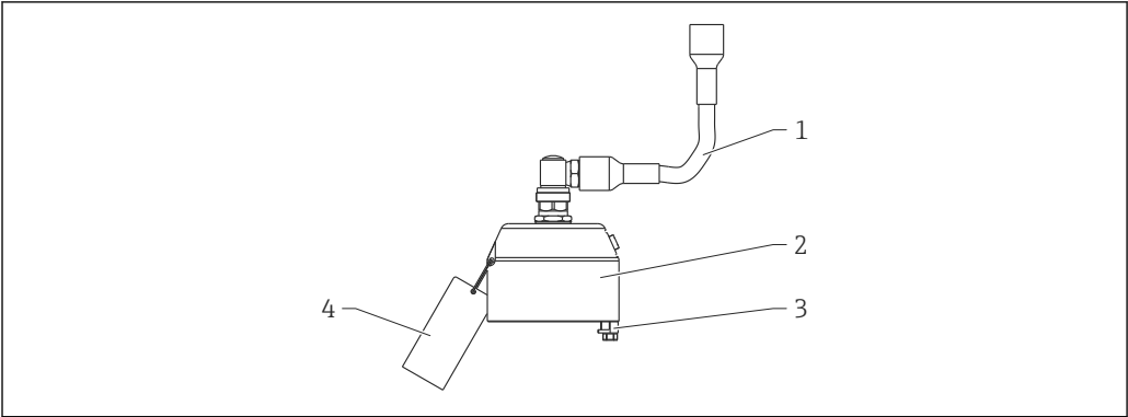
图 34 材质：带“分体式传感器”的仪表型号的转接头和电缆
