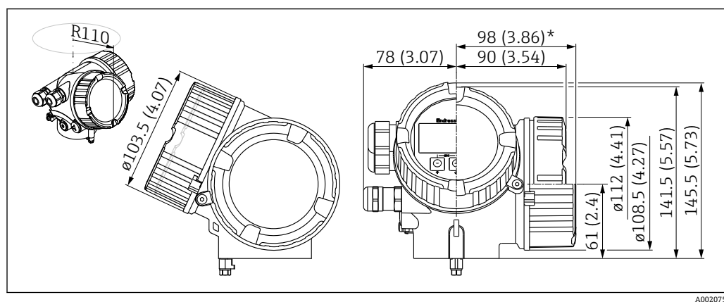
图 28 GT20 外壳 (铝, 带涂层)。测量单位 mm (in)
