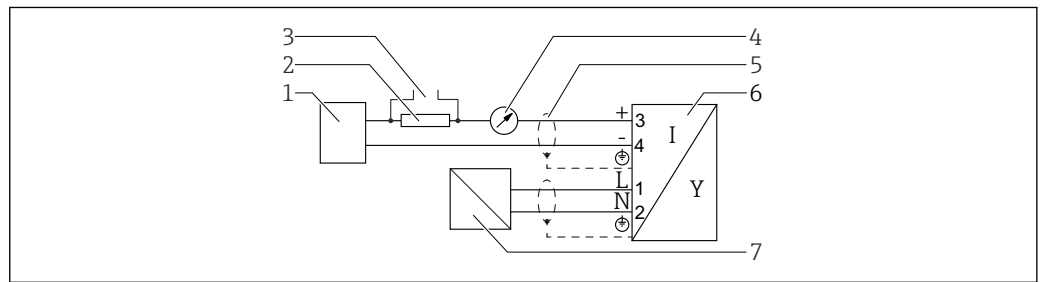
16 功能框图, 四线制: 4 ... 20 mA HART (90 ... 253 V AC )
