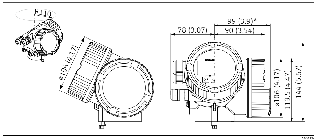
图 27 GT19 外壳 (塑料 PBT)。测量单位 mm (in)
