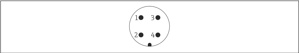
图 11 7/8"插头的针脚分配
