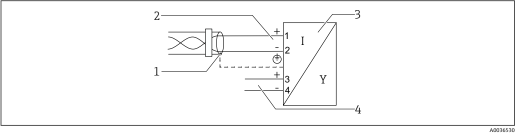
图 10 功能框图: PROFIBUS PA / FOUNDATION Fieldbus
