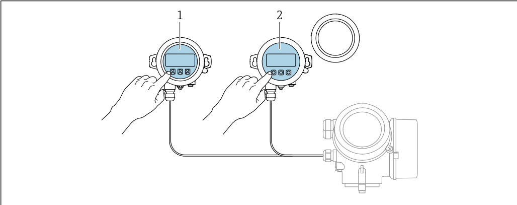
图 14 FHX50 的操作选项
