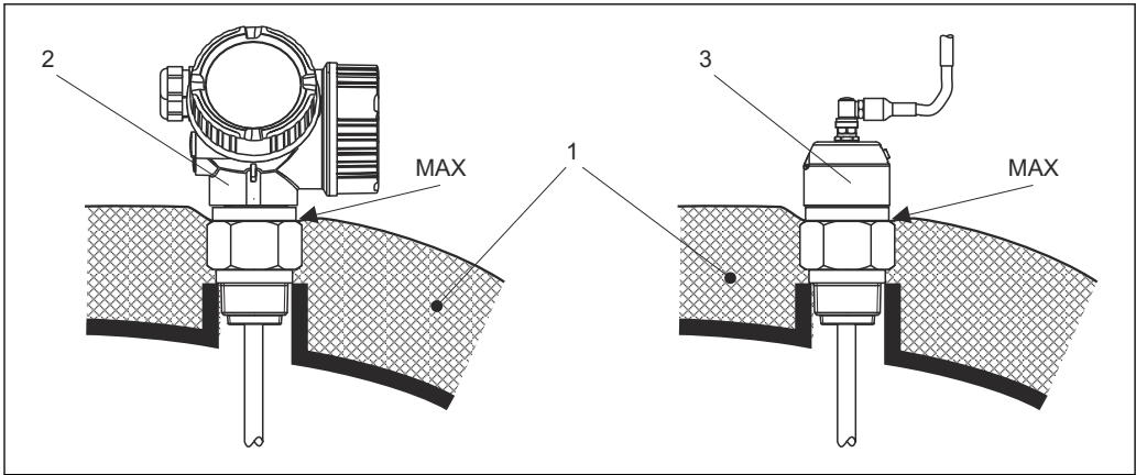
图 5 螺纹过程连接
