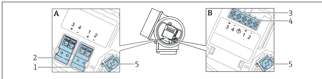
图 9 接线端子分配：PROFIBUS PA / FOUNDATION Fieldbus
