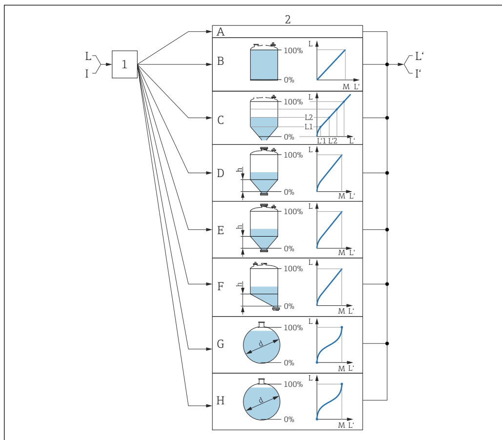
41 线性化：将物位和（相关）界面高度转换成体积或重量；转换取决于罐体形状
