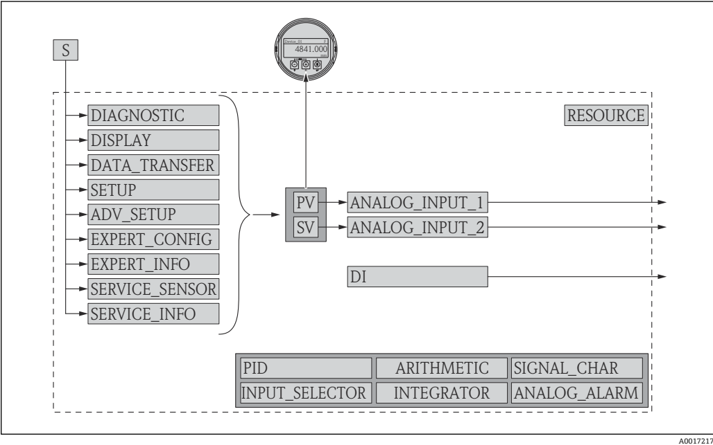
图 20 设备块的出厂设置
