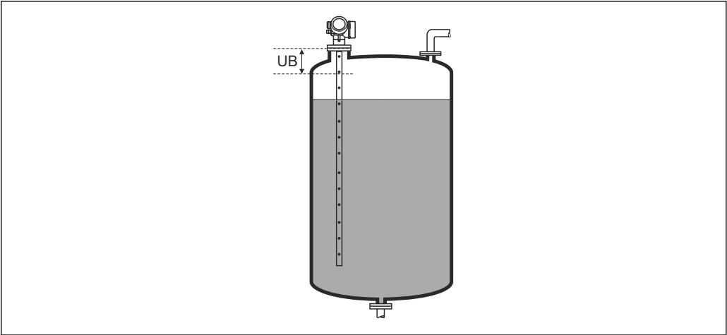
43 液位测量的盲区距离 (UB)
