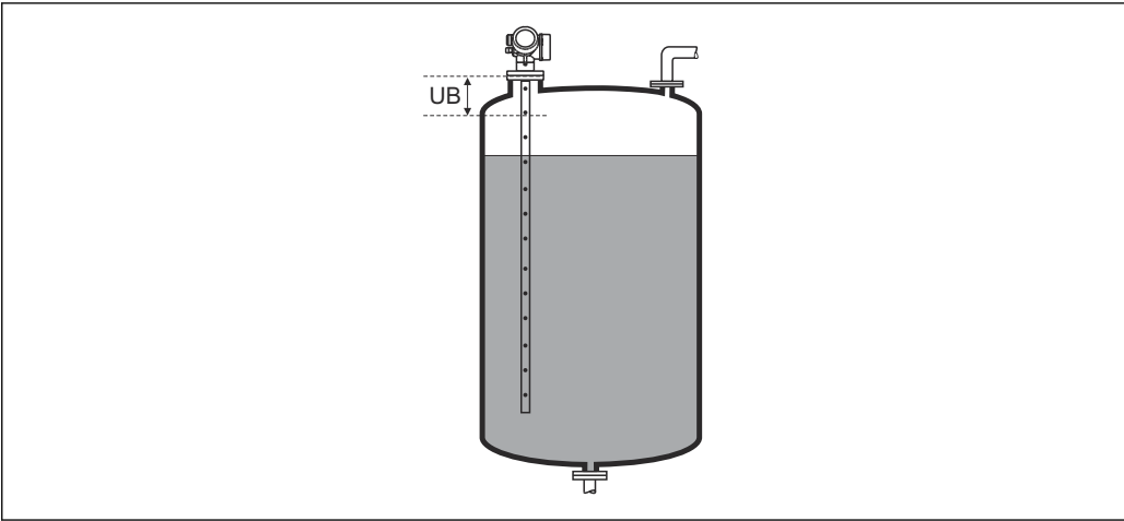
40 液位测量的盲区距离 (UB)
