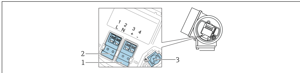
图 8 接线端子分配，四线制：4 ... 20 mA HART (90 ... 253 V AC )
