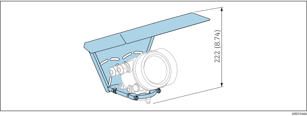
图 31 高度。测量单位 mm (in)
