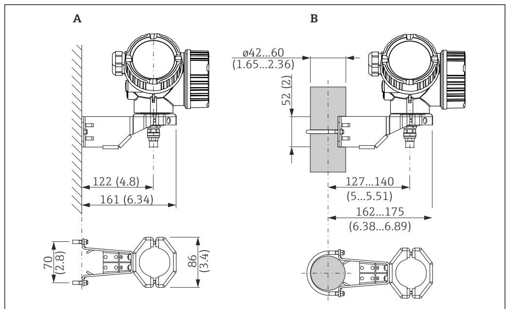
图 33 电子腔外壳安装架; 单位: mm (in)
