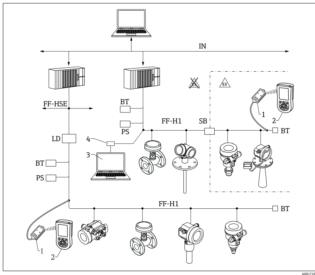
15 FOUNDATION Fieldbus 系统架构及组件
