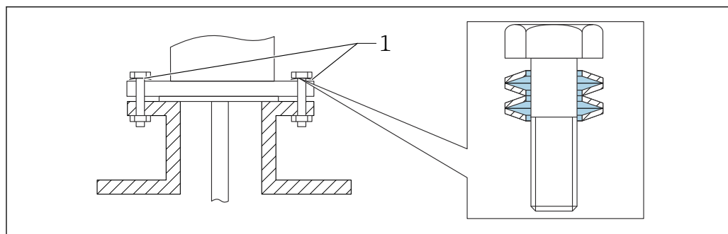
1 弹簧垫圈
