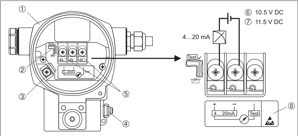
图 5: 4...20 mA HART 电气连接示意图 → 另请参见章节 5.2.1“供电电压”，→ 19。
