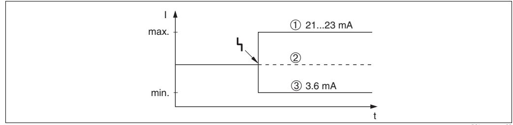
图 13: 报警时的电流输出
