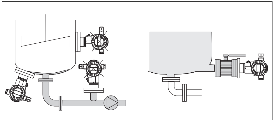
图 1: 液位测量布置
