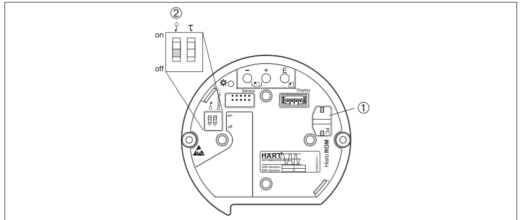
图 11: 可选 HistoROM®/M-DAT 存储单元模块的电子插件
