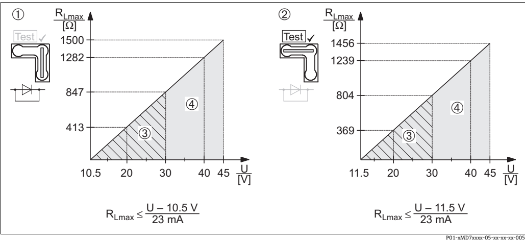
图 8: 负载图, 参考跳线针位置和防爆图标 (→ 19, 章节 5.2.1 “测量 4...20 mA 测试信号” 章节。)
