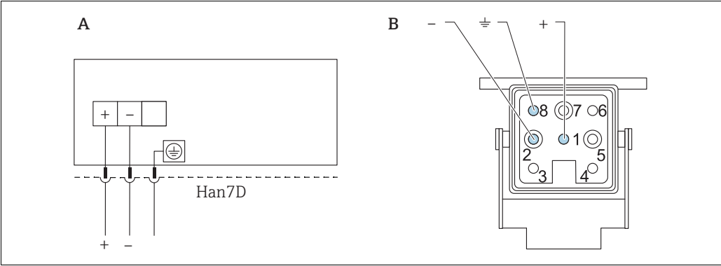
图 6: A 带 Haring Han7D 插头的仪表的电气连接示意图 B 设备接线示意图 - 棕色 / 绿色 / 黄色 + 蓝色
