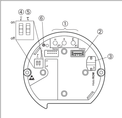
图 10: 内部操作按键 1 操作按键 2 选配显示单元的插槽 3 选配 HistoROM®/M-DAT 的插槽 4 DIP 开关, 锁定 / 解锁测量值参数 5 DIP 开关, 阻尼时间开关切换 6 绿色 LED 指示灯, 表示接收参数
