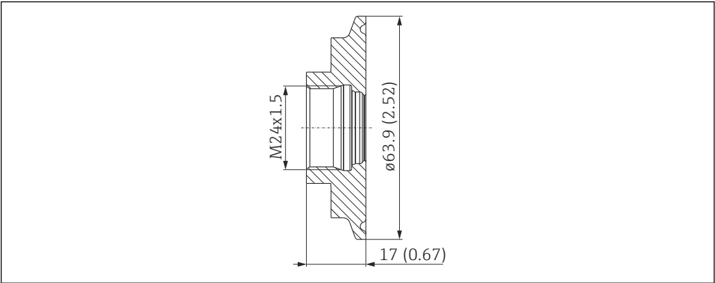
38 2"卡箍（DIN 32676、ISO 2852）（M24）过程转接头的外形尺寸示意图。测量单位 mm (in)
