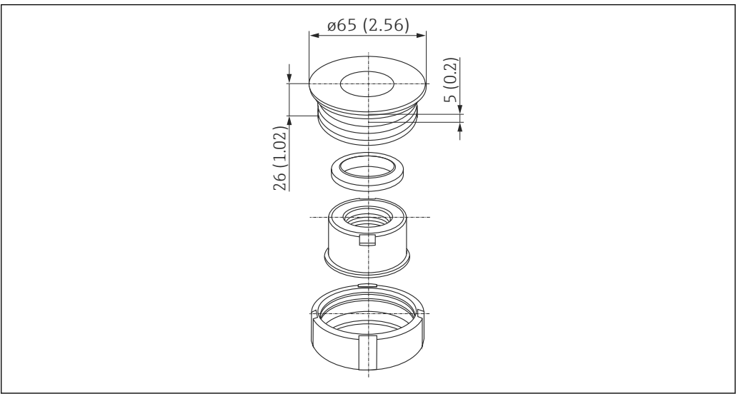
8 G 1 焊接接头（可调整传感器位置）的外形尺寸示意图。测量单位 mm (in)
