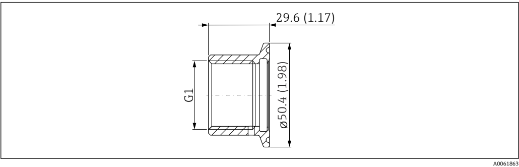
60 1½"卡箍 (G1) 过程转接头的外形尺寸示意图。测量单位 mm (in)
