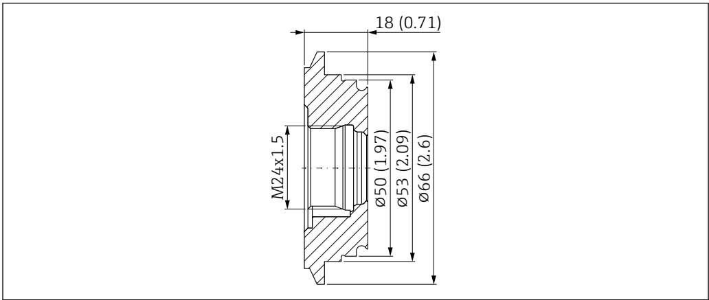
31 Varivent F DN25 (M24) 过程转接头的外形尺寸示意图。测量单位 mm (in)
