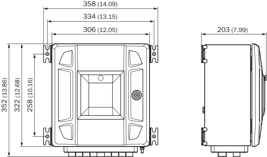
图 139 1 级 2 类接口单元（尺寸单位：mm（in））
