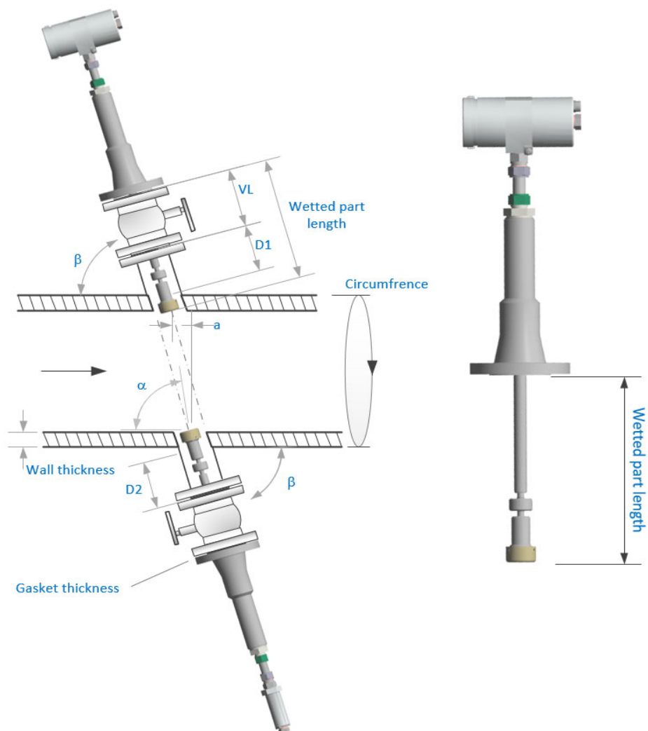
图 36 安装 F1F-S、F1F-M、F1F-H (对穿型)
