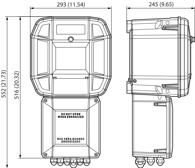
图 141 1 区 Ex d e 接口单元 (尺寸单位: mm (in) )
