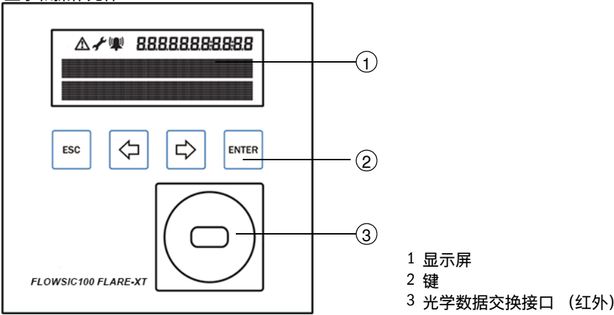
图 121 显示和操作元件
