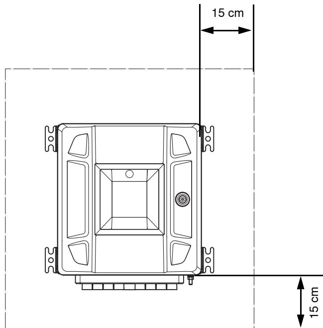
图 64 接口单元周围的距离（适用于所有仪器结构）
