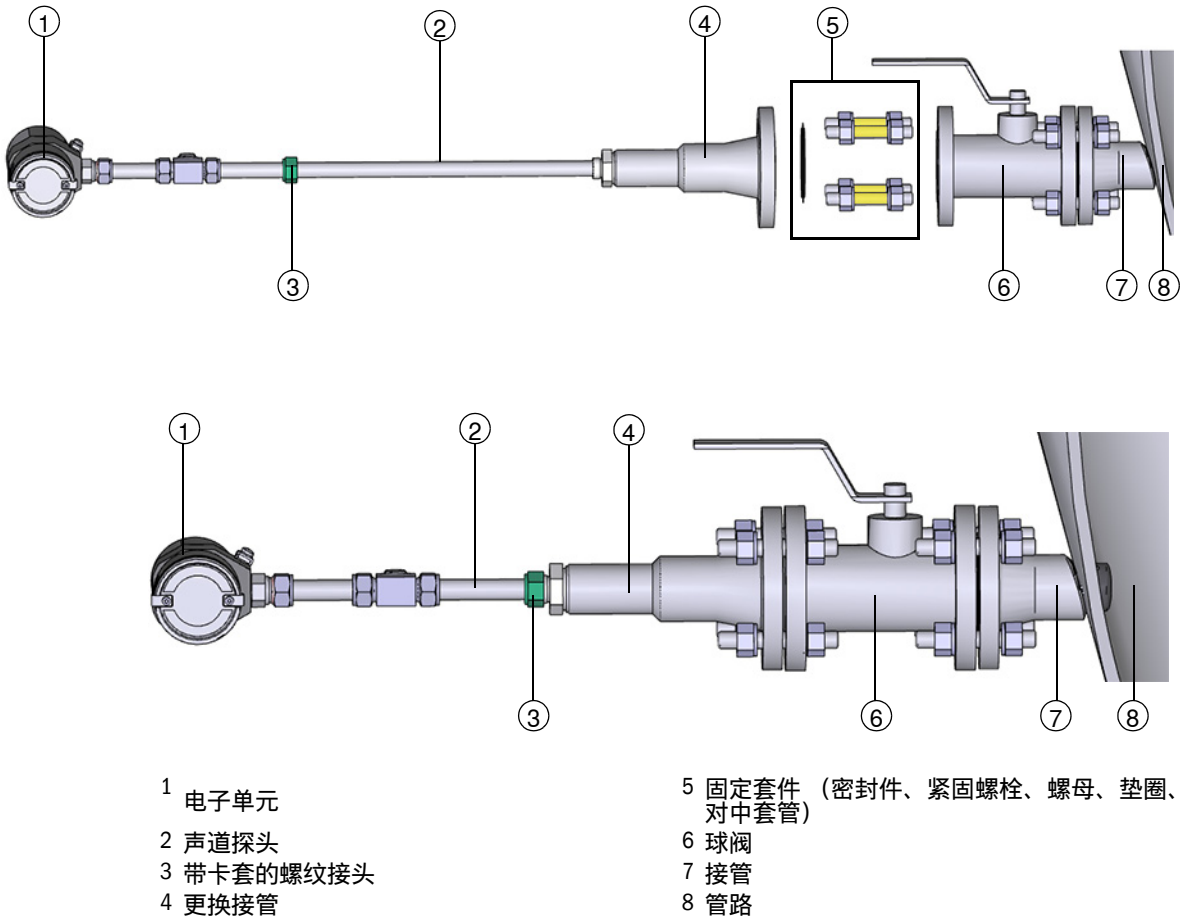
图 32 总览
