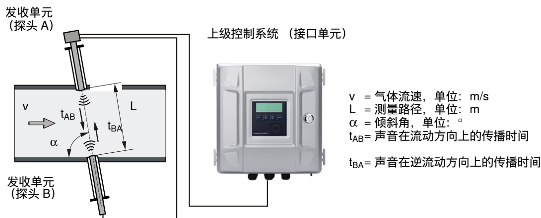
FLOWSIC100 Flare-XT 功能原理
