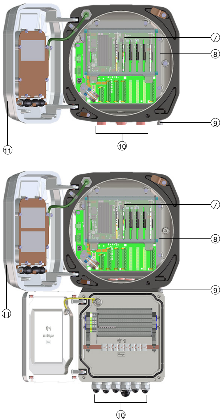
图 59 Ex d 和 Ex de 总览 — 打开的外壳
