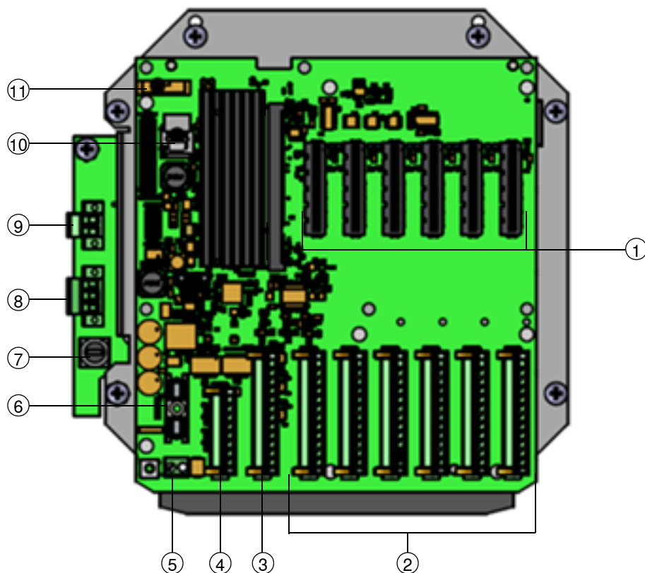
图 80 主机板
