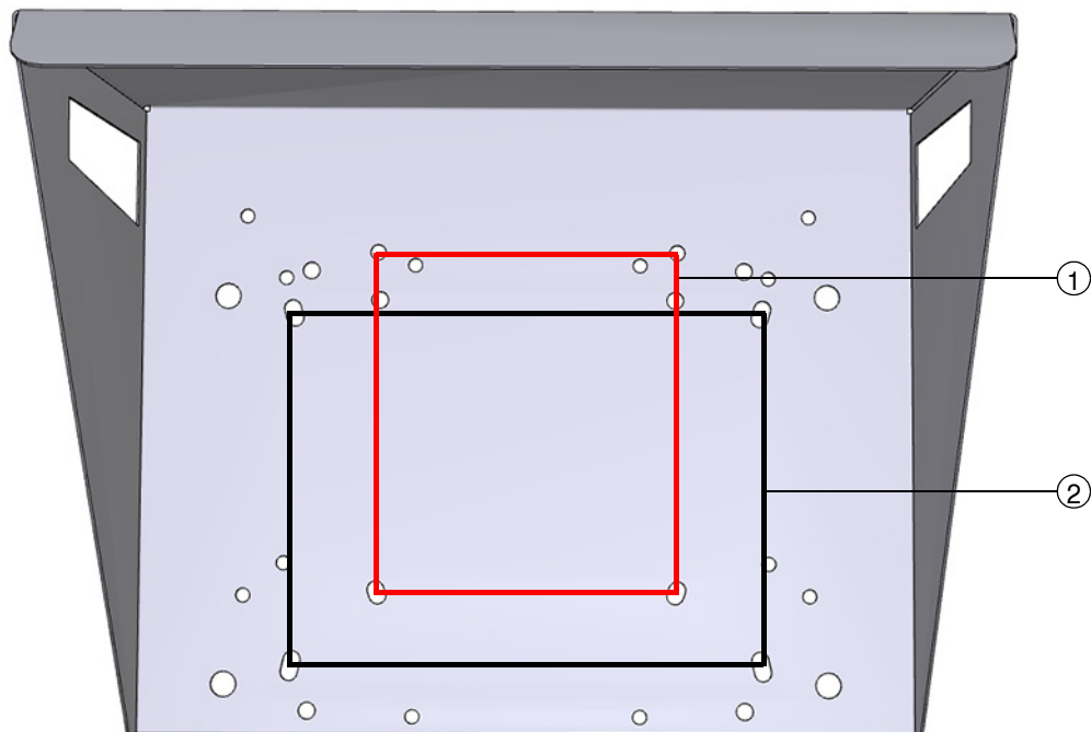
图 69 在防晒（雨）罩上安装接口单元
