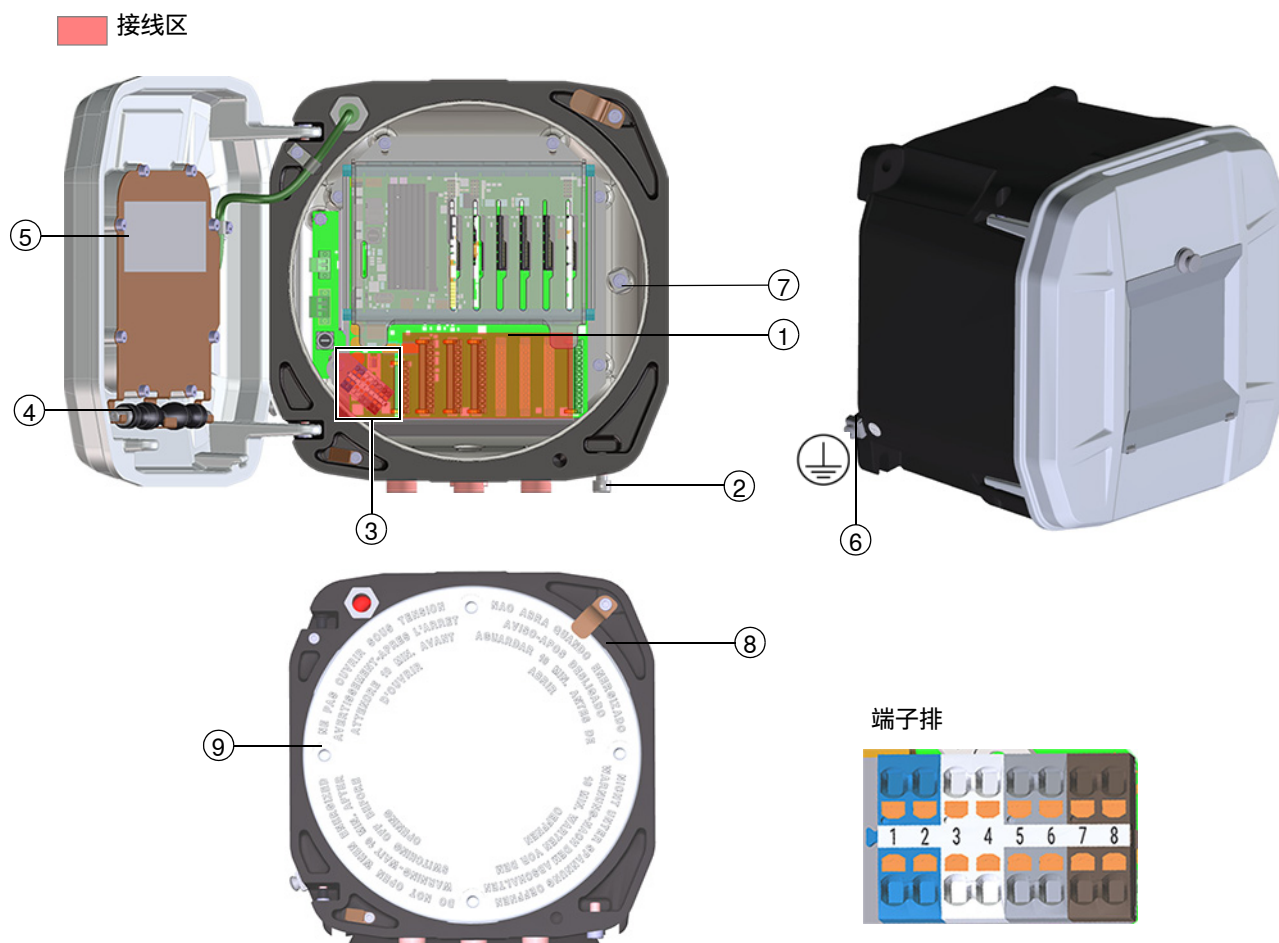
图 78 1 区接口单元 Ex d 的接线区和内部电子设备
