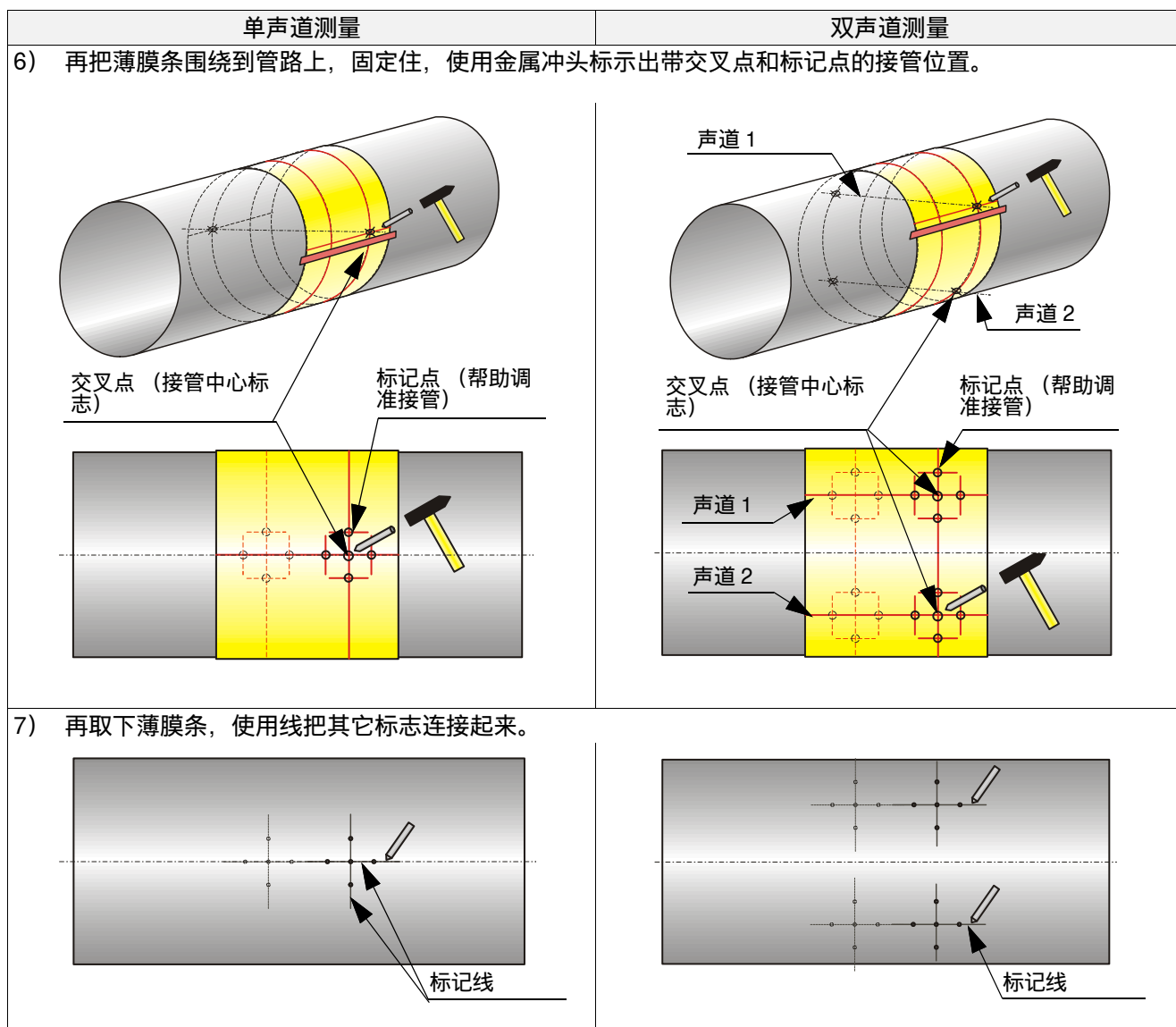
图 26 在管路上标示出对穿型的接管位置
