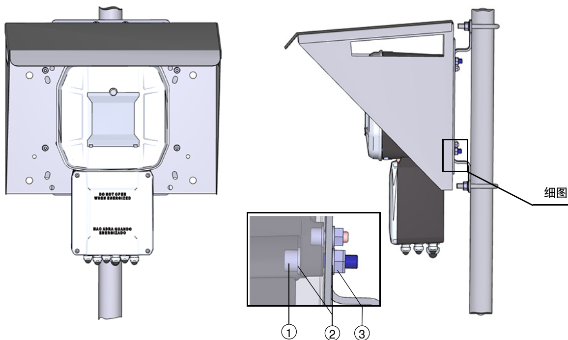
图 73 1 区接口单元与防晒（雨）罩安装在一起
