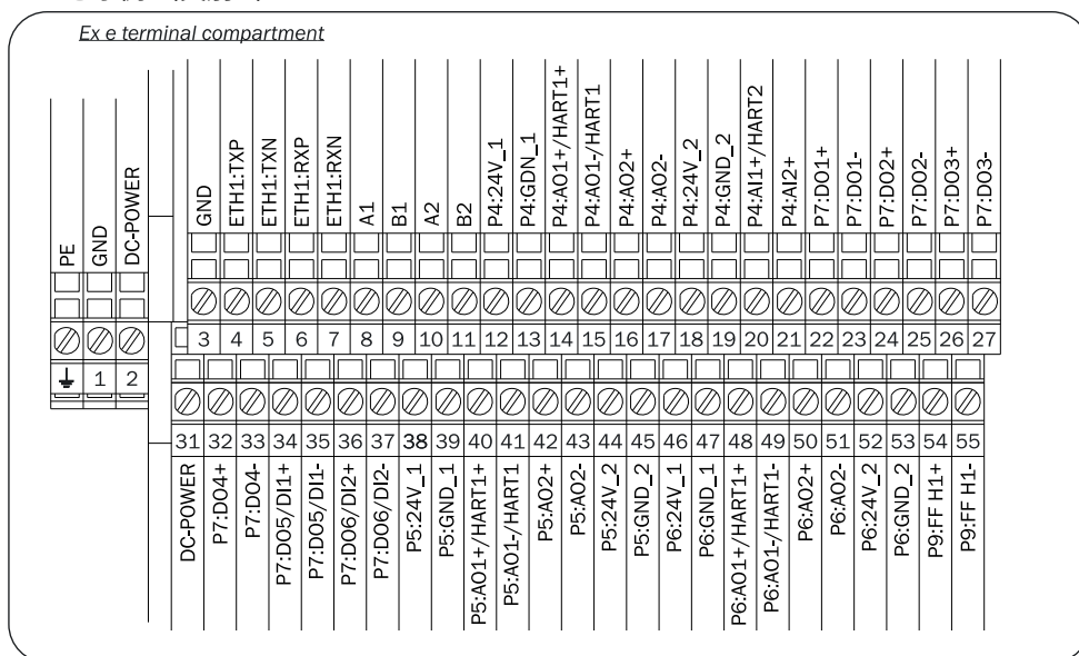
图 89 DC 组态示例 (类别 L)
