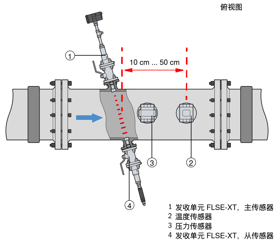
图 6 安装位置
