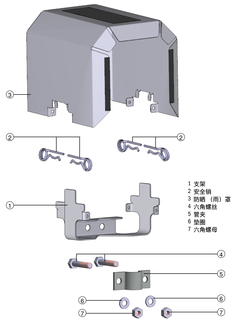
图 44 防晒（雨）罩总览
