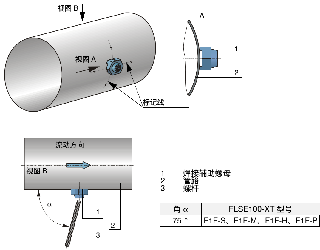
图 29 给焊接辅助螺母定位
