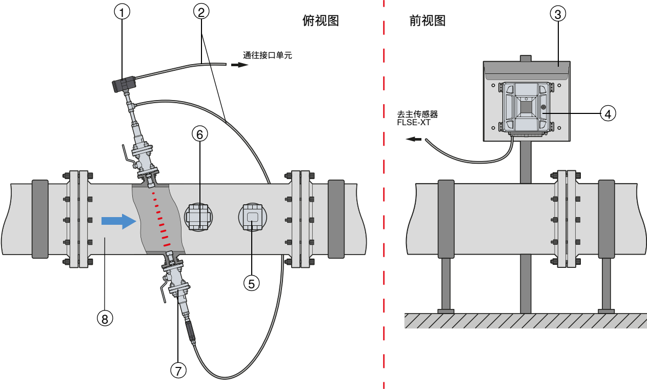
图 2 FLOW SIC100 Flare-XT 系统总览
