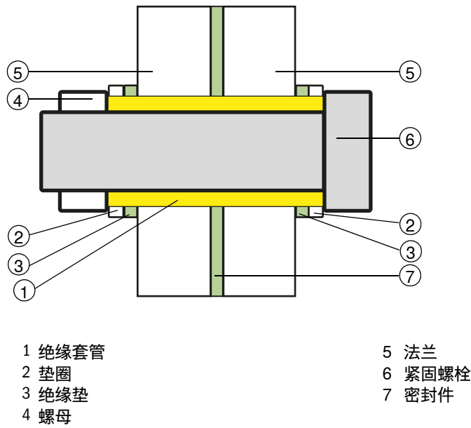
图 34 使用接管绝缘套件
