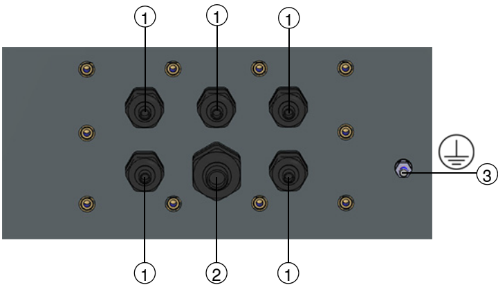
图 56 公制电缆接头（选配提供 9 个电缆接头）
