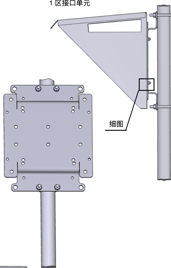
1 区接口单元
