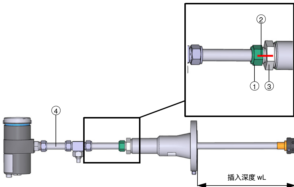
给卡套定位（总览）
