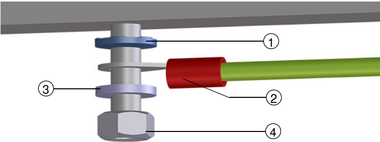
图 81 保护地线接头
