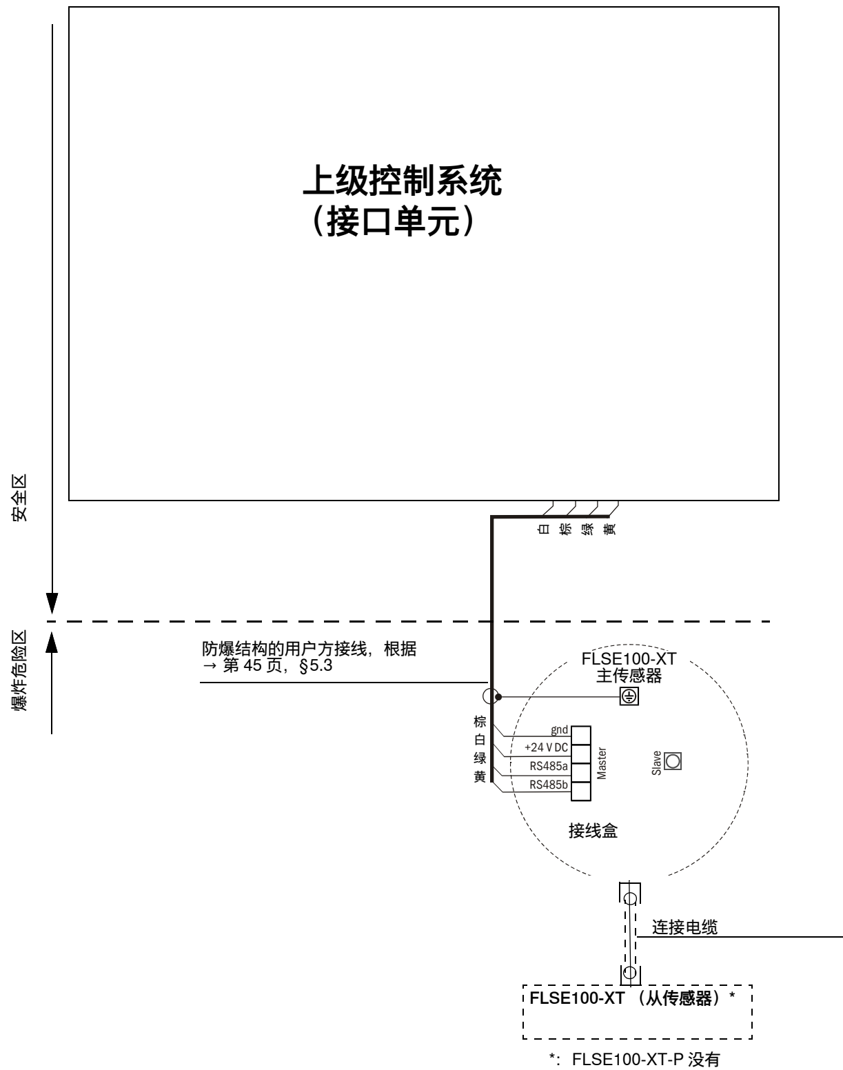
图 47 收发单元的接线
