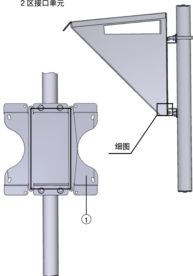
图 70 在安装板上安装防晒（雨）罩 2 区接口单元
