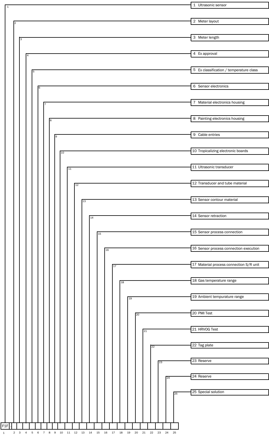
图 151 发收单元 FLSE-XT （总览）
