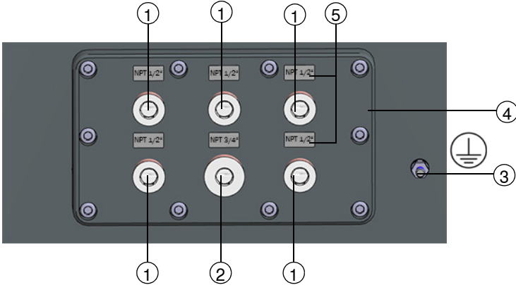
图 57 密封塞 NPT（选配提供 9 个电缆穿入口）
