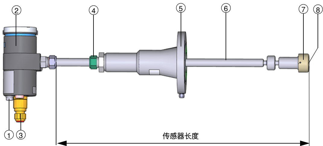
图 13 F1F-H (仅画出主传感器)
