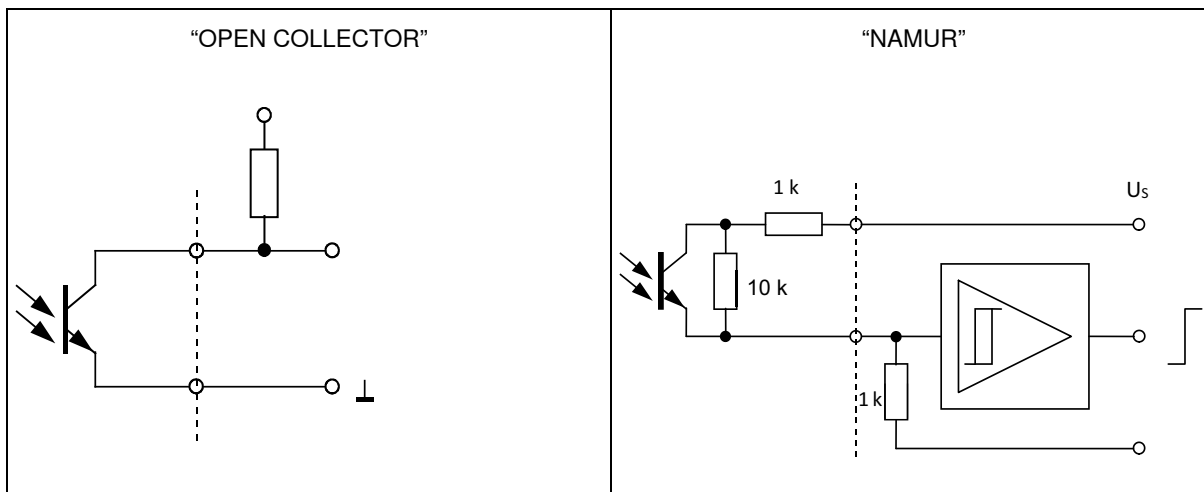
图 92 DO 开关（Open Collector - Namur）
