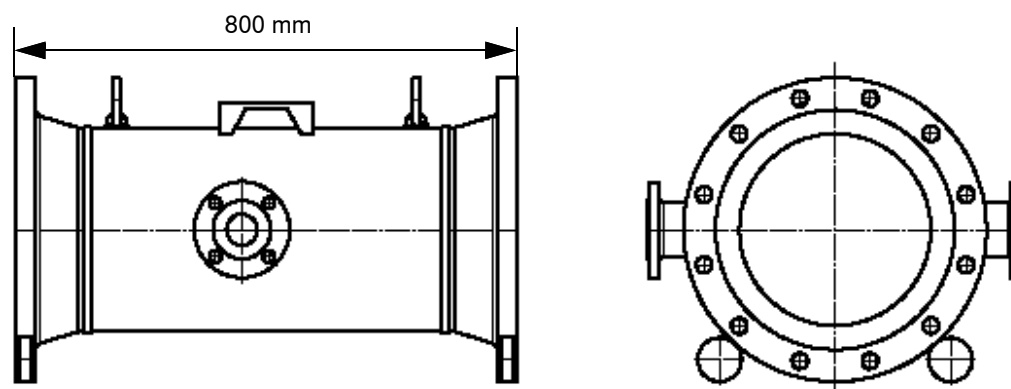
图 16 选配“测量管”（示例）
