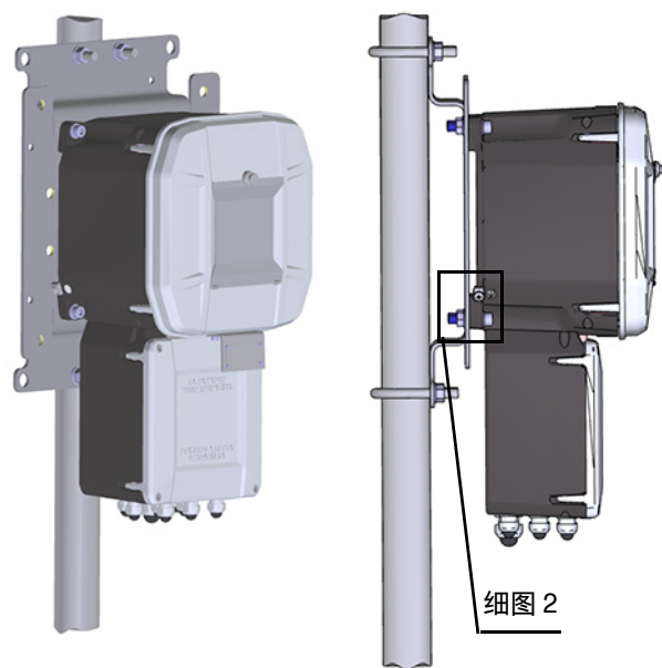
1 区接口单元
