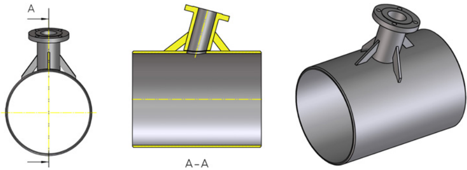
图 19 使用节点板作为接管的机械支撑（示例）
