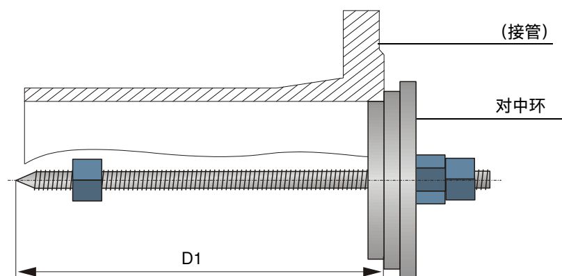
图 31 确定有效接管长度
