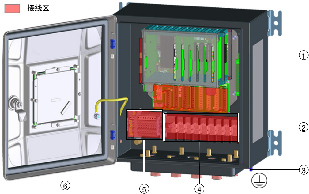
图 77 接口单元的接线区和内部电子设备
