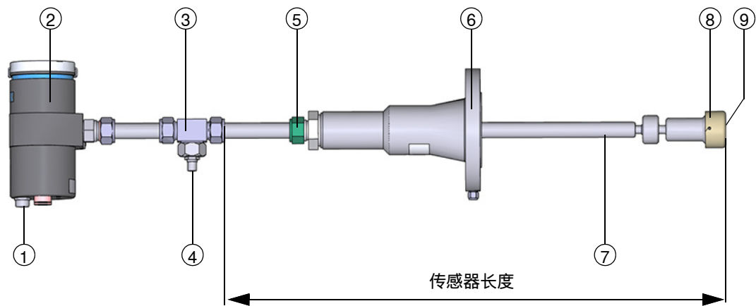
图 12 F1F-M (仅画出主传感器)
