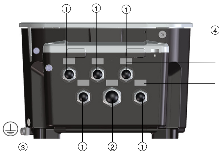
图 62 Ex d e 外壳，公制电缆接头（选配提供 9 个电缆接头）
