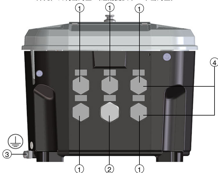
图 60 Ex d 外壳，公制密封塞（选配提供带 9 个密封塞）
