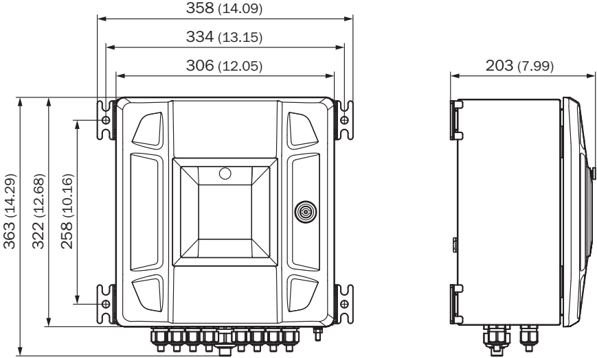
图 138 2 区接口单元（尺寸单位：mm（in））
