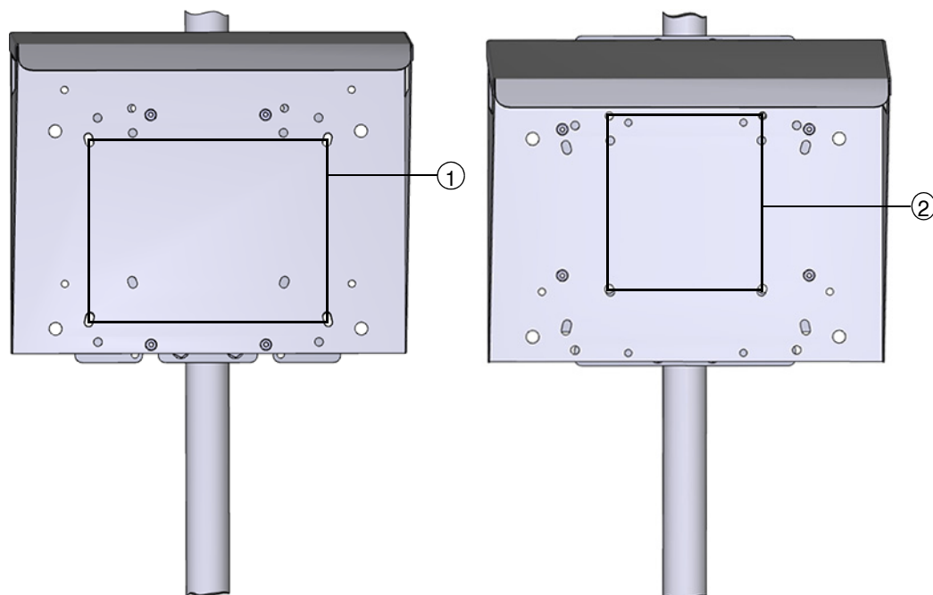
图 71 在防晒（雨）罩上安装接口单元
