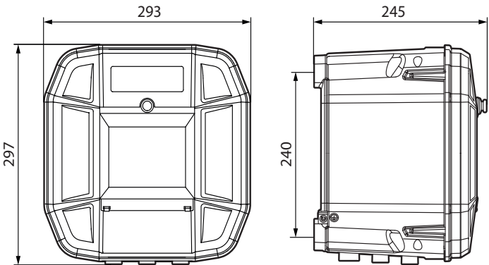
图 140 1 区 Ex d 接口单元 (尺寸单位: mm (in) )
