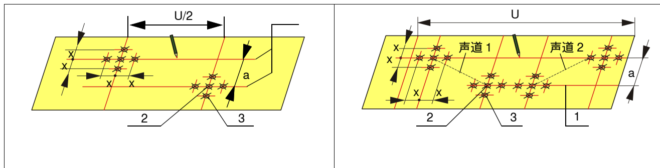
图 26 在管路上标示出对穿型的接管位置
