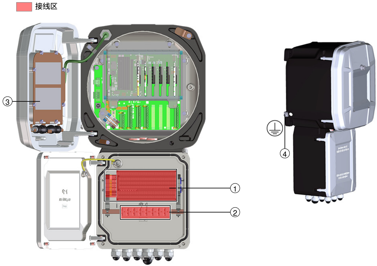
图 79 1 区接口单元 Ex d e 的接线区和内部电子设备
