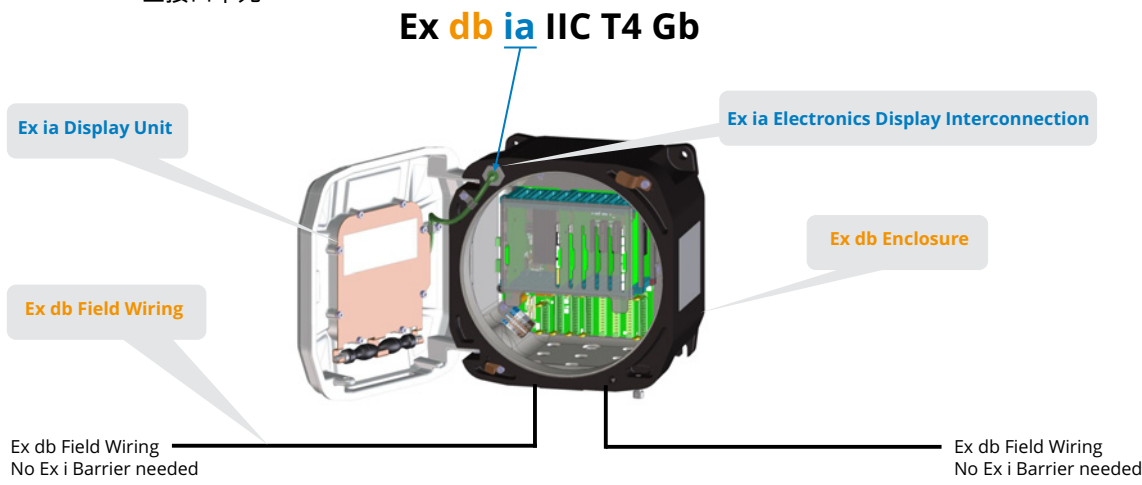
图 155 1 区接口单元 Ex d
