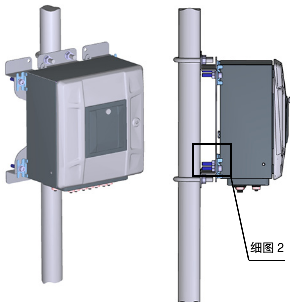
图 66 在安装板上安装接口单元 2 区接口单元
