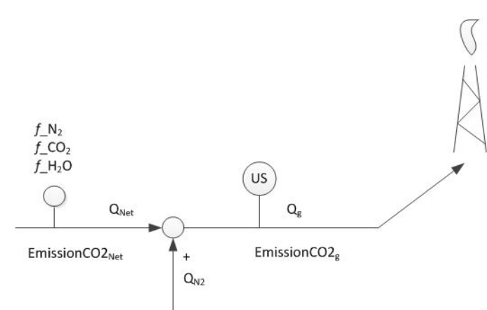
图 113 氮气补偿原理
