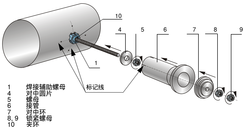
安装接管
