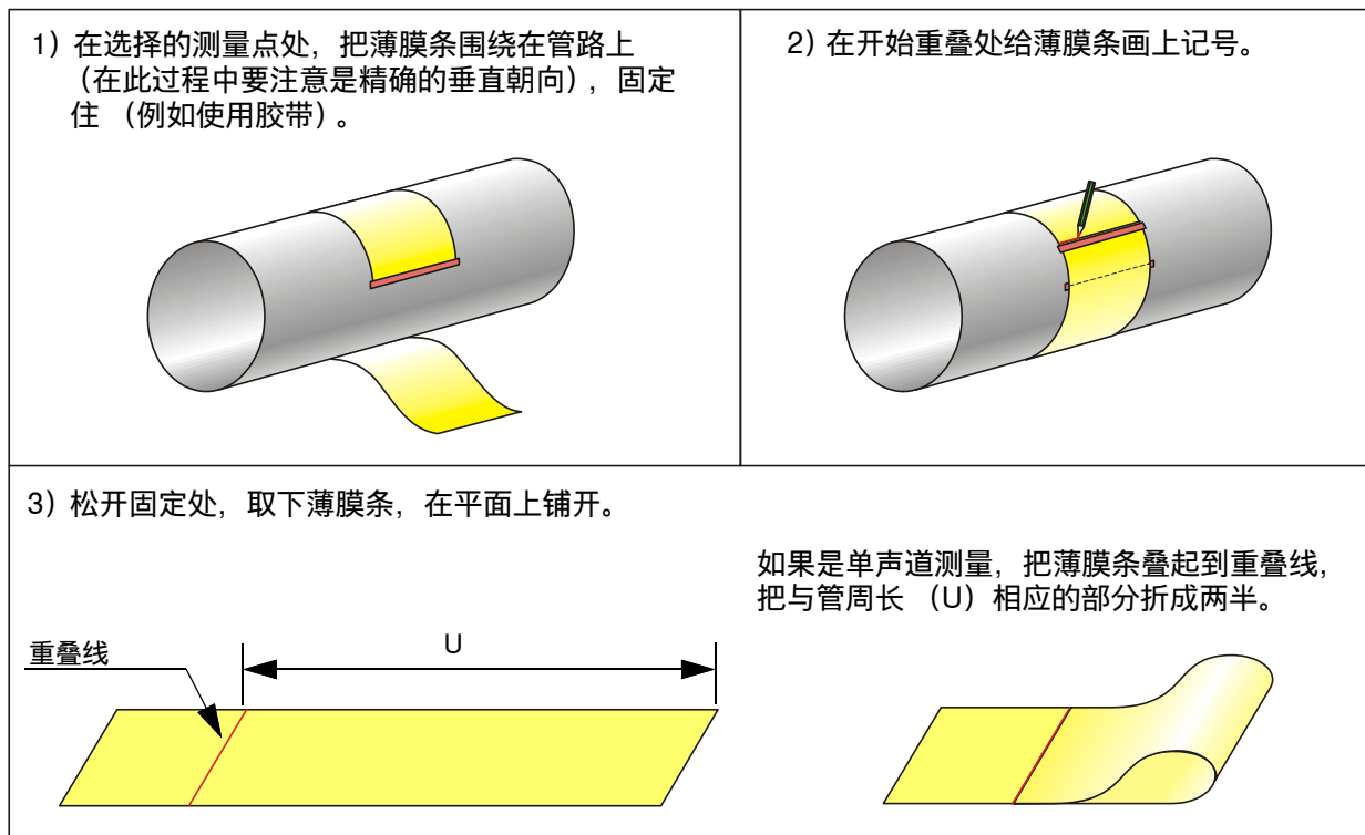
图 23 一般性准备工作
