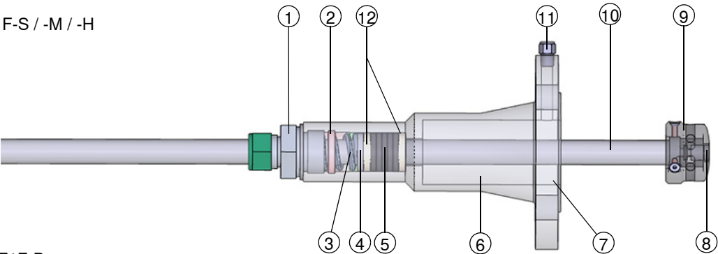
图 15 接触过程气部件
