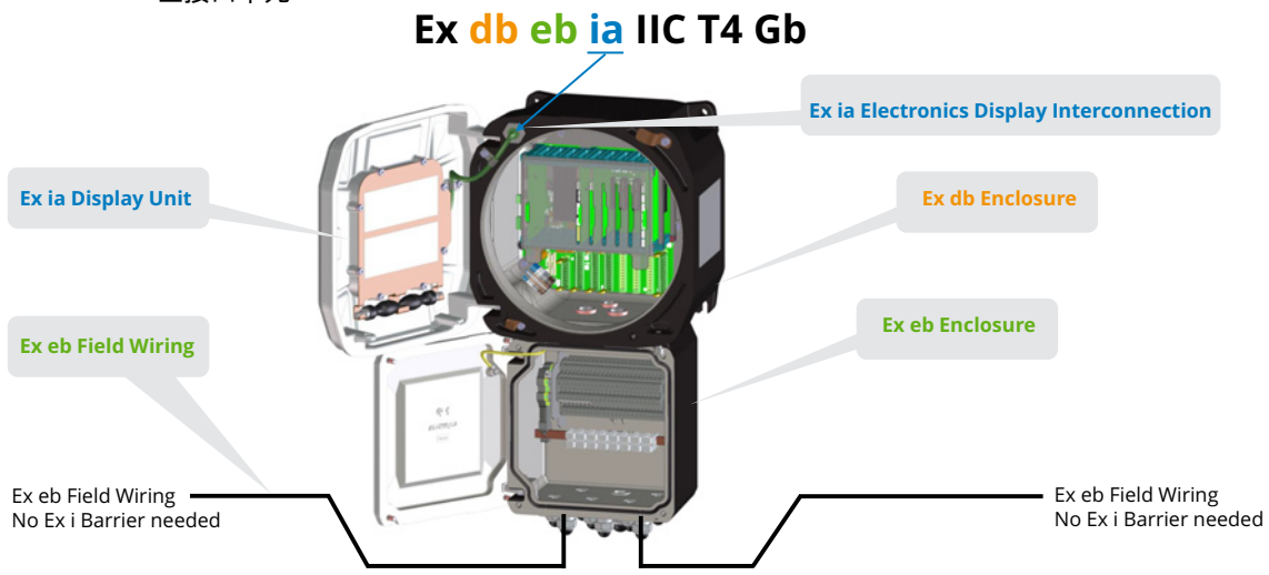
图 156 1 区接口单元 Ex d e
