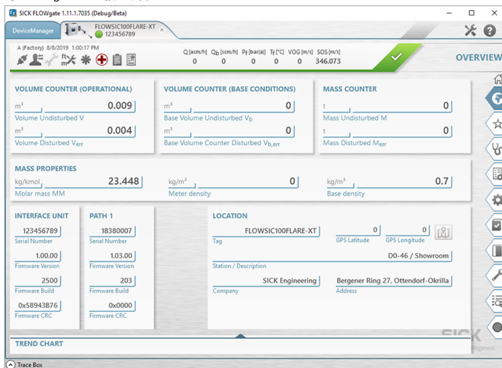
图 98 与 FLOWgate™ 连接 - 总览
