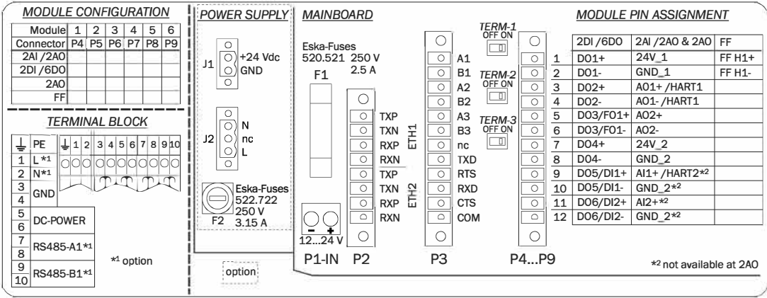
图 83 端子布置
