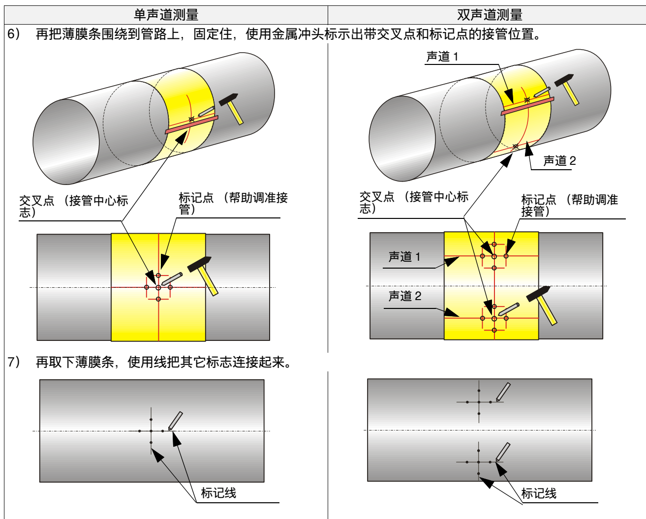
图 28 在管路上标示出测量探头结构的接管位置
