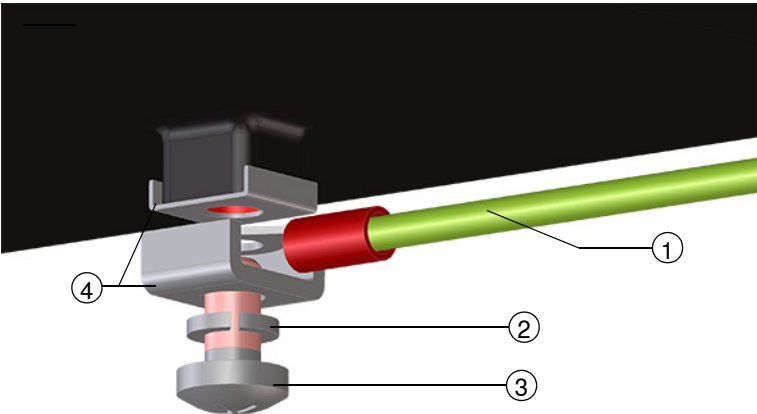
图 82 保护地线接头
