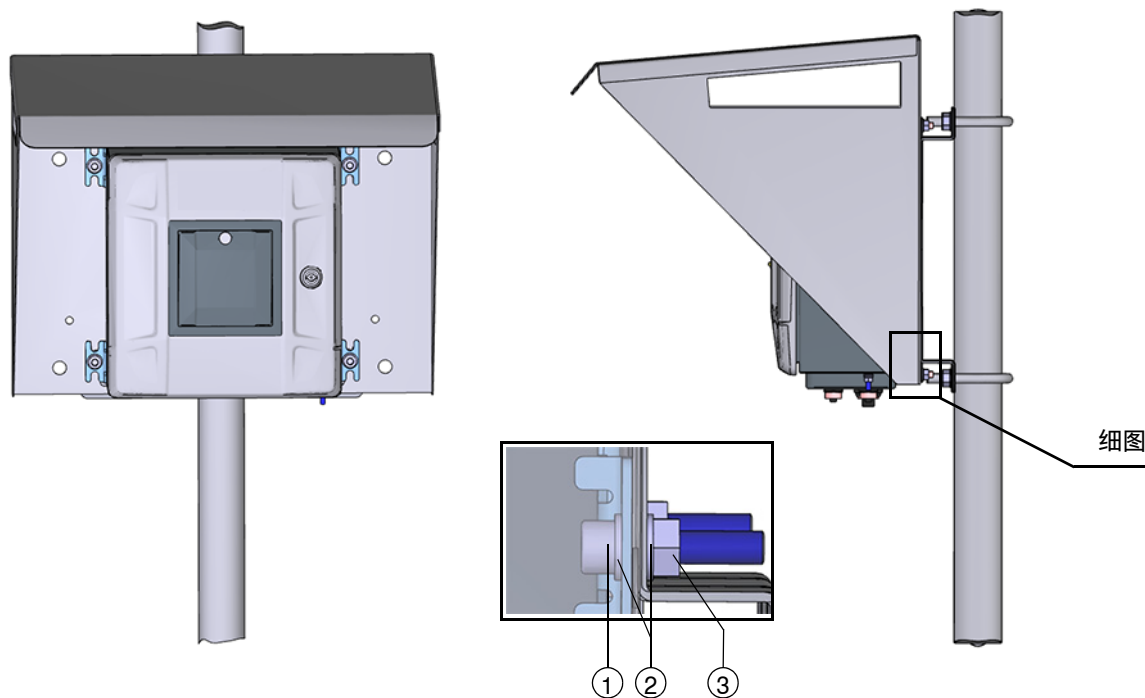
图 72 2 区接口单元与防晒（雨）罩安装在一起
