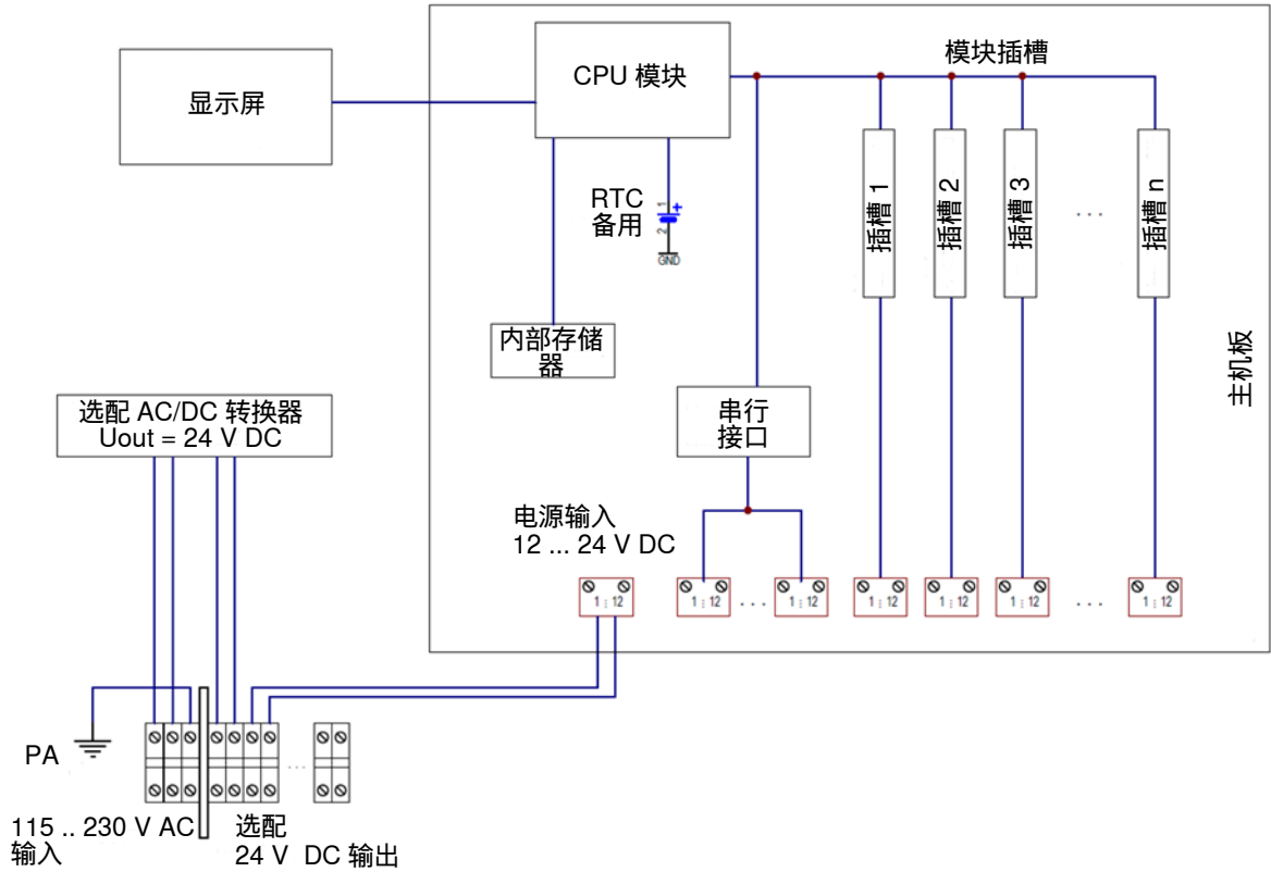
图 63 结构
