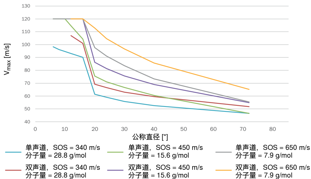
图 130 单声道和双声道对穿型仪器的 V_{\max} 随声速 (SOS) 变化示意图
