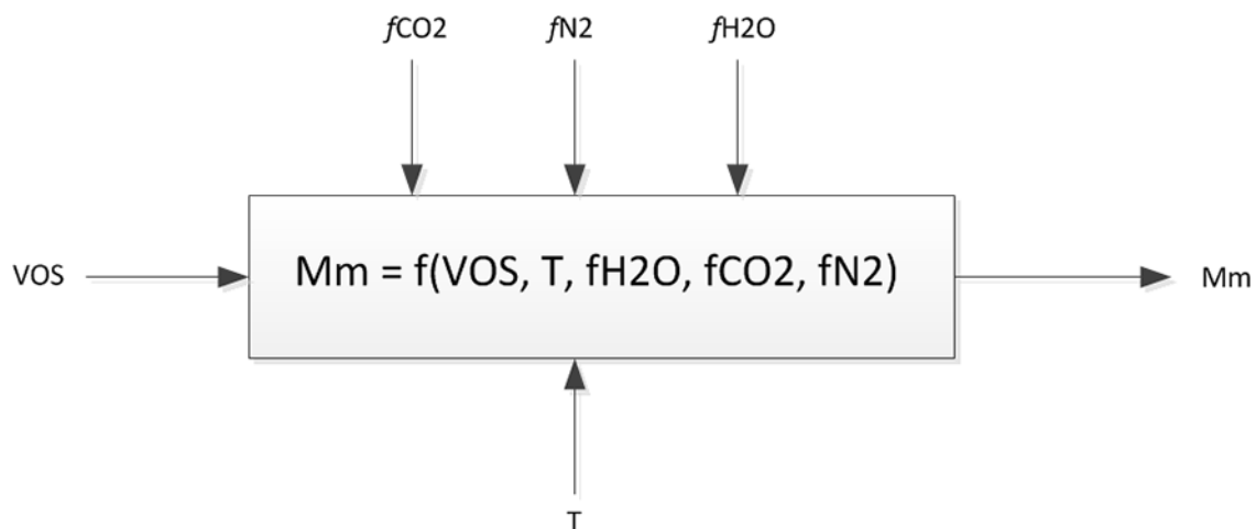
图 111 碳数算法的公式
