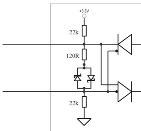
图 93 终端电阻
