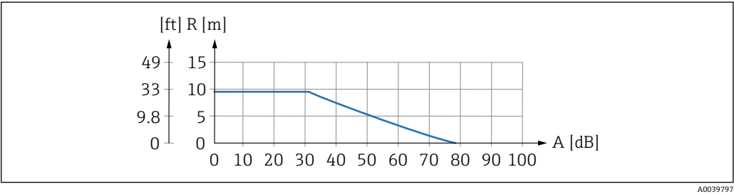
图 2 超声波物位传感器的测量范围曲线图
