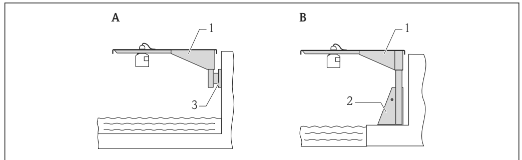
14 使用悬臂安装传感器
