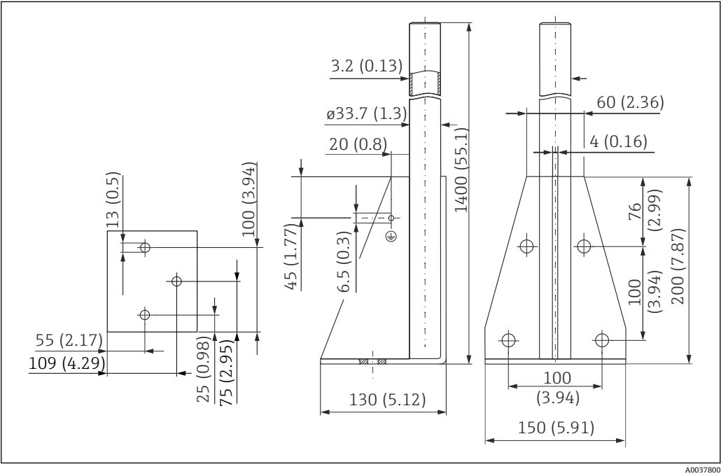
18 外形尺寸示意图。测量单位 mm (in)
