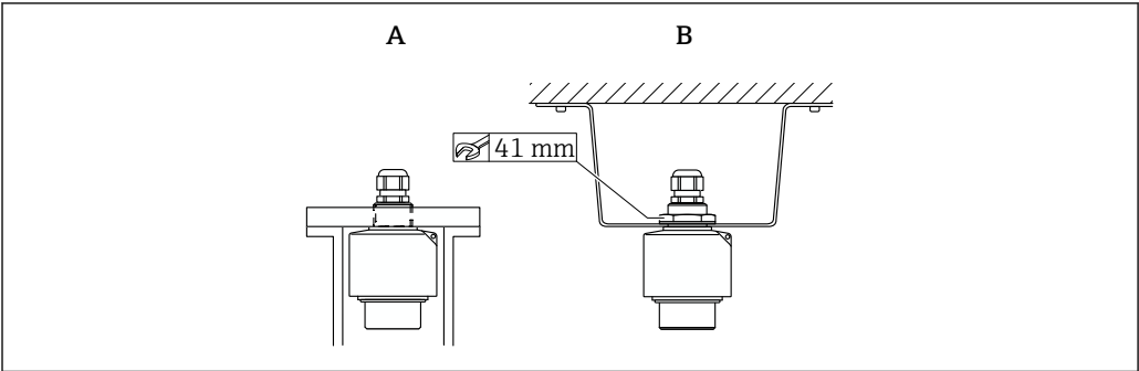
8 固定超声波物位传感器
