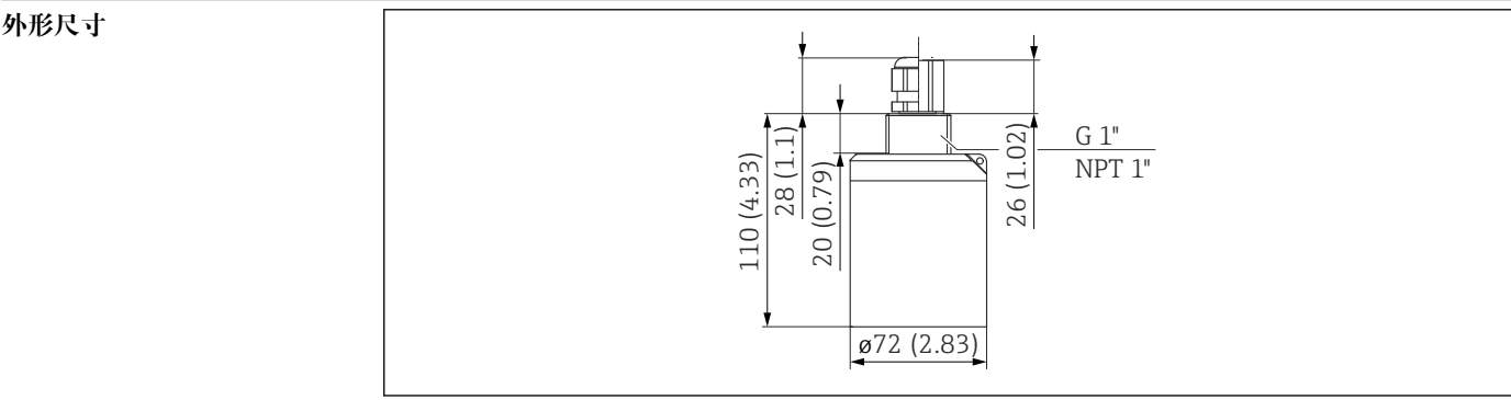
9 外形尺寸。测量单位 mm (in)
