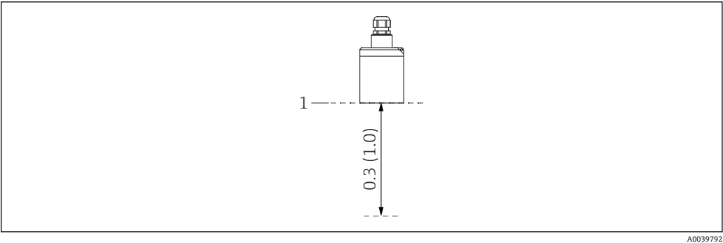
图 1 超声波物位传感器的盲区距离；单位：m (ft)
