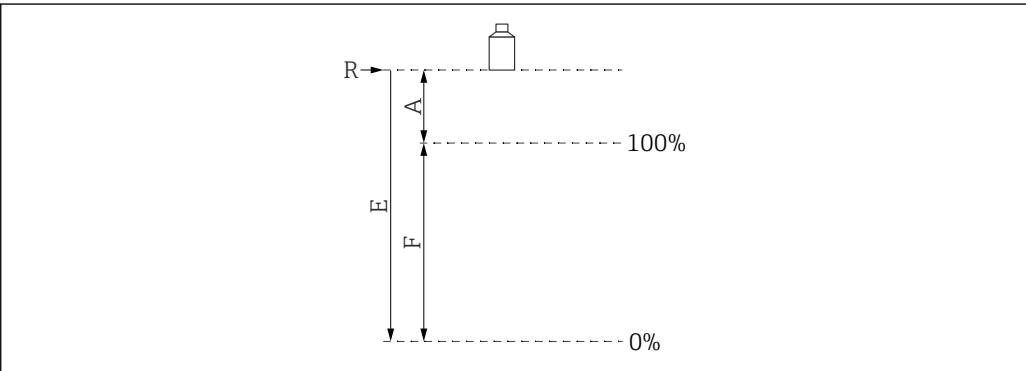
图 12 定义量程所需的变量
