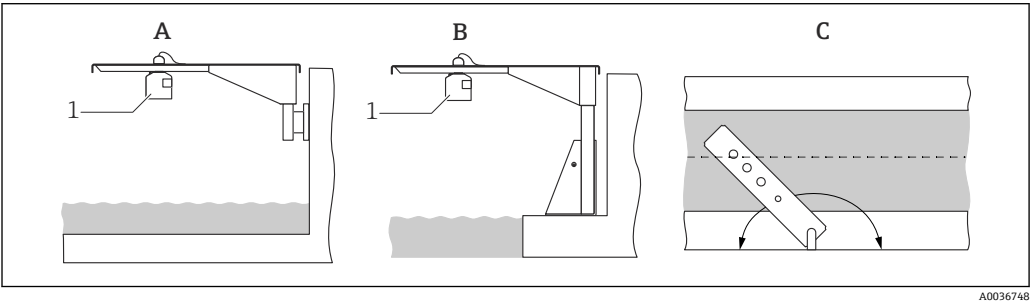
图 7 使用悬臂安装在明渠或水槽上方
