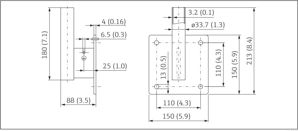
19 墙装架的外形尺寸示意图。测量单位 mm (in)
