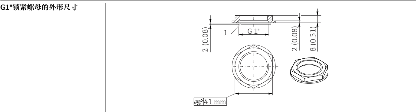
10 锁紧螺母的外形尺寸。测量单位 mm (in)
