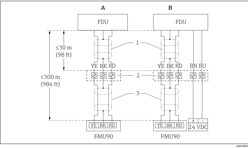
图 3 传感器接线图; YE = 黄色, BK = 黑色, RD = 红色, BU = 蓝色, BN = 棕色, 保护性接地线 (GNYE) = 绿/黄双色
