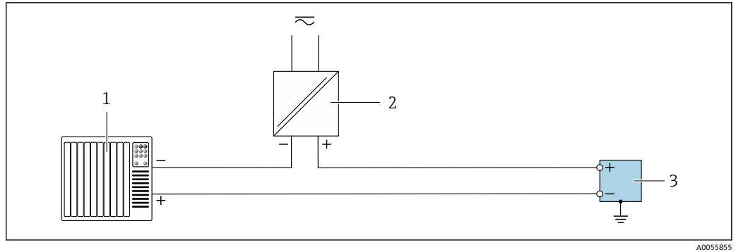
图 22 接线实例：脉冲输出/频率输出/开关量输出（无源）
