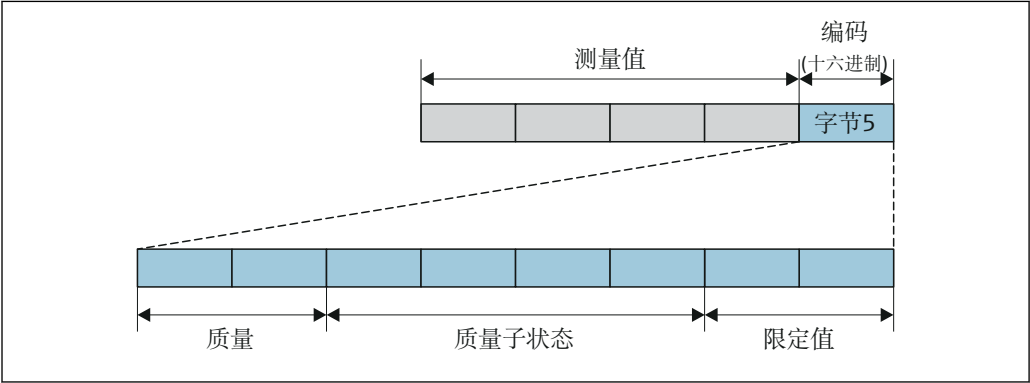
图 39 编码字节结构
