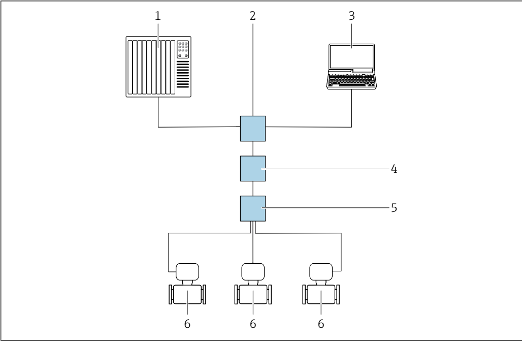
图 23 通过 Modbus TCP + Ethernet-APL 通信进行远程操作（有源信号）
