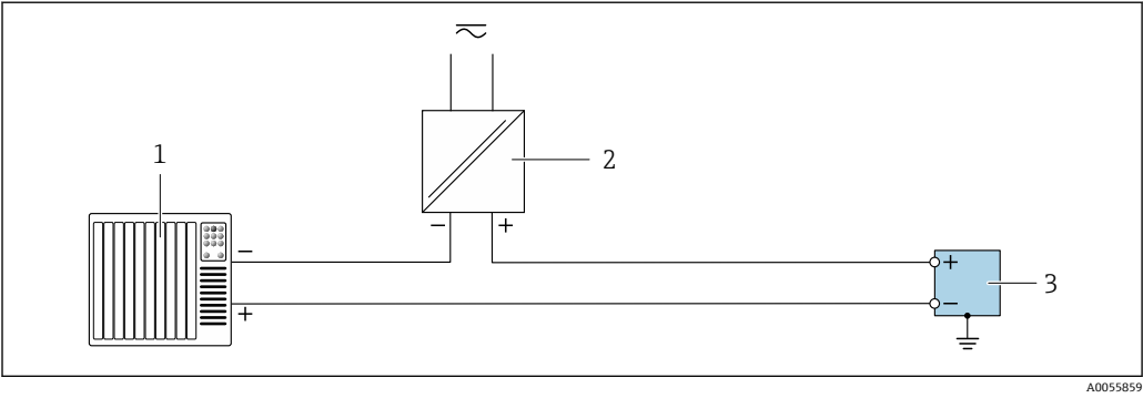
23 接线实例：继电器输出 1 自动化系统，带开关量输入（例如 PLC） 2 电源 3 变送器，带继电器输出
