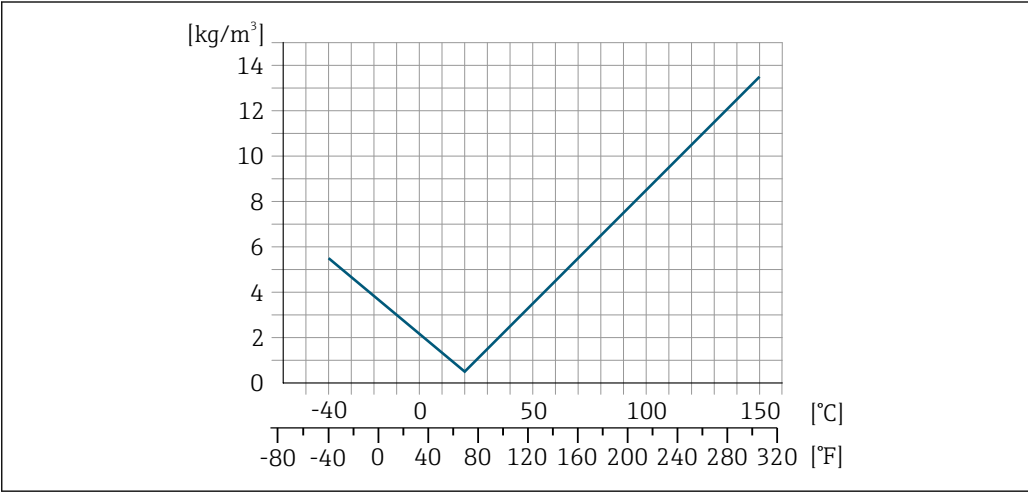
41 现场密度校正，例如在+20 °C (+68 °F)时
