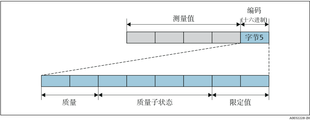
图 38 编码字节结构
