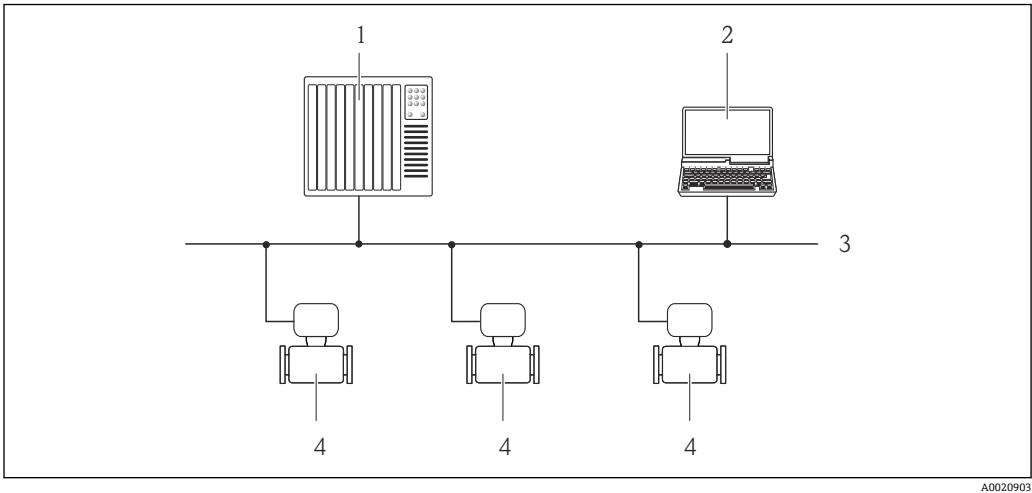
图 30 通过 PROFIBUS DP 网络进行远程操作
