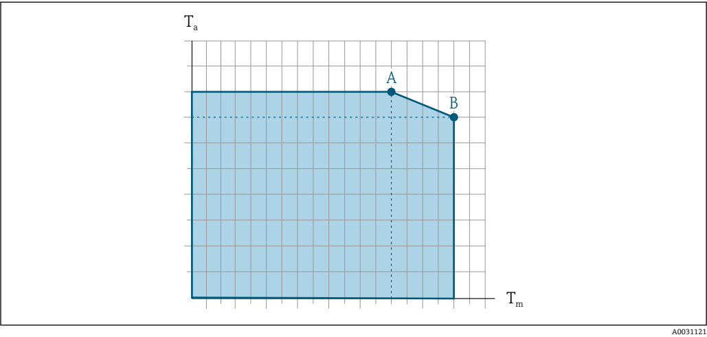
环境温度和介质温度的相互关系
