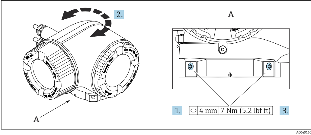
图 16 防爆型外壳
