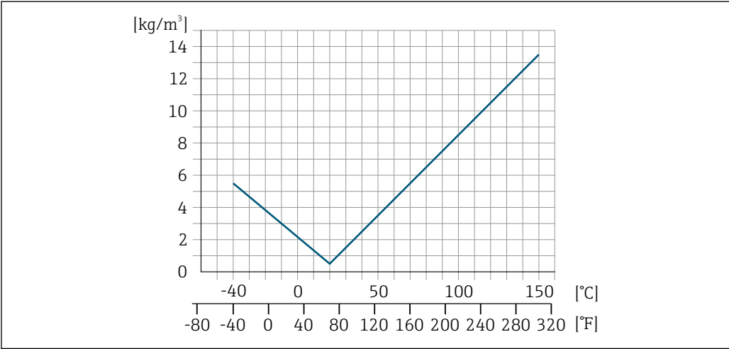
图 42 现场密度校正，例如在+20 °C (+68 °F)时
