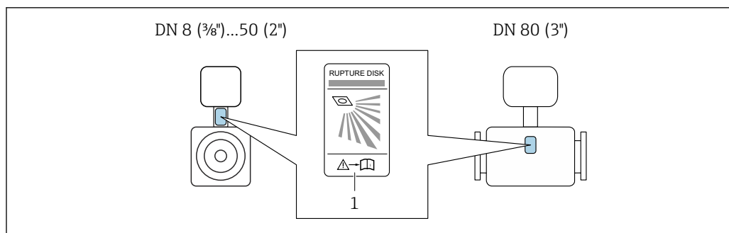
1 爆破片标签
