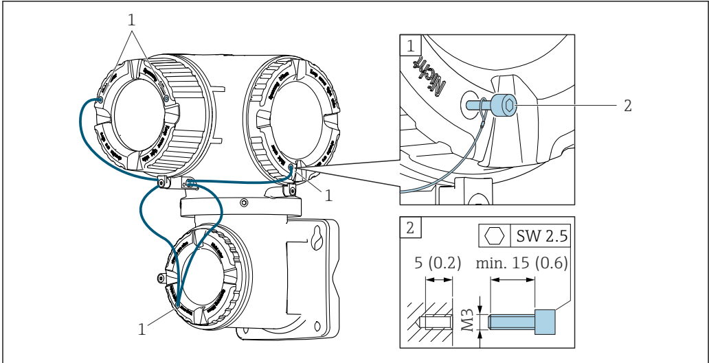
1 盖板上的开孔，用于安装固定螺丝 2 固定螺丝，用于锁定盖板
