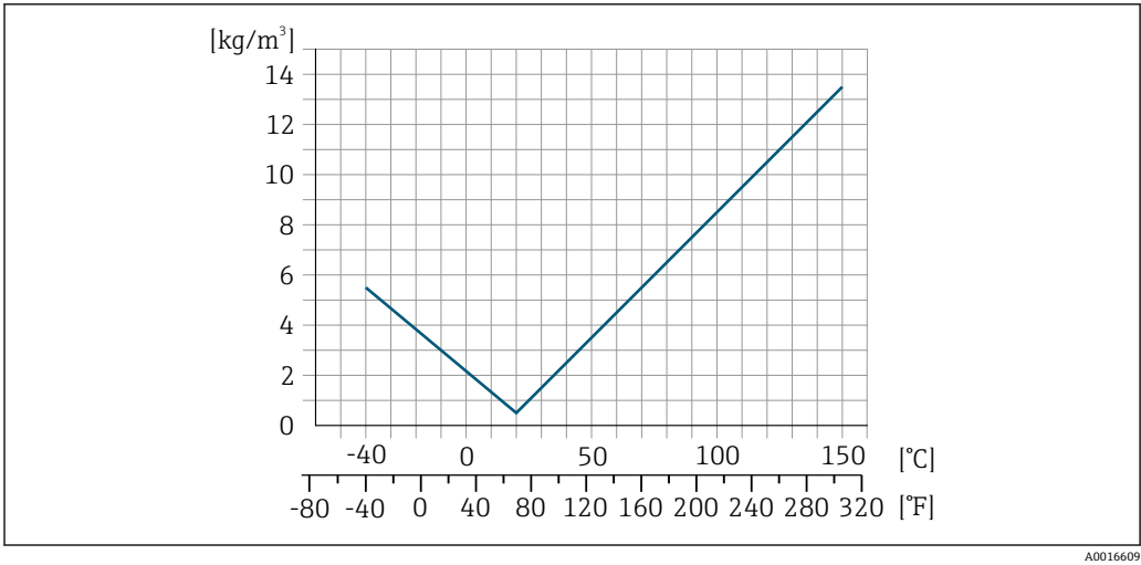
43 现场密度校正，例如在+20 °C (+68 °F)时
