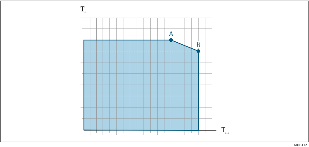
图 38 示例图，具体数值见下表。 T a 环境温度 T m 介质温度 A 介质温度 T m 越高 (T a max = 60 °C (140 °F) 时)，所需的环境温度 T a 越低 B 传感器最高允许介质温度 T m 对应的最高允许环境温度 T a
