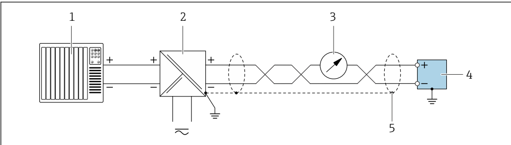
图 20 接线实例：4 ... 20 mA HART 电流输出（无源）
