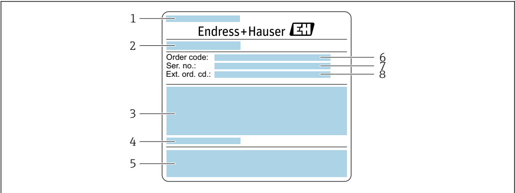
图 3 传感器的铭牌示意图（第 1 部分）
