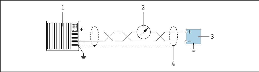
图 19 接线实例：4 ... 20 mA HART 电流输出（有源）
