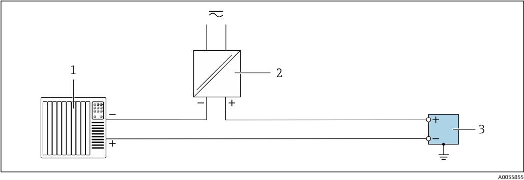
16 接线实例：脉冲输出/频率输出/开关量输出（无源）
