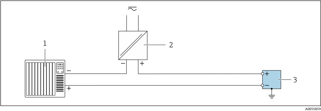
17 接线实例：继电器输出
