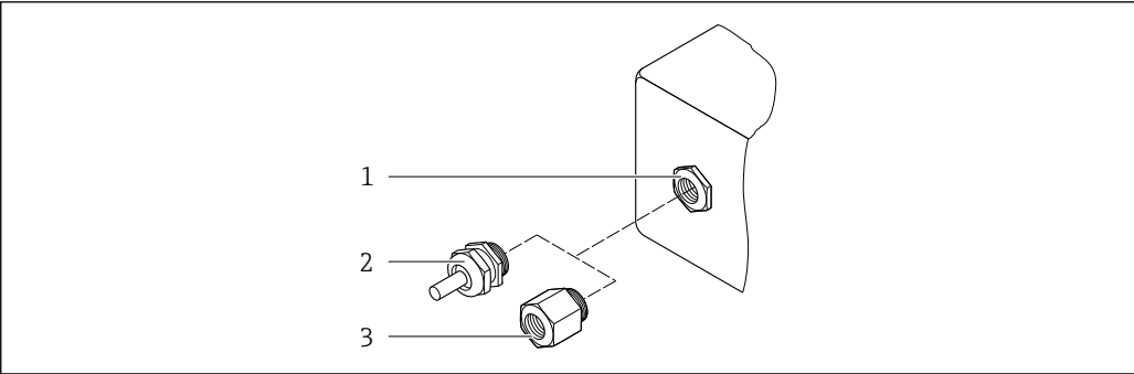
图 39 允许的电缆入口/缆塞 1 M20 × 1.5 内螺纹 2 M20 × 1.5 缆塞 3 转接头，适用 G ½"或 NPT ½"内螺纹电缆入口
