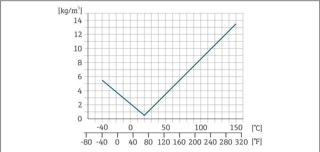
图 37 现场密度校正，例如在+20 °C (+68 °F)时
