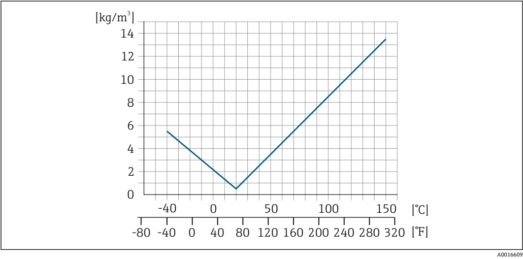
图 35 现场密度校正，例如在+20 °C (+68 °F)时
