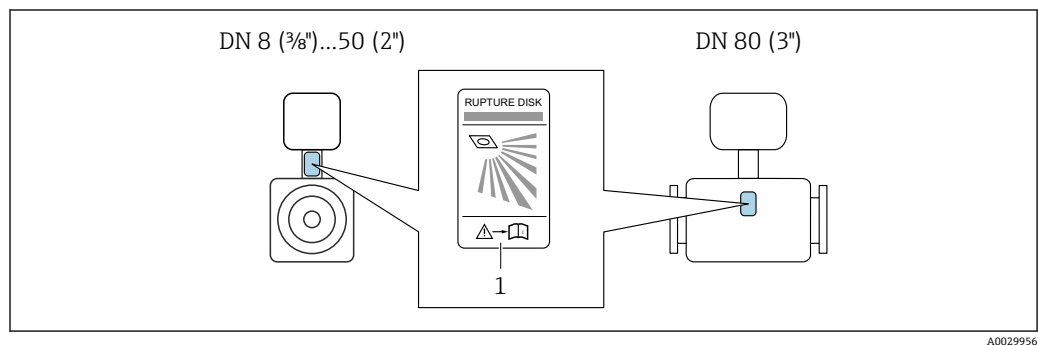
1 爆破片标签
