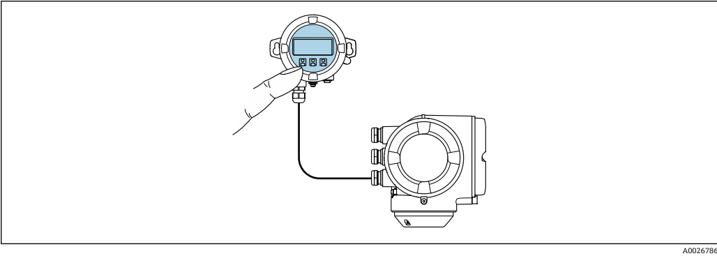
38 通过远传显示单元 DKX001 操作
